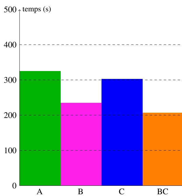
Figure 5.5 – Temps de résolution total pour |T| = 66 , \bar{d} = 30 et g = 1 selon différentes stratégies d'insertion de colonnes.
