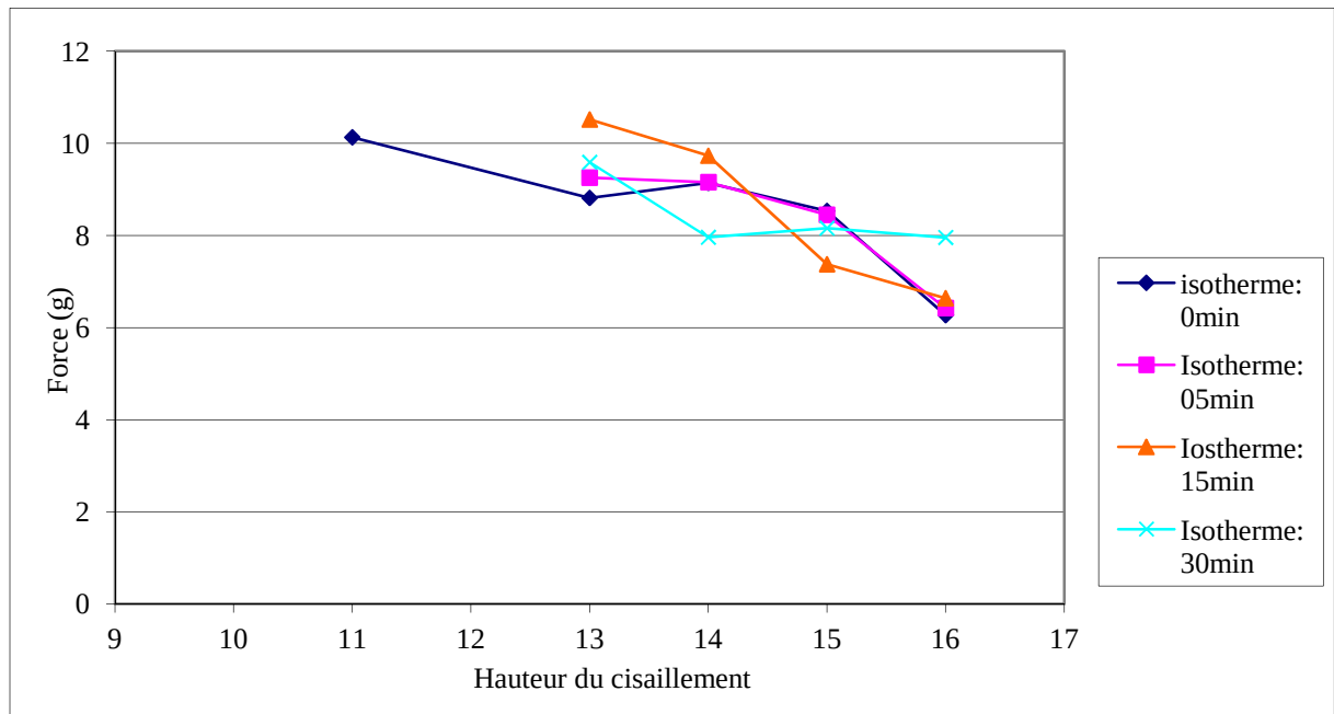
Figure A9-1: Evolution de la force maximale de cisaillement en fonction de la hauteur de cisaillement pour des micro-bumps comprenant une couche de nickel ayant subi des maintiens isothermes à 240^\circ\text{C} de différentes durées de maintien (voir figure 3-19 pour les profils thermiques). Vitesse de cisaillement: v = 70 \mu\text{m.s}^{-1} .
