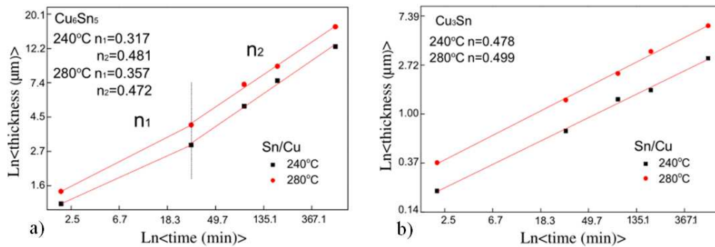
Figure 1-40: Cinétique de croissance des couches \eta - Cu_6Sn_5 (a) et \varepsilon - Cu_3Sn (b) à 240^\circ C et 280^\circ C [77].
