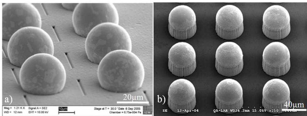
Figure 1-6 : Inspections MEB montrant un exemple de chacune des deux structures de connexion entre puces : le solder ball (a) et le micro-bump (b) [3].
