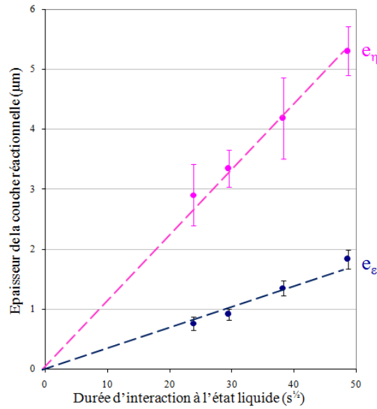
Figure 3-29: Variation de l'épaisseur totale moyenne des intermétalliques \eta -Cu 6 Sn 5 et \varepsilon -Cu 3 Sn en fonction de la racine carrée du temps de maintien à une température supérieure à la température de fusion (217,5°C) au cours des maintiens isothermes à 240°C (0min, 5min, 15min et 30min). Profil thermique en figure 3-19.
