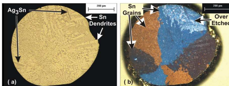
Figure 1-18: Observation de la microstructure de solidification d'un alliage SAC (Sn-3.9%Ag-0.6%Cu) refroidit à une vitesse de 1°C/sec à partir de 250°C. L'échantillon a connu une surfusion de 34°C au delà de la température eutectique. Observation optique (a), en lumière polarisée (b) [38].
