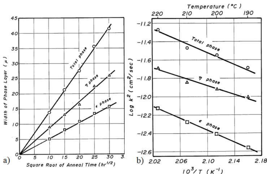
Figure 1-31: Variation de l'épaisseur des couches réactionnelles \eta\text{-Cu}_6\text{Sn}_5 et \varepsilon\text{-Cu}_3\text{Sn} en fonction de la racine carrée de la durée réactionnelle entre le cuivre et l'étain pour une température de 220°C (a), variation de la constante cinétique de croissance k avec la température [66].
