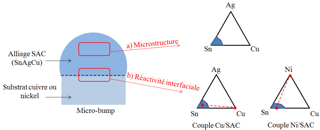
Figure 3-2: Représentations schématisques des systèmes ternaires concernés par les axes d'études: microstructure (a), réactivité interfaciale (b).
