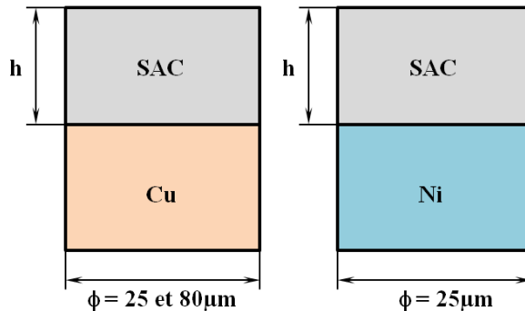
Figure 3-1: Présentation schématique des systèmes d'études: micro-bump ( \phi = 25\mu m ) et bump face arrière ( \phi = 80\mu m ) après le dépôt, sur substrat cuivre et sur substrat nickel.
