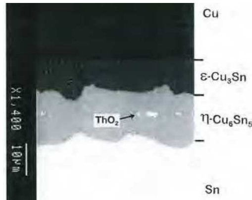
Figure 1-30: Cliché MEB de la zone interfaciale Cu/Sn après mise en contact de 225h à 215°C [65].
