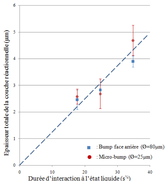
Figure 3-33: Variation de l'épaisseur totale moyenne de la couche réactionnelle ( e_{\text{totale}} = e_{\text{Cu}_6\text{Sn}_5} + e_{\text{Cu}_3\text{Sn}} ) en fonction de la racine carrée du temps de maintien à une température supérieure à la température de fusion (217,5°C) lors de maintiens isothermes à 230°C. Micro-bump ( \phi = 25\mu\text{m} ): • et bump ( \phi = 80\mu\text{m} ): ■.
