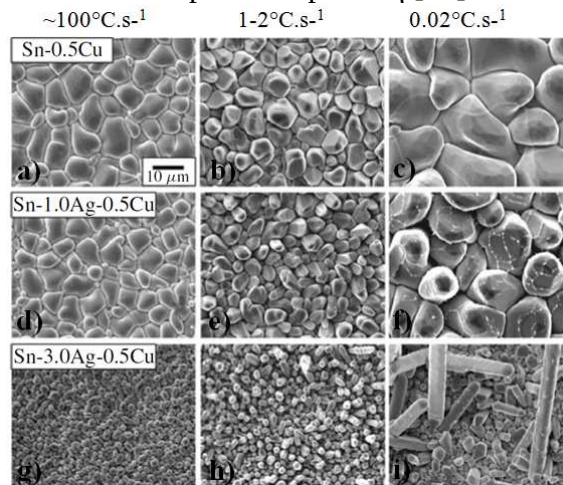
Figure 1-41 : Images MEB de la couche \eta apr  s un recuit de 5 min    250  C puis gravure chimique de la brasure n'ayant pas r  agi. Teneurs en Ag: 0% (a, b, c); 1% (d, e, f); 3% (g, h, i). Vitesse de refroidissement: 100^{\circ}\text{C.s}^{-1} (a, d, g); 1\text{-}2^{\circ}\text{C.s}^{-1} (b, e, h) 0.02^{\circ}\text{C.s}^{-1} (c, f, i) [82].
