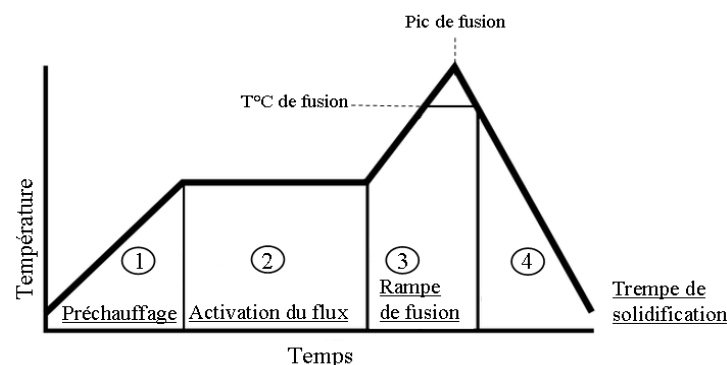
Figure 2-19: Représentation schématisée d'un profil de recuit thermique utilisé pour un procédé de bumping.
