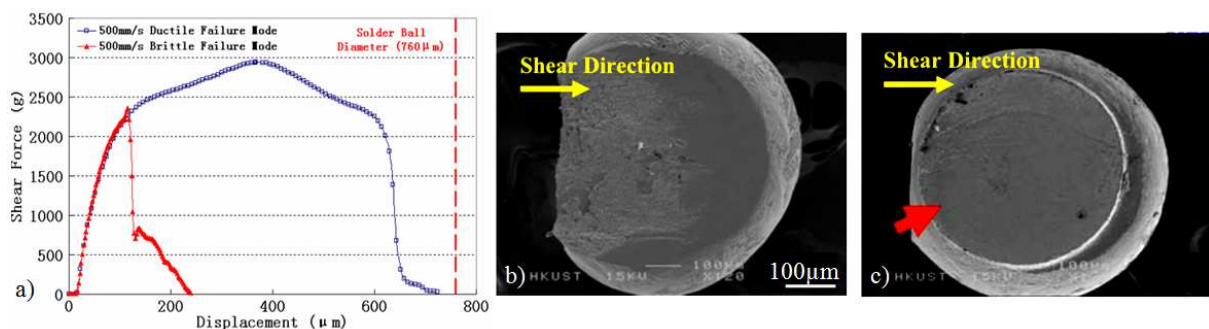
Figure 1-54 : Profil de force de cisaillement en fonction du déplacement effectué sur deux bumps type BGA (a). Rupture ductile (courbe bleue), micrographie du faciès de rupture ductile (b), rupture fragile (courbe rouge) micrographie du faciès de rupture fragile (c) [108].
