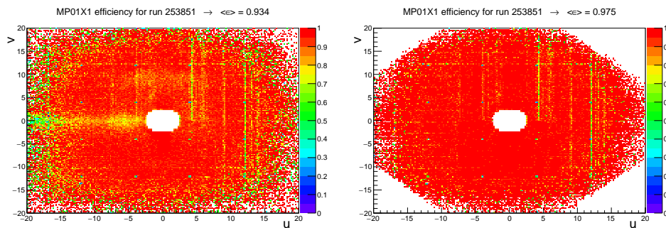
FIGURE 7 – Carte d'efficacité du détecteur MP01X1 avec (à droite) et sans (à gauche) sélection des traces détectées par les autres plans de Micromegas pixelisés
