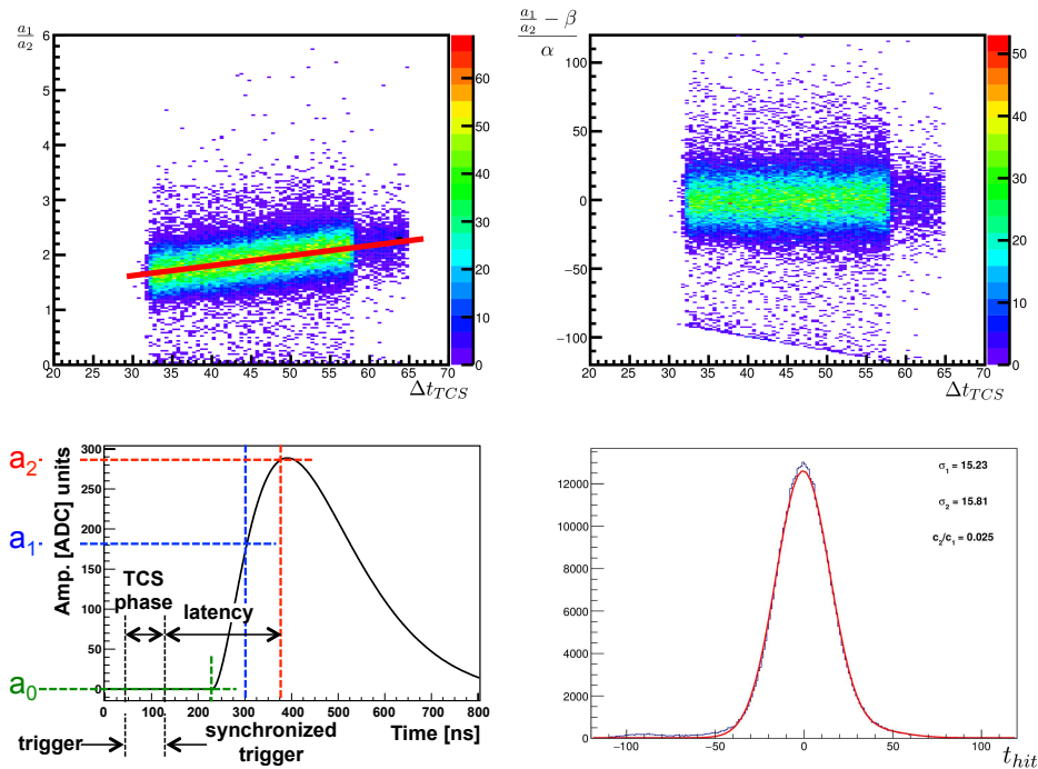
FIGURE 6 – Figures pour la calibration du timing des carte APV. En haut figures montrant le ratio a_1/a_2 avec et sans corrections. En bas à gauche schéma montrant le principe de mesure du temps du signal. En bas à droite distribution des temps des signaux corrigée
