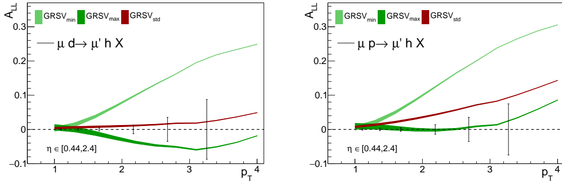
FIGURE 2 – Asymétries calculées en 2005 (1) pour le domaine cinématique de COMPASS
