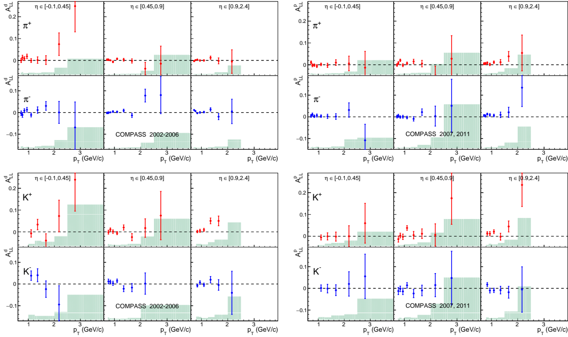
FIGURE 10 – Asymétries A_{LL}^d (à gauche) et A_{LL}^p (à droite) pour les pions identifiés (en haut) et les kaons identifiés (en bas)
