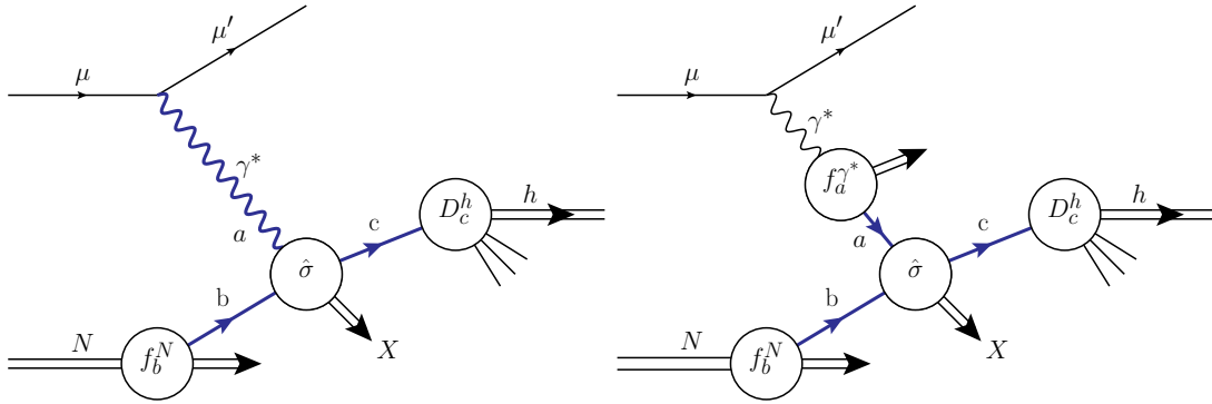
FIGURE 1 – Diagrammes de Feynman séparant les deux genres de contribution à la section-efficace en régime de photo-production : "directe" (à gauche) et "résolue" (à droite)
