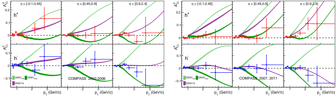
FIGURE 11 – Comparaison des asymétries A_{LL}^d et A_{LL}^p expérimentales avec les calculs théoriques pour deux jeux extrêmes de PDFs de GRSV et le jeu de PDFs le plus récent DSSV14
