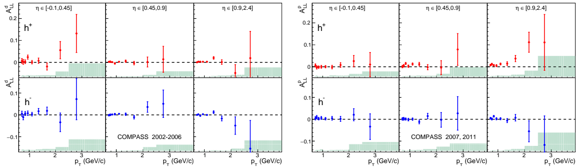
FIGURE 9 – Asymétries A_{LL}^d pour les données avec une cible de deutérium (à gauche) et A_{LL}^p pour les données avec une cible de proton (à droite) pour trois intervalles en \eta_{cms} [-0.1, 0.45, 0.9, 2.4] pour tous les hadrons positifs (en haut) et les hadrons négatifs (en bas)
