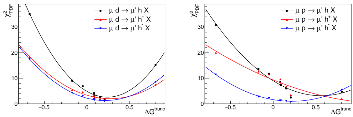
FIGURE 12 – Illustration de la minimisation du \chi^2 pour extraire \Delta G_{data}^{trunc} avec les calculs fait avec DSS14
