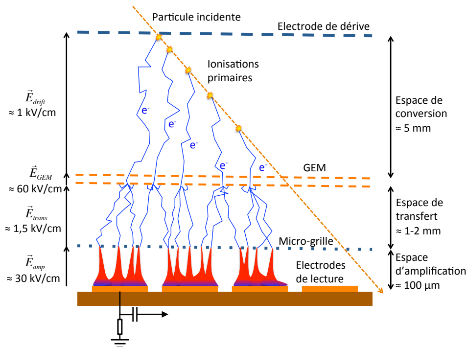
FIGURE 5 – Schéma de fonctionnement des Micromegas pixelisés
