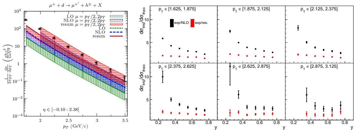
FIGURE 3 – Mesures des sections efficaces non polarisées pour des données de deutérium de COMPASS comparées aux calculs théoriques à différents ordres (LO, NLO et NLL) (à gauche). Ratios des sections efficaces expérience/théorie en fonction de y à NLO (en noir) et NLL (en rouge) (à droite)
