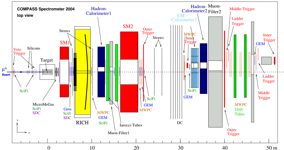
FIGURE 4 – Schéma en coupe du spectromètre de COMPASS
