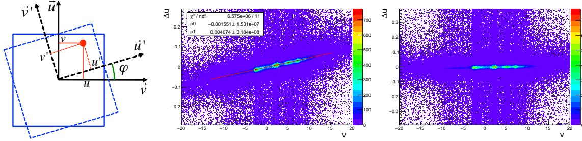
FIGURE 8 – Distribution des 2D des résidus avant (au centre) et après (à droite) correction de l'angle du détecteur. À gauche schéma montrant les changements de variable pour la rotation
