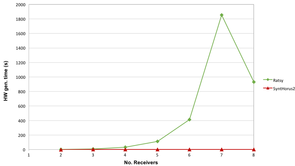
FIGURE 10.1 – Le temps de génération HW : GenBuf avec 2 émetteurs, plusieurs récepteurs et FIFO
