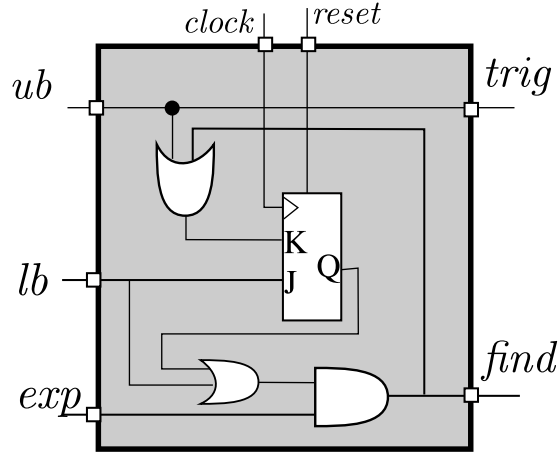
FIGURE 5.7 – La mise en oeuvre de \exists i \in [lb, ub]
