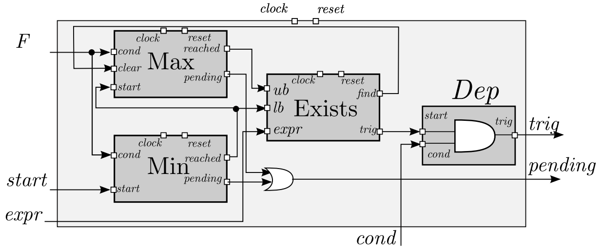
FIGURE 5.6 – La mise en oeuvre de l'expression de "exist"
