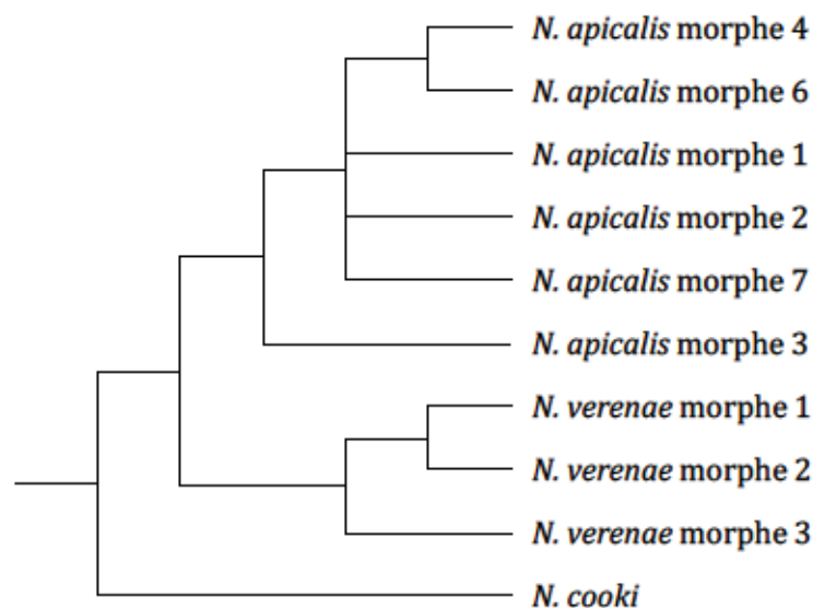
Figure 1. Arbre consensus des relations phylogénétiques bien soutenues au sein du complexe N. apicalis . La position de N. obscuricornis n'est pas connue.
