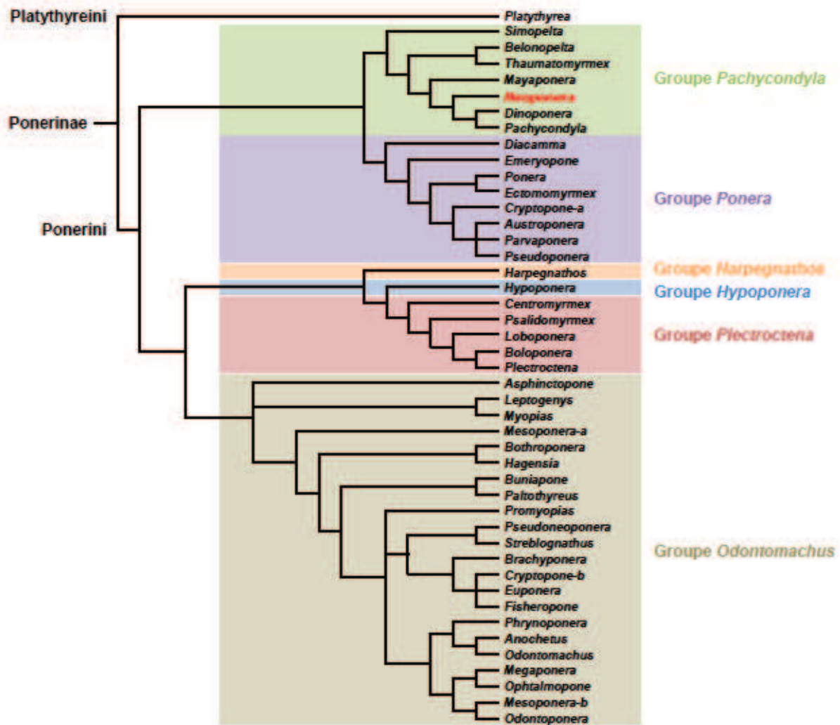
Figure 1. Relations entre les genres de Ponerinae. Cryptopone-a représente C. hartwigi , Cryptopone-b représente C. gilva et C. testacea , Mesoponera-a représente M. melanaria et Mesoponera-b représente M. ambigua . La position des taxons suivants n'est pas connue : Dolioponera , Feroponera , Iroponera et Rasopone . D'après Schmidt (2013) et Schmidt et Shattuck (2014), avec leur autorisation.
