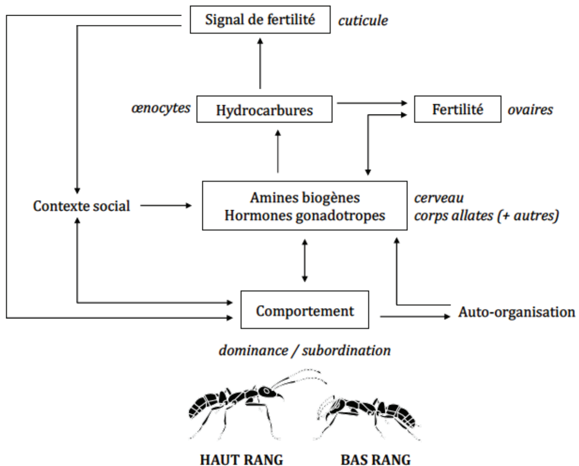
Figure 2. Mécanismes proximaux intervenant dans la détermination des rangs hiérarchiques et leurs influences mutuelles.
