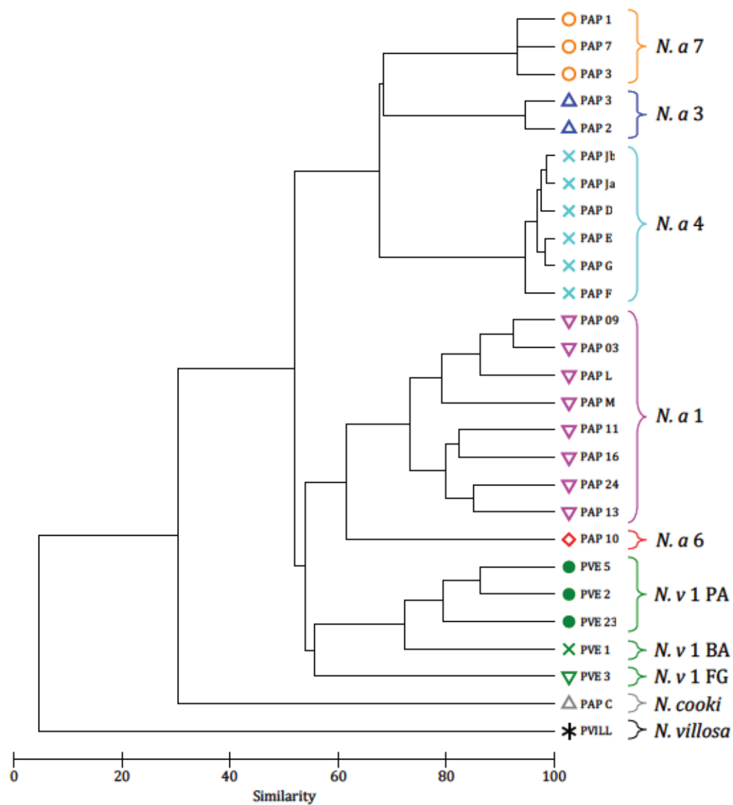
Figure 3. Chemical dendrogram of the mean CHC profiles of all colonies. N. a , N. apicalis ; N. v , N. verenae ; BA, Bahia; PA, Pará; FG, French Guiana.
