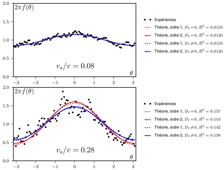
Figure 2.3 – Comparaison entre les distributions angulaires expérimentales et théoriques, sans paramètre d’ajustement, pour deux valeurs de v_s/v . R^2 , donné par l’équation (2.23), quantifie la qualité de l’accord entre expérience et théorie. D_r = 0.64 \text{ s}^{-1} , D_t = 0.274 \mu\text{m}^2 \cdot \text{s}^{-1} , v_s = 0.33 \mu\text{m} \cdot \text{s}^{-1} .
