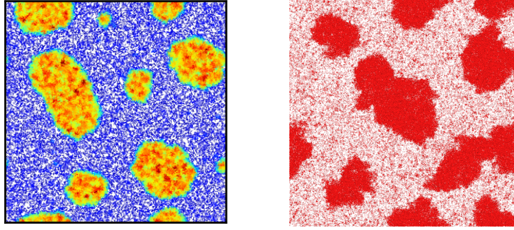
Figure 4.3 – Exemples de MIPS pendant la phase de coarsening. Gauche : Pour des RTP nageant à une vitesse v(\bar{\rho}) où \bar{\rho} est la densité moyenne au voisinage d’une particule. Reproduite de l’article C. Droite : Pour des sphères dures ABP. Reproduite de [59].
