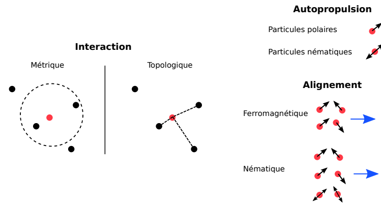
Figure 1.6 – Variations autour du modèle de Vicsek étudiées dans la littérature [68–71]. L’interaction peut être métrique ou topologique (ici avec les trois plus proches voisins). L’autopropulsion est polaire ou nématique et l’alignement ferromagnétique ou nématique.
