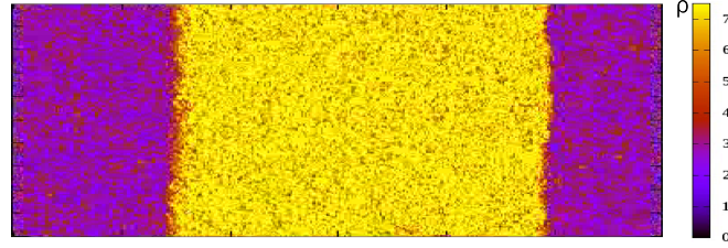
Figure 5.9 – Séparation de phase dans le modèle de Potts actif à quatre couleurs. Paramètres : \beta = 4.5 , \rho_0 = 5.5 , \varepsilon = 0.9 , D = 1 , taille du système 600 \times 200 .
