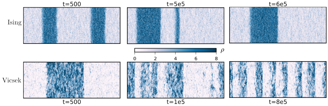
Figure 5.5 – Dynamique des bandes dans le modèle d'Ising actif (haut) et dans le modèle de Vicsek (bas). Haut : dans le modèle d'Ising actif, les échanges de masse entre bandes (centre) conduisent à des variations de vitesse, si bien que deux bandes fusionnent aux temps longs (droite). Paramètres : \beta = 1.8 , \rho_0 = 2.8 , D = 1 , \varepsilon = 1.9 , taille du système 800 \times 100 . Bas : dans le modèle de Vicsek, un domaine liquide est métastable (gauche). Il se fractionne en plusieurs bandes. Les bandes échangent de la masse pour égaliser leur taille et une interaction répulsive conduit à un arrangement périodique (droite). Paramètres : v = 0.5 , \eta = 0.4 (bruit angulaire), \rho_0 = 2.25 , taille du système 800 \times 100 .
