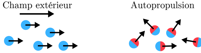
Figure 1.1 – Contrairement à l’application d’un champ extérieur (par exemple un champ électrique sur des particules chargées), les particules actives sont propulsées chacune par des forces internes.
