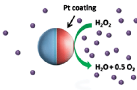
Figure 1.3 – Autopropulsion par diffusiophorèse de colloïdes Janus recouverts de platine sur la moitié de leur surface. La réaction chimique entre le platine et le peroxyde d’hydrogène \text{H}_2\text{O}_2 crée un gradient de concentration qui propulse la particule. Reproduite de [33].
