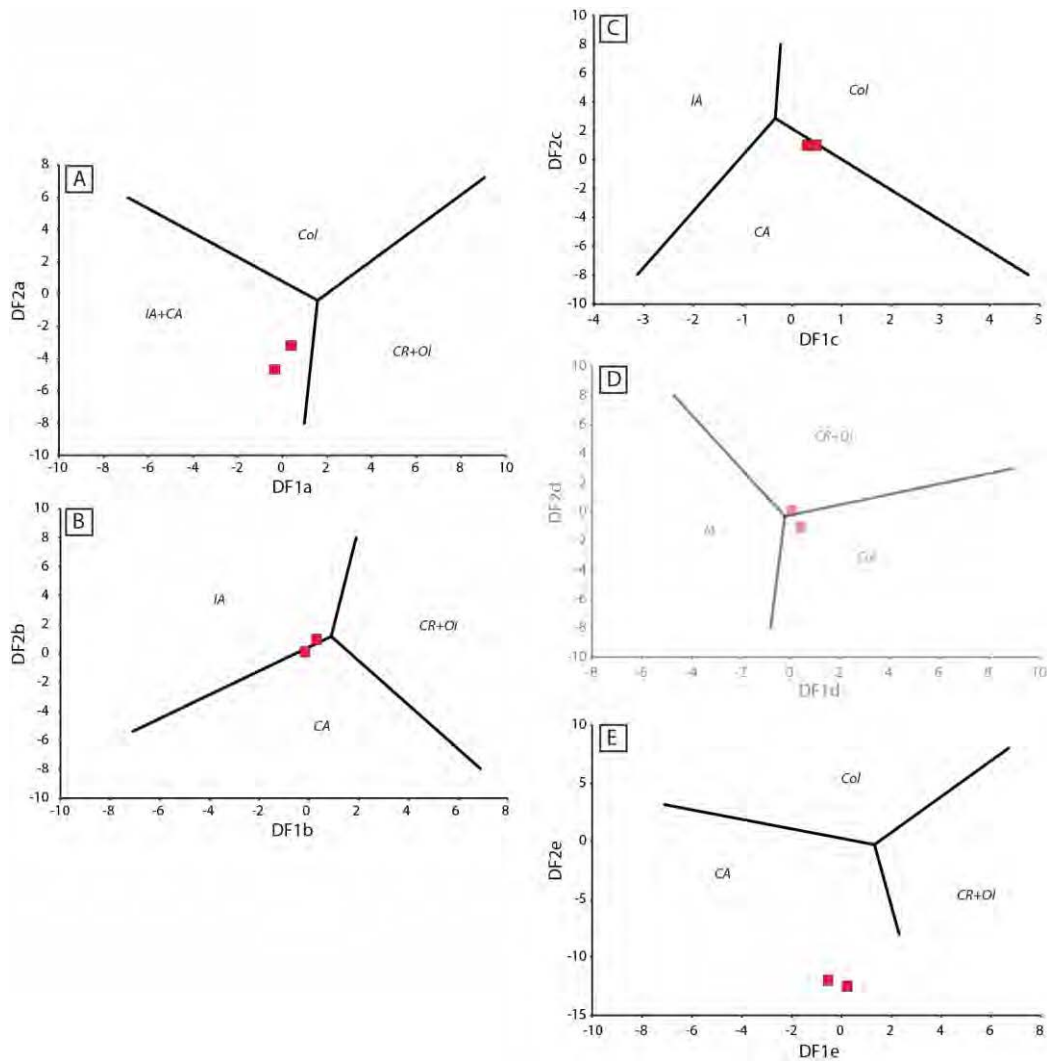
Figure 4.48. Diagrammes de discriminations des roches acides ( \text{SiO}_2(\text{adj}) > 63\% ), Verma et al., 2013. DF : Fonctions discriminantes. IA: Island Arc ; CA: Continental Arc ; CR: Continental Rift ; OI: Oceanic Island ; Col: Collision . Le diagramme D correspond au diagramme inapplicable (le champ CA n'est pas présent dans ce diagramme).
