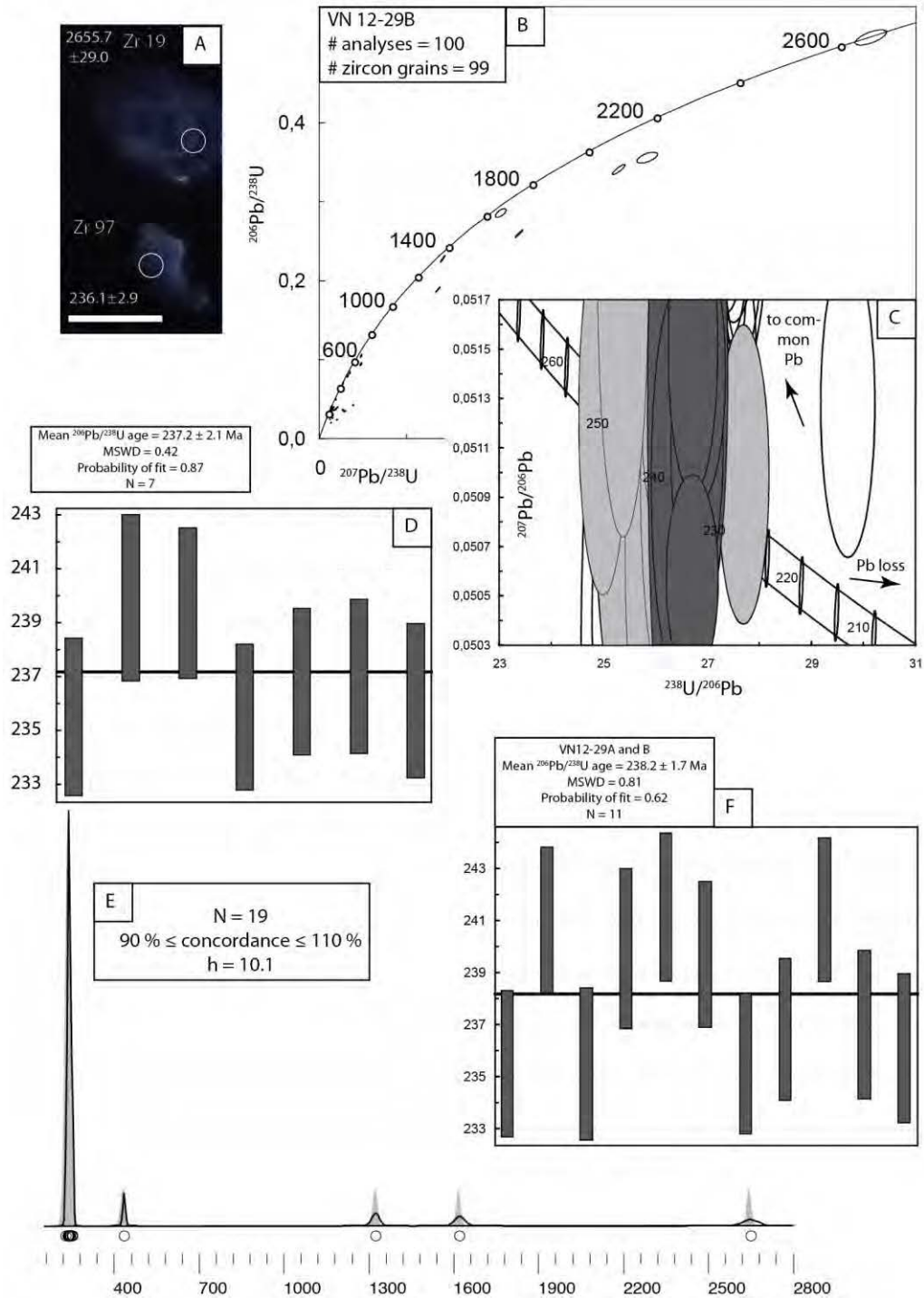
Figure 4.18. Analyses géochronologiques de l'échantillon VN 12-29B (échantillonnage classique). A. Image en cathodoluminescence de deux zircons appartenant à deux populations différentes. La barre d'échelle mesure 100 \mu\text{m} . Les cercles ( \varnothing = 25 \mu\text{m} ) indiquent les emplacements échantillonnés par ablation laser. Les incertitudes sont données à 1\sigma . B. Diagramme Concordia Wetherill. Les ellipses sont dessinées à 1\sigma . C. Diagramme Concordia Tera-Wasserburg focalisé sur les analyses les plus jeunes. Les ellipses sont dessinées à 1\sigma , les ellipses en gris clair correspondent aux analyses concordantes, les ellipses en gris foncé correspondent aux analyses utilisées pour calculer l'âge maximum de dépôt. D. Age maximum de dépôt pour le « sous échantillon » VN 12-29B, calculé comme l'âge moyen pondéré ^{206}\text{Pb}/^{238}\text{U} du cluster d'analyses le plus jeune. N : nombre d'analyses incluses dans le calcul. Les boîtes sont dessinées à 1\sigma .
