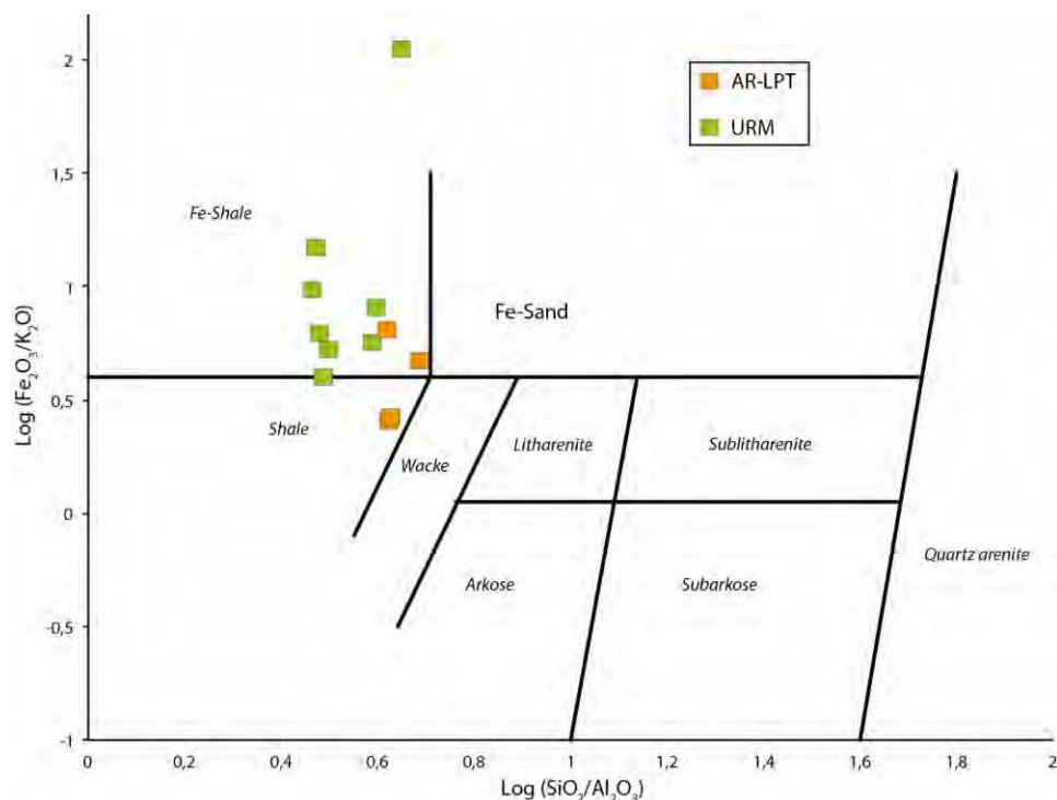
Figure 1. Classification chimique des roches volcano-sédimentaires du Bassin de Luang Prabang. Tous les échantillons se placent dans les champs des shales alors qu'il s'agit de grès lithiques ou feldspathiques (arkoses). L'emploi de cette classification chimique est donc déconseillé, au moins pour les roches volcano-sédimentaires. AR-LPT : Echantillons des Argiles Rouges et Tuffites de Luang Prabang, URM : échantillons de l'Unité des Roches Mafiques.
