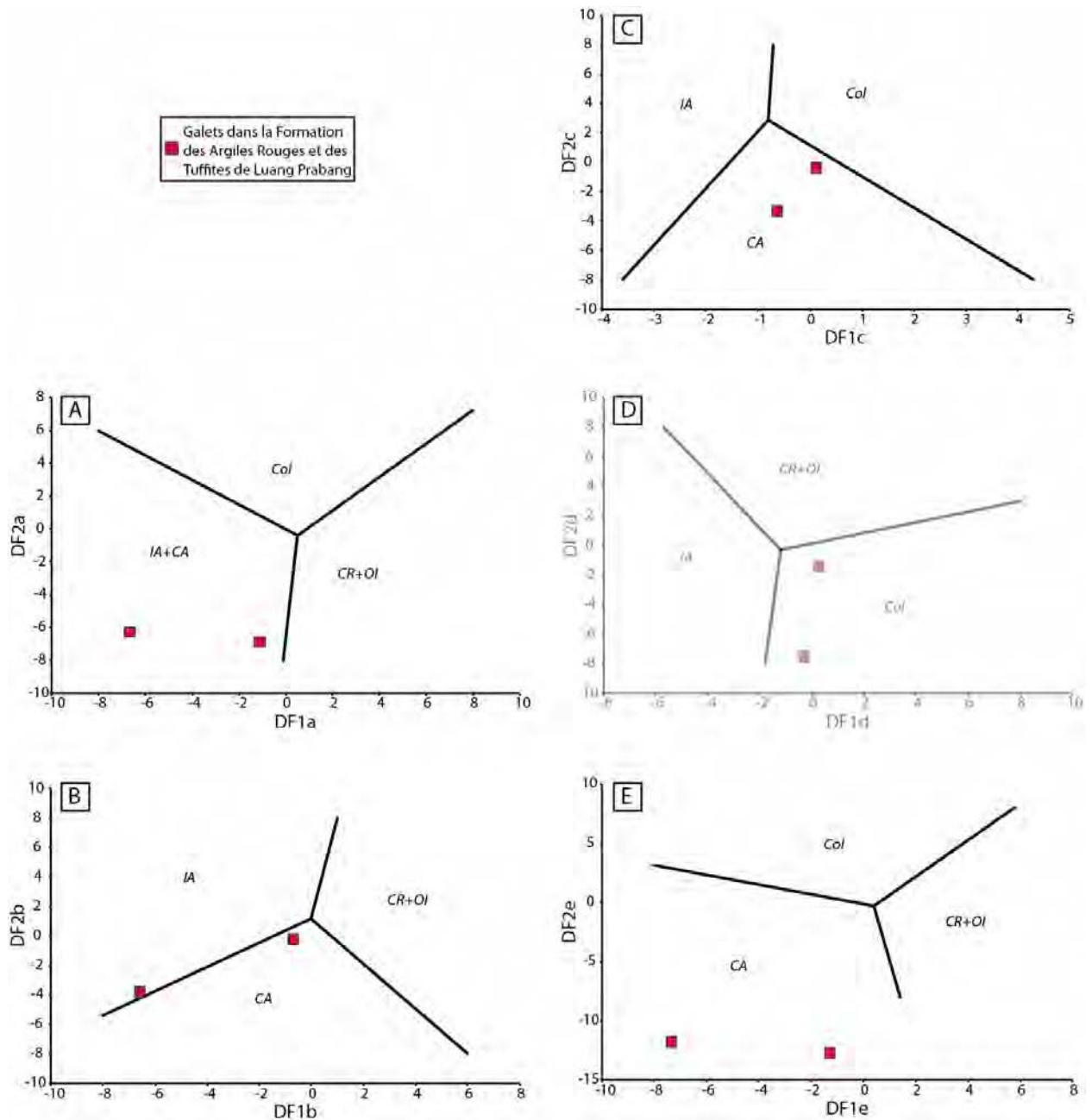
Figure 3.39. Diagrammes de discrimination des roches acides ( \text{SiO}_{2(\text{adj})} > 63\% ), Verma et al., 2013. DF : Fonctions discriminantes. IA: Island Arc ; CA: Continental Arc ; CR: Continental Rift ; OI: Oceanic Island ; Col: Collision . Le diagramme D correspond au diagramme inapplicable (le champ CA n'est pas présent dans ce diagramme).
