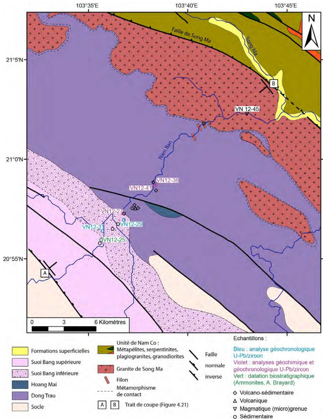
Figure 4.4. Carte du Bassin de Sam Nua (révisée d'après Son et al., 2005 et cette étude). Les échantillons VN 12-27, 29, 31, 38 et 41 ont été étudiés dans le cadre de ce travail. Les échantillons VN 12-25 et VN 12-45 ont été prélevés au cours de la même mission de terrain puis ont été analysés, respectivement par A. Brayard (Biogéosciences Dijon) et F. Roger (Géosciences Montpellier).
