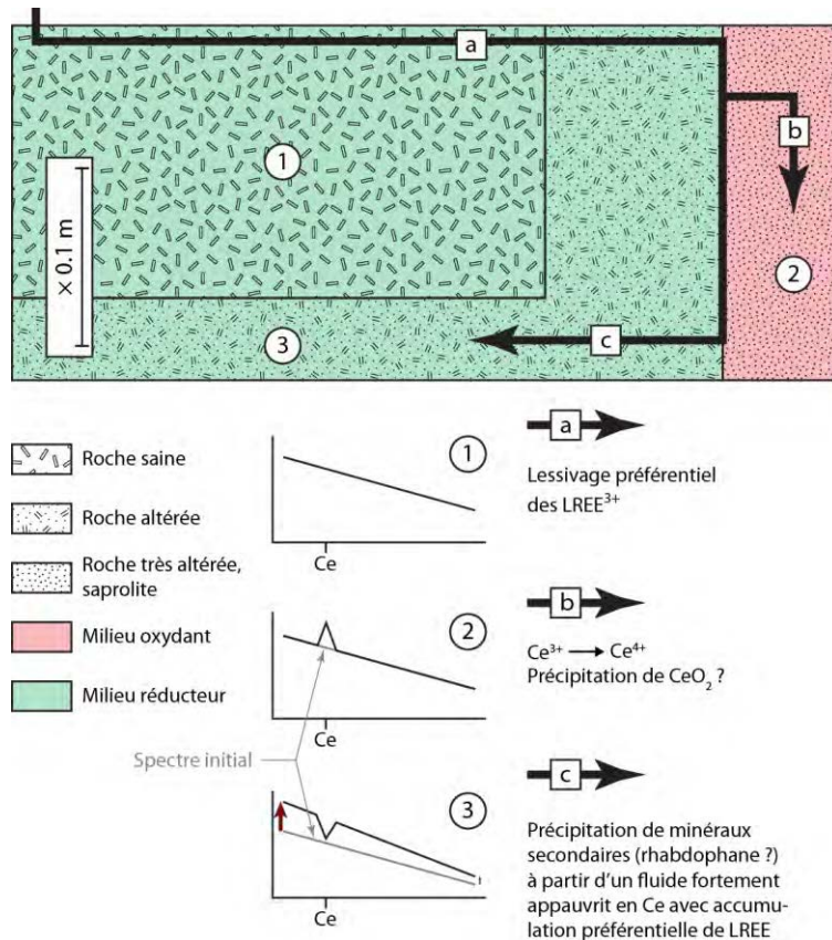
Figure 4. Rôle de la mobilité différentielle des REE sur l'allure du spectre. Les numéros correspondent aux emplacements des échantillons analysés. L'échelle proposée (quelques décimètres) correspond à la distance séparant des échantillons de roche fraîche d'échantillons dans lesquels sont observés des accumulations en REE dans les travaux de Marsh (1991) et Förtser (2000).
