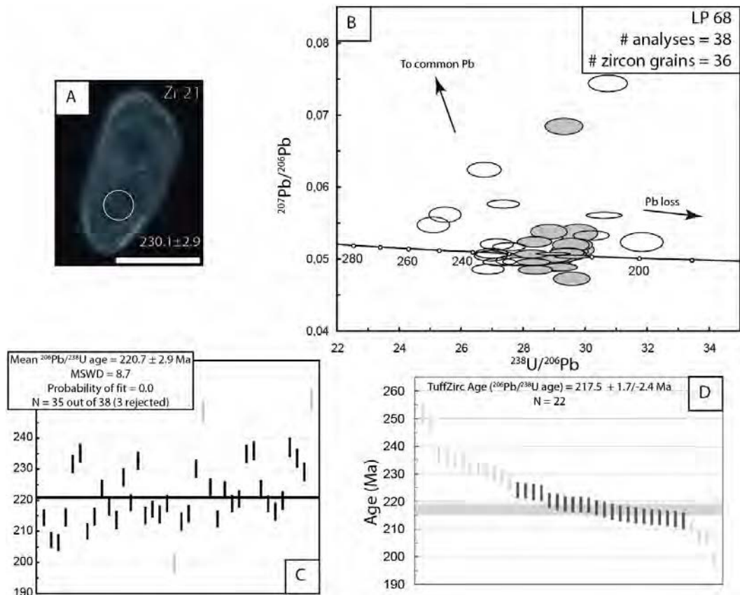
Figure 3.13. Analyses géochronologiques de l'échantillon LP 68.
