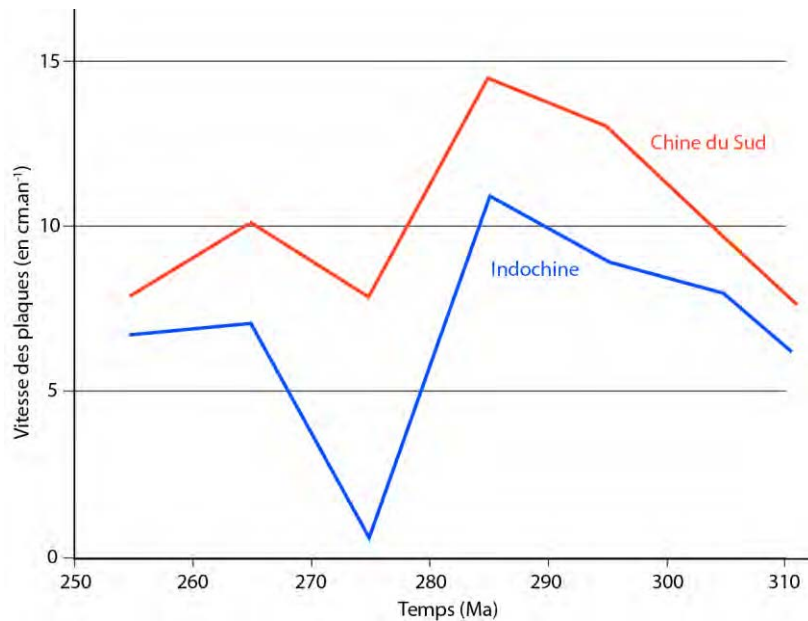
Figure 1.21. Vitesse moyenne (en cm.an -1 , sur un pas de temps de 10 Ma) des plaques Indochine (Annamia) et Chine du Sud au Permien dans le modèle de Domeier et Torsvik (2014).
