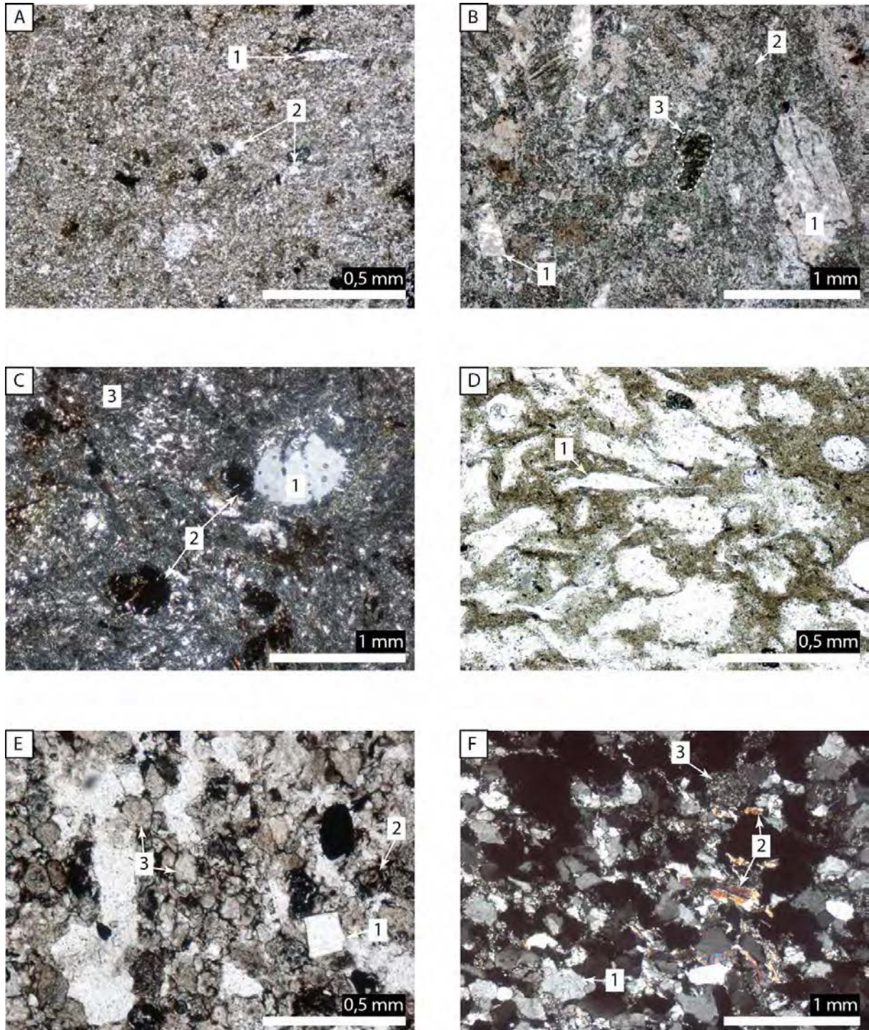
Figure 4.6. Photos de lames minces des formations de Dong Trau et Suoi Bang inférieure, Bassin de Sam Nua.
