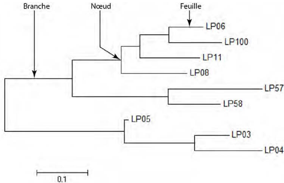
Figure 2.17. Arbre obtenu à partir de la matrice de similarité présentée Figure 14. Cet arbre a été réalisé avec le logiciel MEGA 21 (v. 5.2., Tamura et al., 2011) en utilisant l’algorithme du « Neighbor-Joining ». Le vocabulaire employé pour décrire des arbres (branche, nœud, feuille) y est indiqué.
