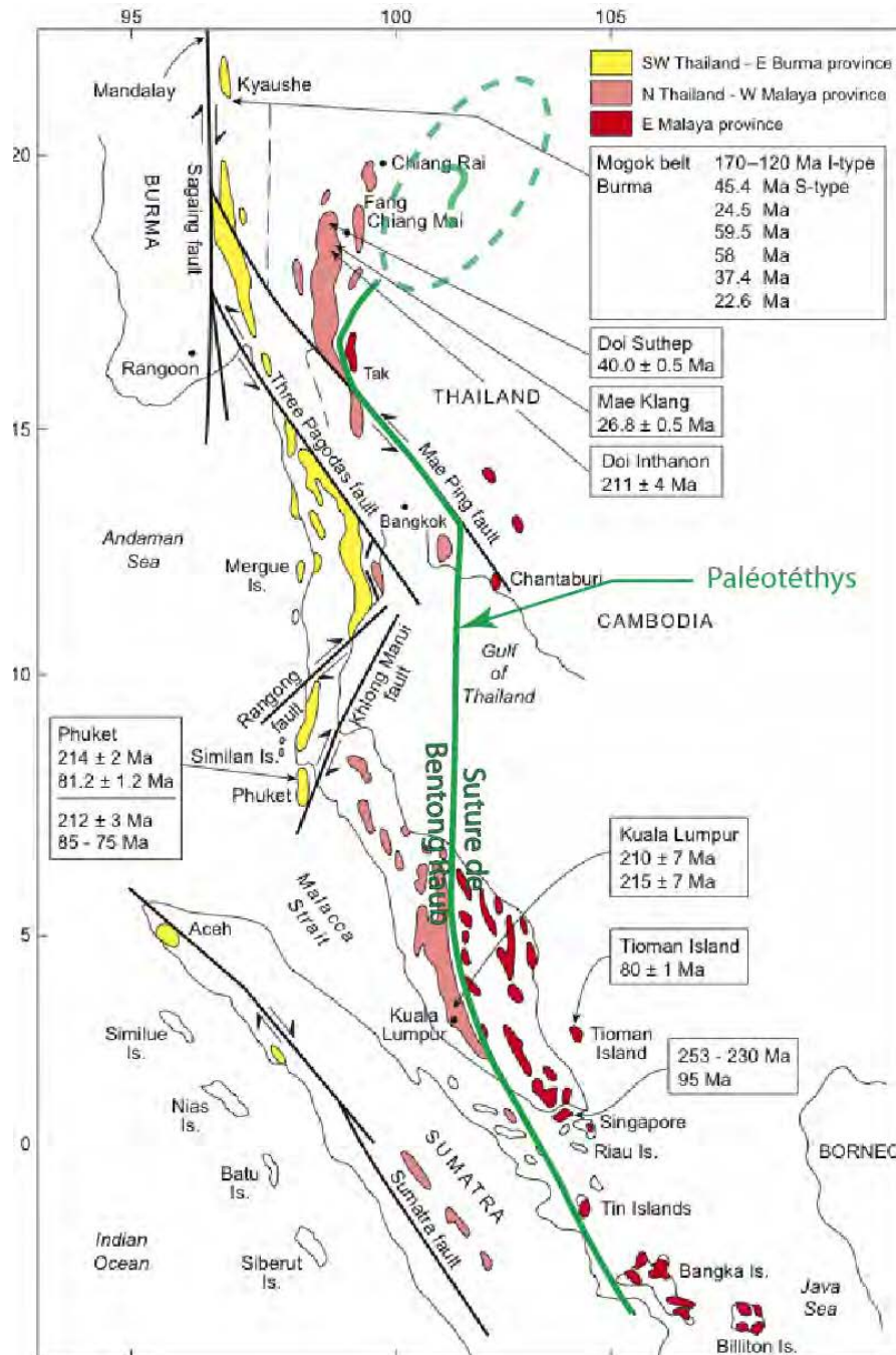
Figure 1.7. Provinces granitiques en Asie du Sud Est. Modifié d'après Searle et al. (2012). La province Sud Ouest Thaïlandaise - Est Birmanie comprend des granites de type I et S. La province Nord Thaïlandaise - Ouest Malaisienne comprend essentiellement des granitoïdes de type S. La province Est Malaisienne comprend essentiellement des granitoïdes de type I. L'ellipse en pointillé souligne la zone du Nord de la Thaïlande - Ouest du Laos pour laquelle les données sur les granitoïdes manquent pour délimiter ces provinces granitiques.
