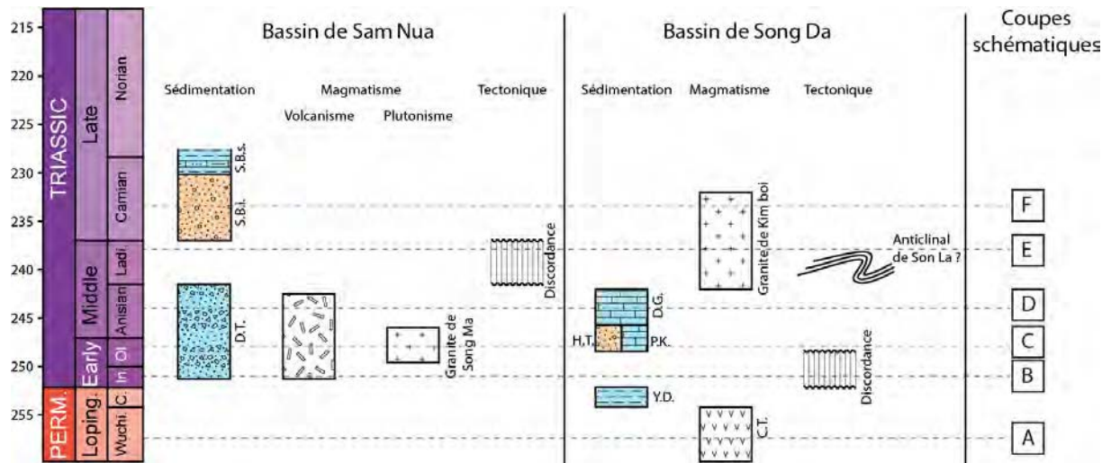
Figure 5.3. Charte synthétique résumant les principaux événements sédimentaires, magmatiques et tectoniques des bassins de Sam Nua et de Song Da et localisation des coupes schématique de la Figures 5.4.
