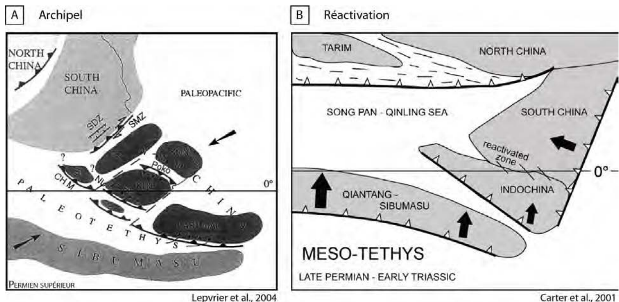
Figure 1.19. Familles de modèles d'évolution géodynamique du domaine Est Téthysien du Permien supérieur - Trias inférieur.
