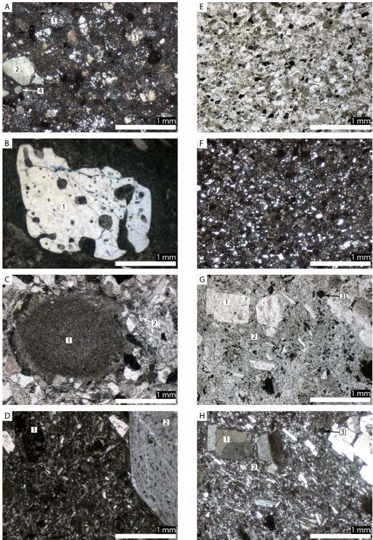
Figure 3.5. Photographies de lames minces des échantillons étudiés de la Formation des Argiles Rouges. Toutes les photographies sont prises en LPA, hormis les images E et G. A, B, C : arénite lithique (échantillon LP 57) (photo A reprise de Blanchard et al., 2013).
