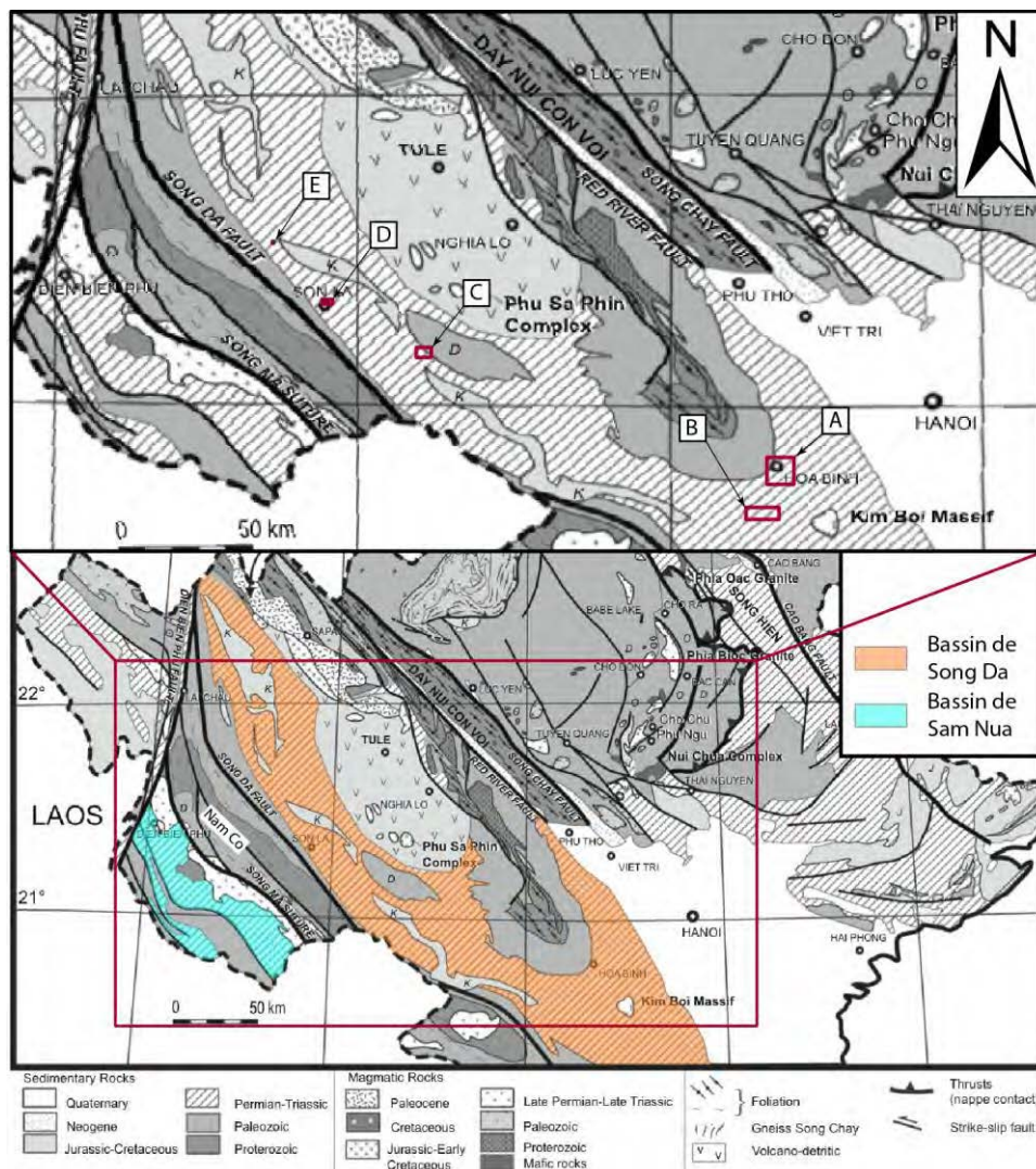
Figure 4.22. Localités étudiées dans le Bassin de Song Da (modifié d'après Roger et al., 2012).
