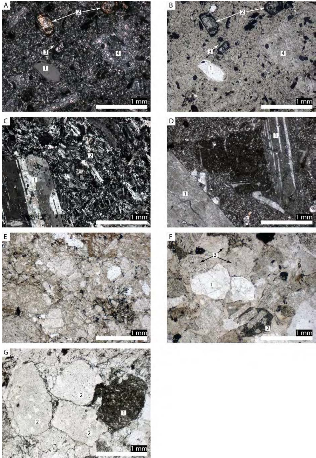
Figure 3.6. Photographies de lames minces d'échantillons représentatifs de la Formation des Tuffites de Luang Prabang.
