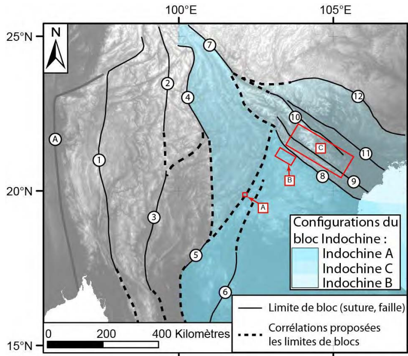
Figure 1.23. Localisation des bassins étudiés dans ce travail dans le bloc Indochine. Configurations du bloc Indochine : voir Figure 1.16 et Tableau 1.6. Limites de bloc : 1 : Mae Yuam, 2 : Changning Menglian, 3 : Inthanon, 4 : Jinghong, 5 : Nan Uttaradit, 6 : Loei, 7 : Ailaoshan, 8 : Song Ma, 9 : Song Da, 10 : Ailaoshan-Fleuve Rouge, 11 : Song Chay, 12 : Babu. Bassins étudiés dans ce travail : A : bassin de Luang Prabang ; B : Bassin de Sam Nua ; C : Bassin de Song Da.
