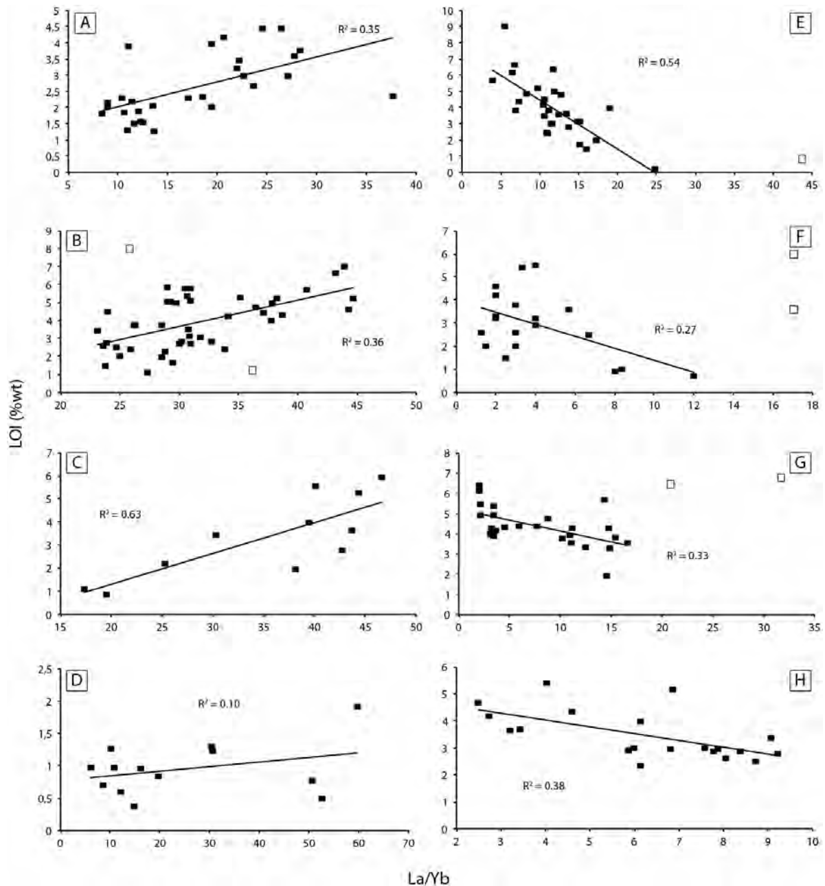
Figure 6. Evolution du rapport La/Yb pour différentes séries magmatiques calco-alcalines triasiques du domaine Est Téthysien (sauf E) en fonction de l'altération.
