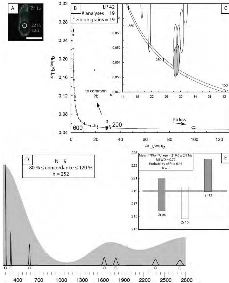
Figure 3.21. Analyses géochronologiques de l'échantillon LP 42.
