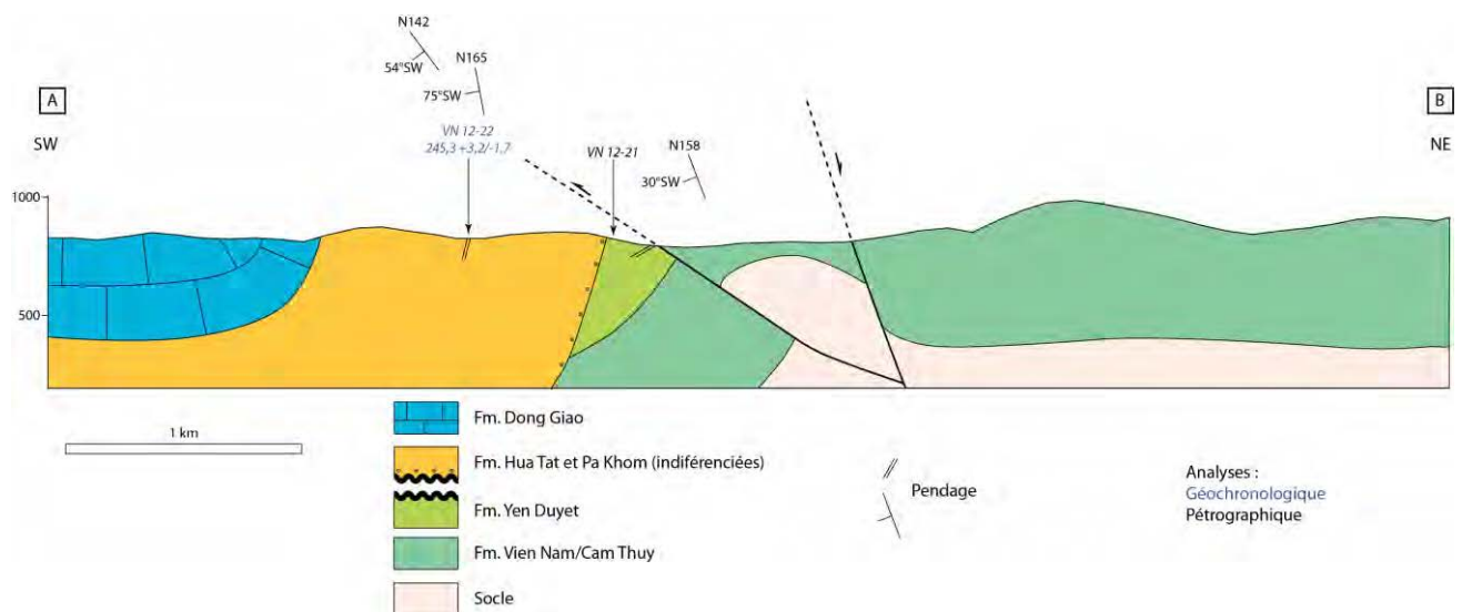
Figure 4.35. Coupe de Mai Son. Basé sur la carte révisée de la localité de Mai Son (Figures 4.22 et 4.23) selon le profil A-B (Figure 4.23).
