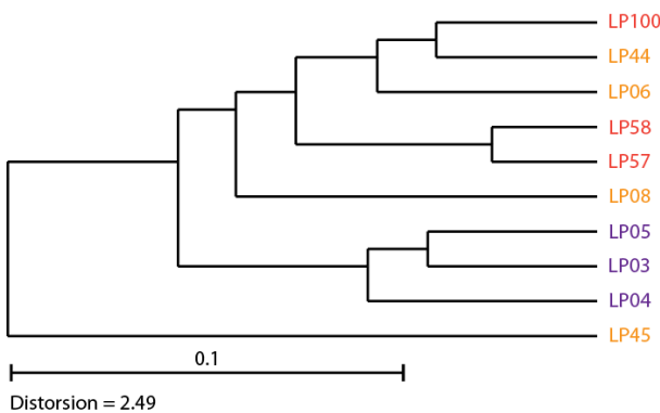
Figure 3.27. Influence de l'algorithme sur le regroupement opéré. NJ : Neighbor Joining , UPGMA : Unweighted Pair Group Method using arithmetic Averages .
