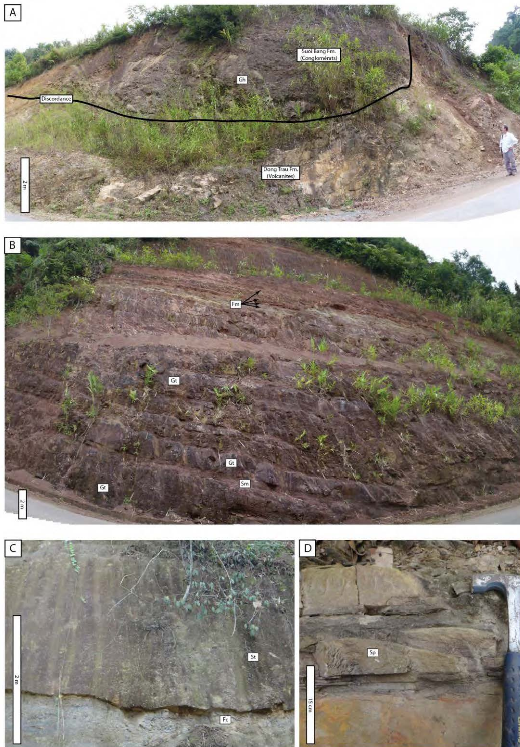
Figure 4.9. Formation de Suoi Bang inférieure. A. Discordance séparant les formations Suoi Bang inférieure et Dong Trau, B. Faciès représentatifs de la base de la Formation Suoi Bang inférieure, C., D. Faciès représentatifs de la Formation Suoi Bang.
