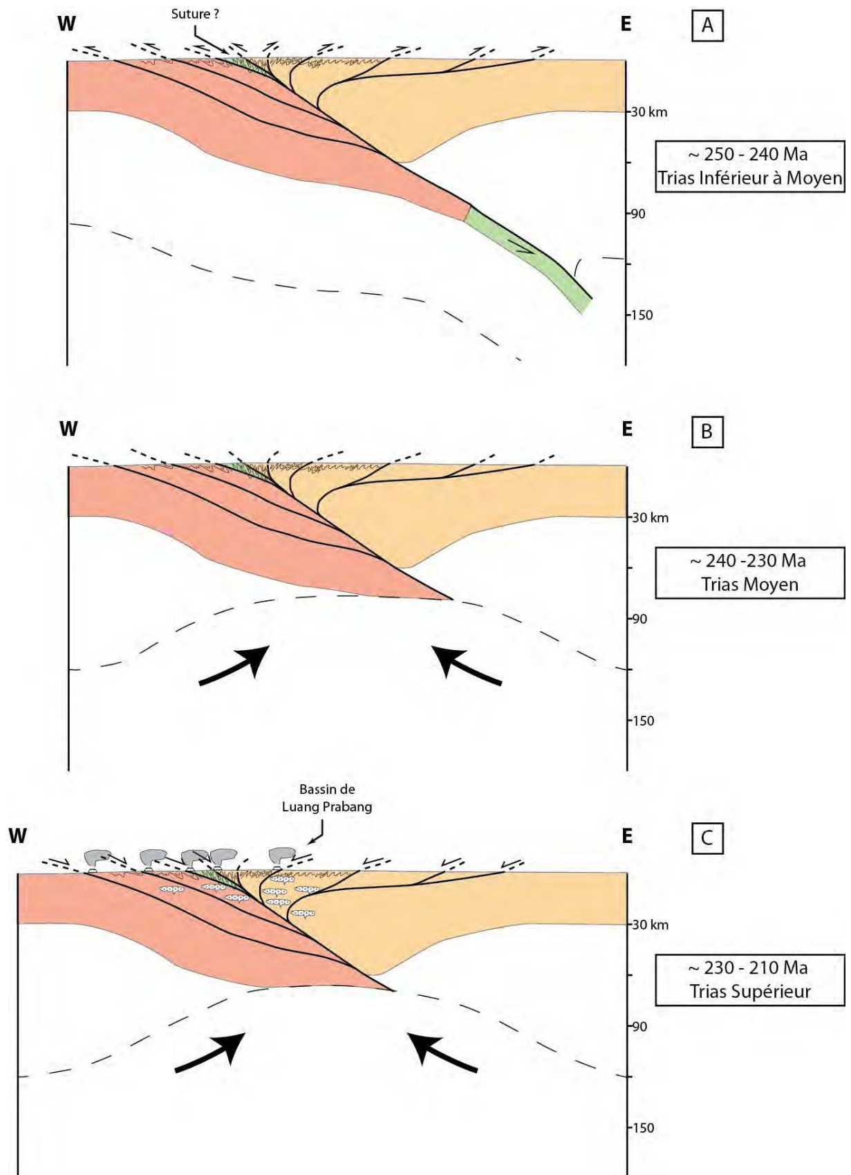
Figure 5.12. Proposition de modèle géodynamique pour le Bassin de Luang Prabang et sa périphérie envisageant une collision au Trias inférieur.
