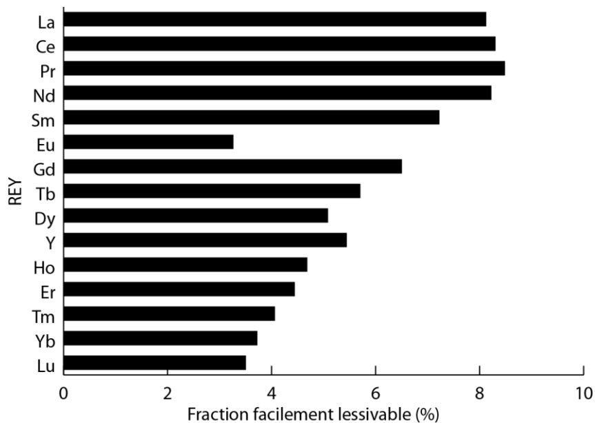
Figure 3. Fraction facilement lessivable d'une andésite fraîche. Condition expérimentale : lessivage d'1 gramme d'andésite fraîche broyée par de l'eau distillée à 70°C pendant 1 heure et en présence d'une résine échangeuse de cations. Modifié d'après Bau et al., 1998.
