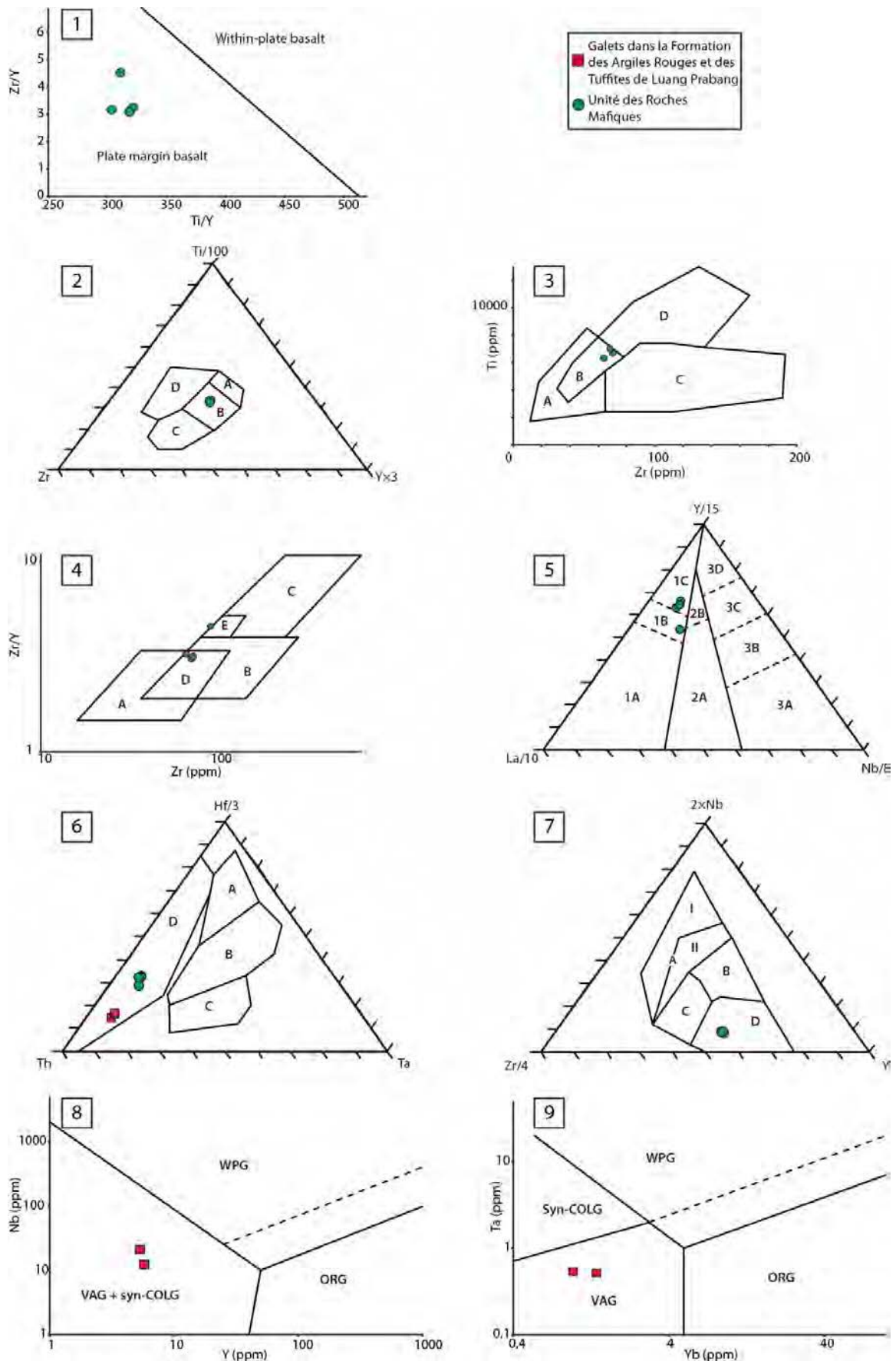
Figure 3.38. Diagrammes de discrimination « classiques » pour les roches volcaniques du Bassin de Luang Prabang.
