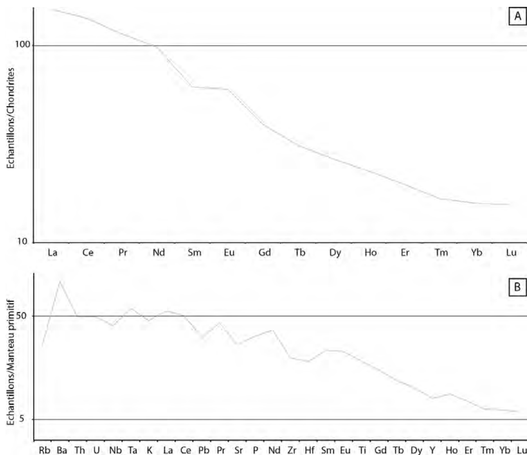
Figure 4.51. Spectre de Terres Rares (REE) et multi-élémentaire de l'échantillon VN 12-49. A. Spectre REE normalisé aux chondrites (valeurs de normalisation : Sun S.-S. et McDonough, 1989). B. Diagramme multi-élémentaire normalisé au manteau primitif (valeurs de normalisation : Sun S.-S. et McDonough, 1989).
