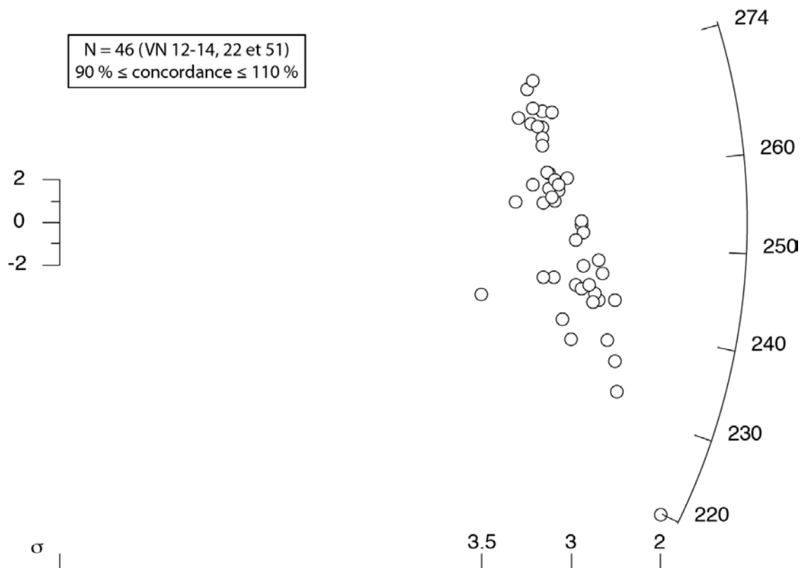
Figure 4.33. Diagramme radial de l'ensemble des analyses concordantes obtenues sur les échantillons de roche sédimentaire de la Formation de Hua Tat.
