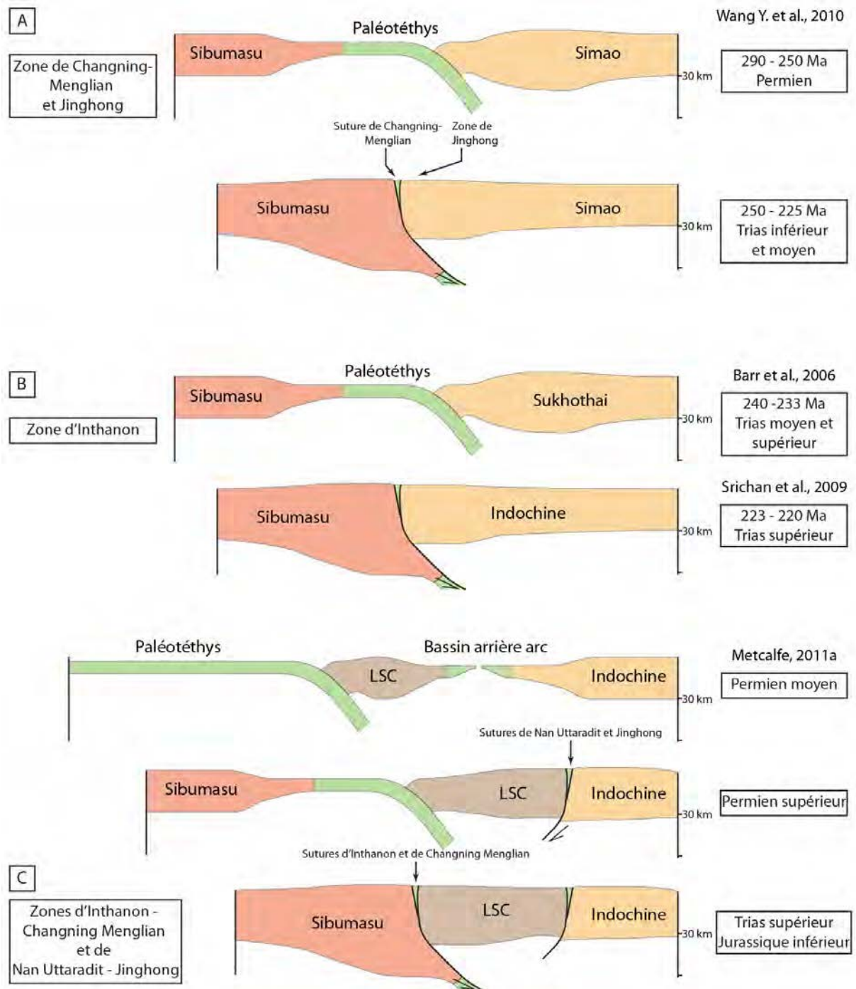
Figure 5.6. Principaux modèles d'évolution géodynamiques proposés pour les zones de Changning Menglian, Jinghong, Inthanon et Nan Uttaradit. Les lettres indiquent la position approximative des coupes sur le schéma 5.5. Les blocs indiqués sont ceux mentionnés dans les publications sélectionnées (cf. section 3.1, Chapitre 1). LSC : Lincang - Sukhothai - Chanthaburi.
