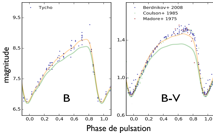
FIGURE 2.6 – Exemple de l’effet de la présence d’un compagnon chaud dans la photométrie en B et B - V de U Car. En jaune : modèle sans compagnon. En vert : modèle obtenu en introduisant un compagnon.
