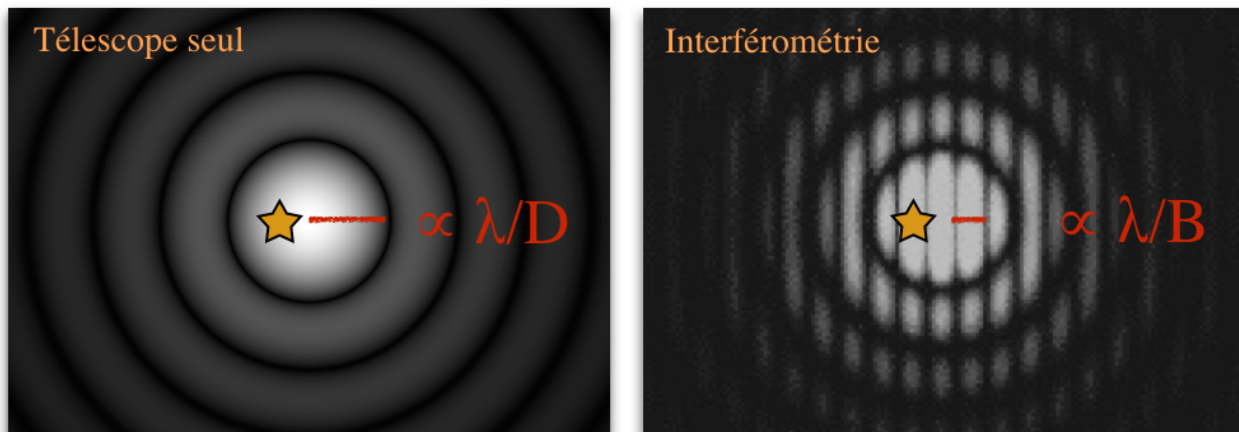
FIGURE 1.22 – La limite de résolution d'un télescope simple est inversement proportionnelle au diamètre D du miroir primaire (taille de la tâche d'Airy), alors que la résolution théorique d'un interféromètre est inversement proportionnelle à la base B séparant les deux télescopes utilisés (taille des franges sur le ciel). Cette technique instrumentale permet donc d'atteindre plus facilement une plus grande résolution.
