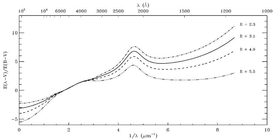
FIGURE 2.3 – Courbes d’extinction (allant de l’infrarouge lointain jusqu’aux UV) obtenues pour différentes valeurs du paramètre R_V . Ce graphique est issu du papier de Fitzpatrick (1999) .
