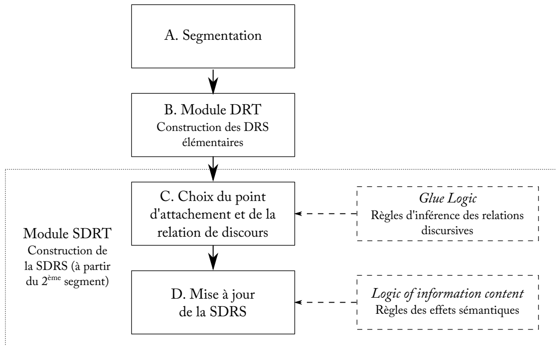
FIGURE 4.5 – Étapes de la construction de la représentation du discours en SDRT
