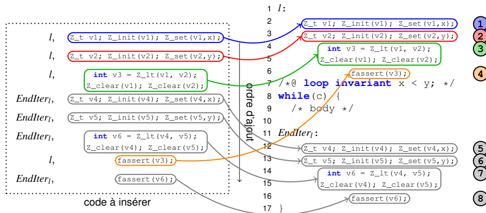
FIGURE 4.3 – Insertion du code généré pour l'invariant de la figure 4.2
