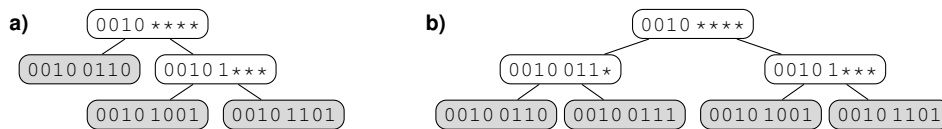
FIGURE 5.4 – Exemple de Patricia trie avant (a) et après (b) insertion de 0010 0111
