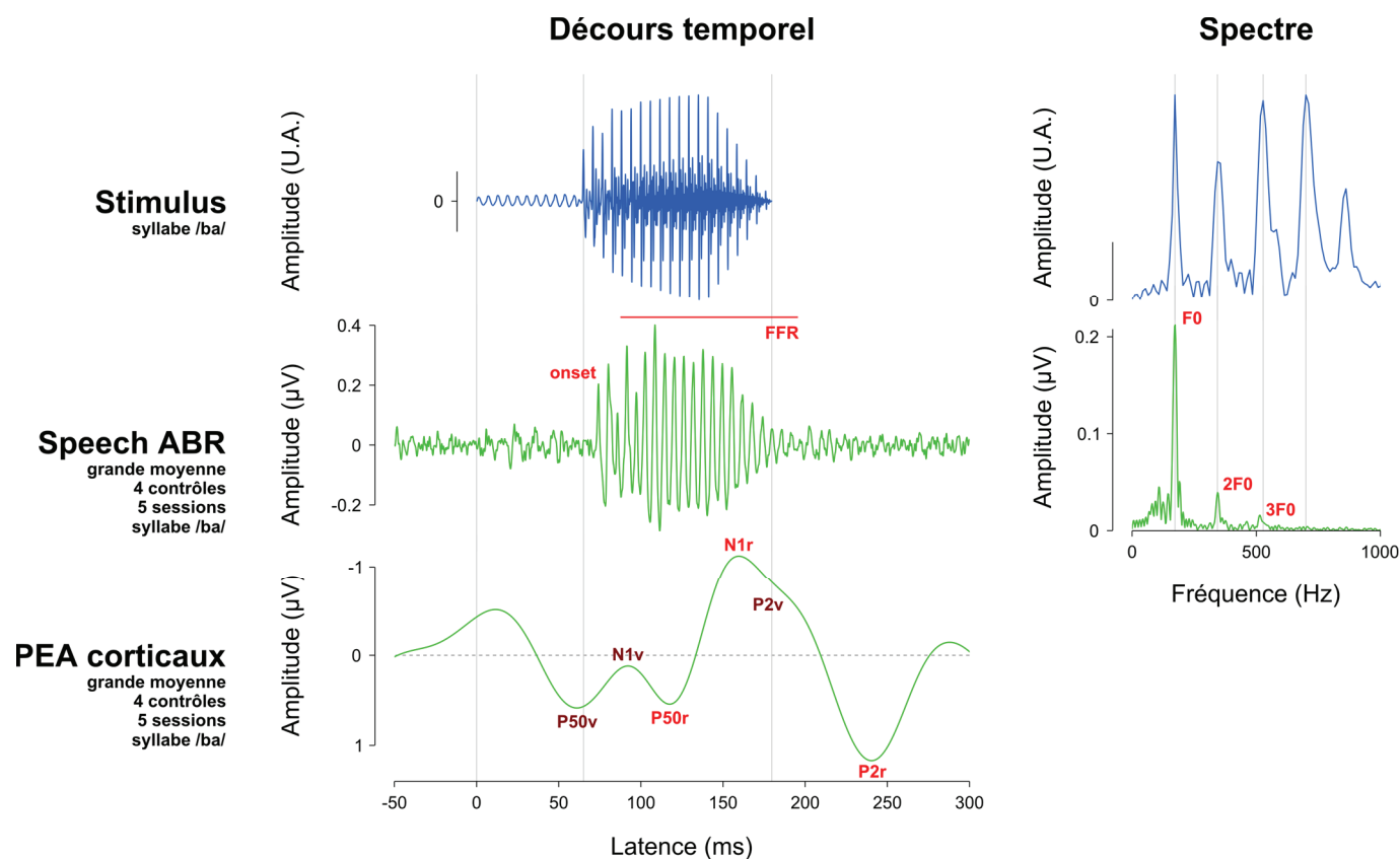
Figure 8. Grande moyenne des Speech ABR et PEA corticaux à la syllabe ba pour le groupe contrôle. Pour la Speech ABR, la moyenne est composée de 38046 essais (4 contrôles x 5 sessions x 2000 essais par
