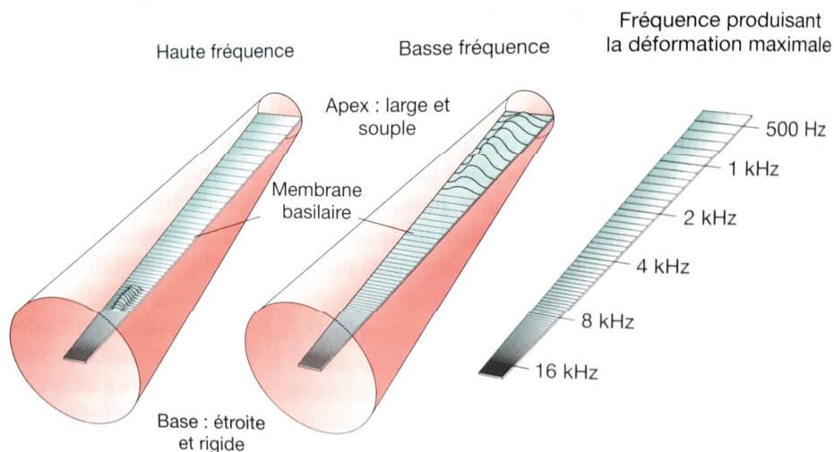
Figure 2.11. Membrane basilaire et origine de la tonotopie (Bear et al. , 2007). La fenêtre ovale, « l'entrée » du signal sonore dans la cochlée, se situe au niveau de la base. L'hélicotremme n'est pas représenté ici.
