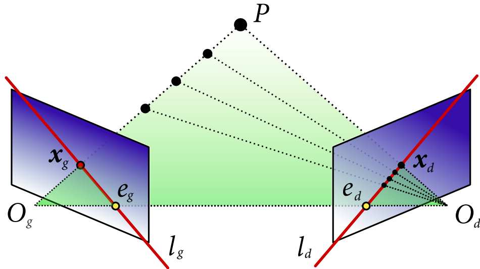
FIGURE 6.3 : Géométrie épipolaire.
