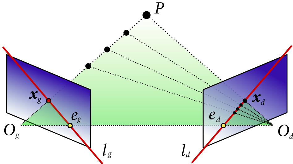
FIGURE 6.3 : Géométrie épipolaire.
