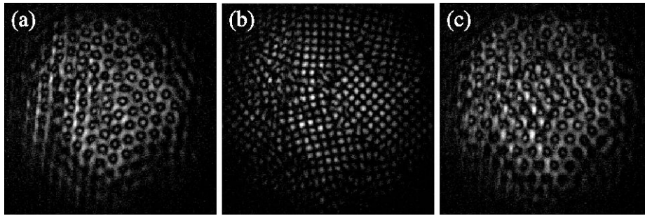
FIGURE 2.32 – Impact de B_z : transition carrés-hexagones. B_x = B_y = 0 . (a) B_z = -0,2 G; (b) B_z = 0 ; (c) B_z = +0,2 G. Paramètres : I = 12,4 \text{mW}/\text{cm}^2 , \delta = -7,8 \Gamma , t_{\text{pump}} = 200 \mu\text{s} .
