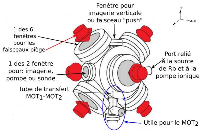
FIGURE 1.13 – Architecture de l'enceinte à vide avec ses différents ports (voir texte).
