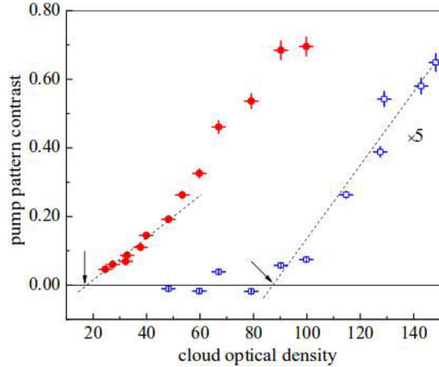
FIGURE 2.21 – Seuils en densité optique des instabilités électronique ( t_{pump} = 1 \mu\text{s} , carrés bleus) et opto-mécanique ( t_{pump} = 200 \mu\text{s} , points rouges). I = 487 \text{ mW}/\text{cm}^2 et \delta = 6 \Gamma . Source : Supplément [51]
