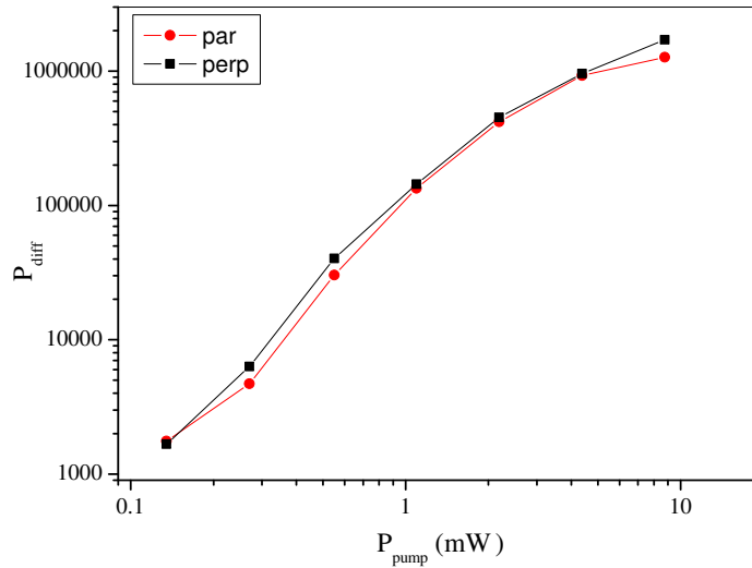
FIGURE 2.42 – Puissance diffracté dans le canal \perp en fonction de la puissance des pompes. Paramètres : \delta = -5,71 \Gamma ; t_{\text{pump}} = 200 \mu\text{s} .
