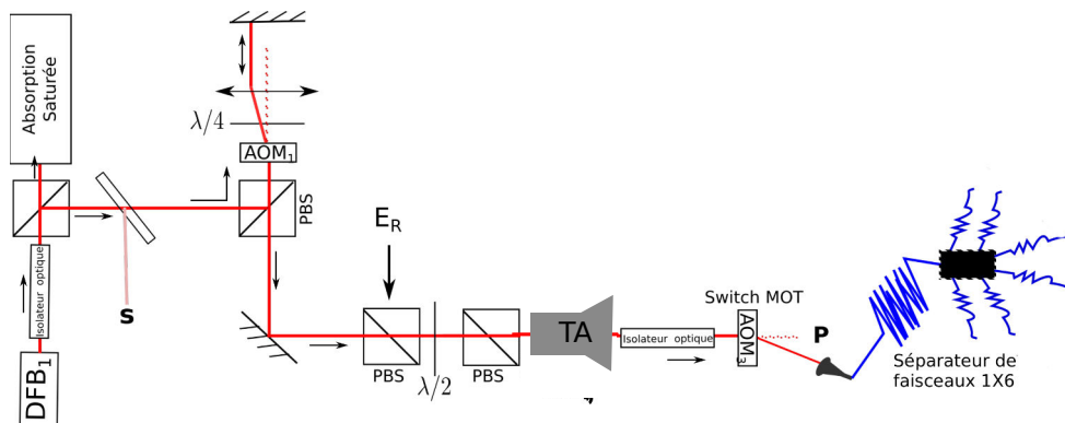
FIGURE 1.8 – Schéma descriptif du système de génération des faisceaux "MOT". Un AOM est utilisé pour contrôler la fréquence et l'amplitude du faisceau émis par le DFB 1 . Un amplificateur TA de 2,5 W est utilisé pour fournir assez de puissance pour le MOT, avant l'injection du faisceau dans un fibre séparateur 1x6. Les faisceaux S et P servent respectivement à générer les faisceaux sonde et pompe, alors que l'entrée E R est utilisée pour mélanger du repompeur aux faisceaux "MOT" (voir la suite).
