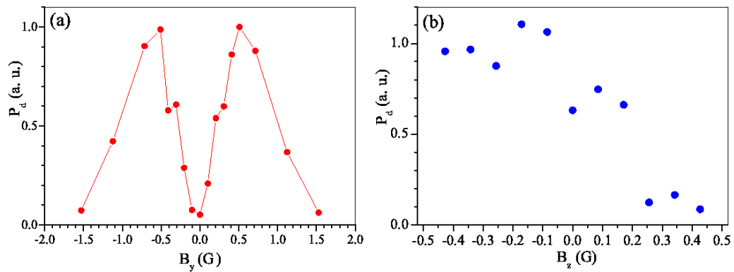
FIGURE 2.43 – Puissance diffractée en fonction du champ magnétique : (a) P_d vs B_y ( B_x = B_z = 0 ) (b) P_d vs B_z ( B_x = B_y = 0 ). Paramètres : I = 24 \text{ mW}/\text{cm}^2 , \delta = -7.8 \Gamma .
