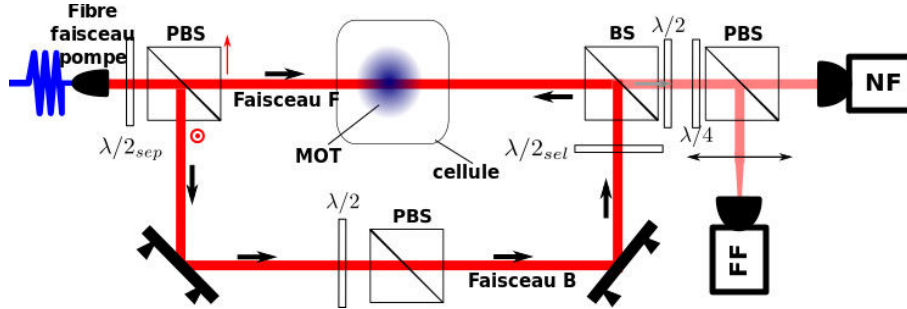
FIGURE 2.7 – Montage expérimental pour l'étude des instabilités avec deux faisceaux (pompes) indépendants contra-propageants. \lambda/2_{sep} permet de séparer le faisceau en deux et \lambda/2_{sel} permet de sélectionner la polarisation du faisceau B.
