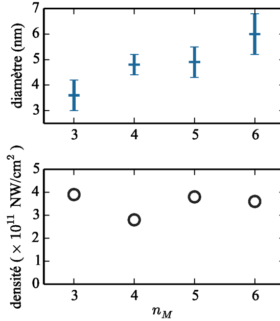
FIGURE 2.2: Diamètre et densité des fils pour les échantillons (\text{STO12|M6})_{40}^A , (\text{STO12|M5})_{40}^A , (\text{STO12|M4})_{40}^A et (\text{STO12|M3})_{40}^A en fonction du nombre de tirs sur la cible de l'oxyde du métal des nanofils. En croix bleues, le diamètre. En cercles noirs, la densité.
