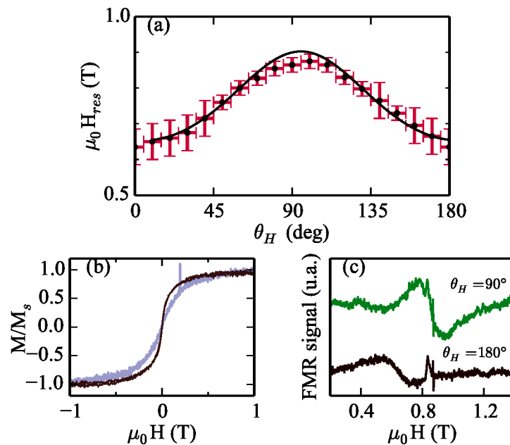
FIGURE 4.13: Mesures magnétiques réalisées sur l'échantillon (\text{STO6|M1})_{00} à T = 300 K. Champs de résonance ferromagnétique en fonction de l'angle polaire \theta (voir figure 4.1 pour la définition des angles). (b) Cycles d'hystérésis hors-plan (trait fin noir) et dans le plan (trait bleu clair épais). (c) Deux exemples de courbes de résonance ferromagnétique, pour \theta_H = 90^\circ et \theta_H = 180^\circ
