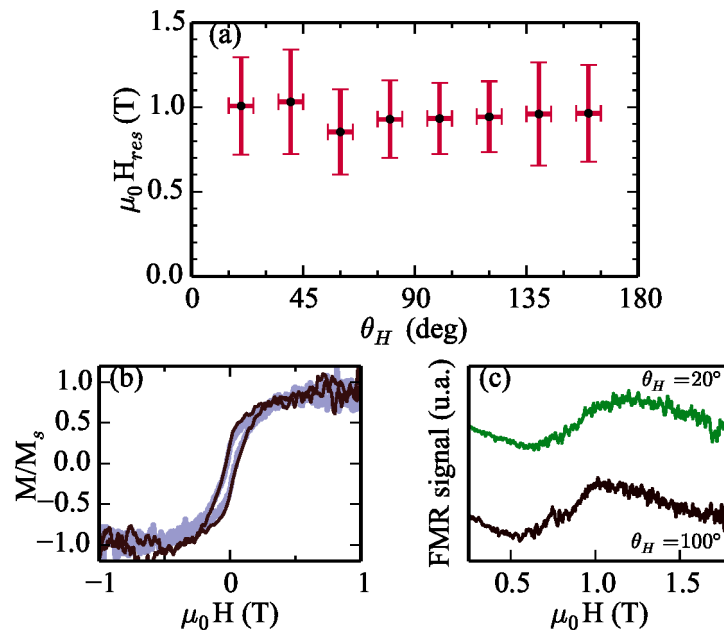
FIGURE 4.12: Mesures magnétiques réalisées sur l'échantillon (\text{STO6|M1})_{00} à T = 20 K. Champs de résonance ferromagnétique en fonction de l'angle polaire \theta (voir figure 4.1 pour la définition des angles). (b) Cycles d'hystérésis hors-plan (trait fin noir) et dans le plan (trait bleu clair épais). (c) Deux exemples de courbes de résonance ferromagnétique, pour \theta_H = 20^\circ et \theta_H = 100^\circ
