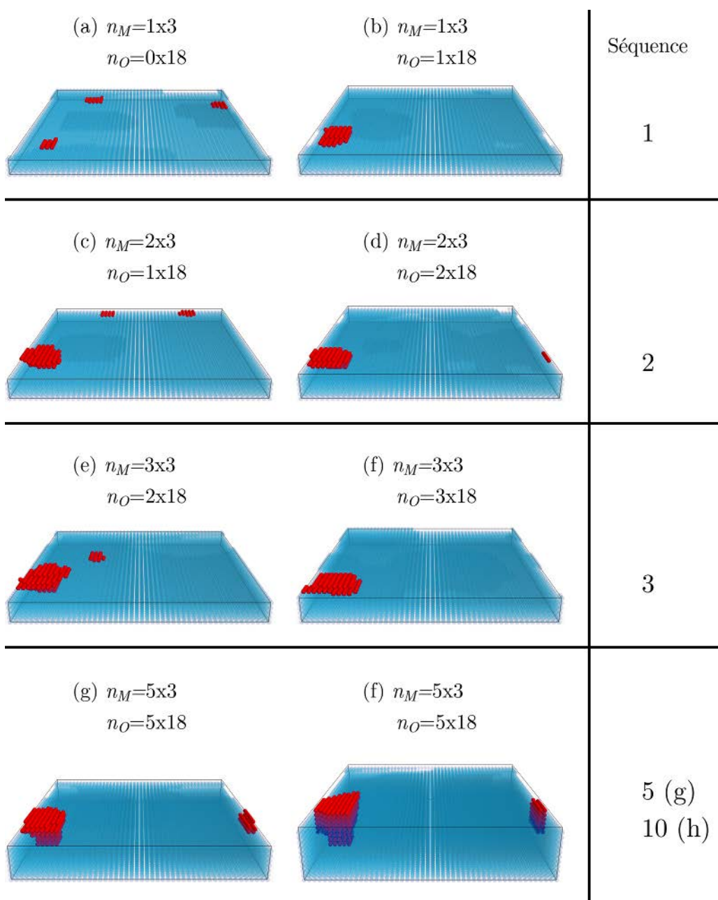
FIGURE 2.8: Étapes successives lors de la simulation de la croissance d'un nanofil en matrice. La cellule fait (50 \times 50) sites. La température de croissance est T = 870 K. La séquence de dépôt est (18 - 3) . Huit situations sont montrées. Pour chacune d'elle, le nombre de tirs qu'il y a eu jusque là sur chaque cible est indiqué, en multiples de la séquence, n_M est le nombre de tirs sur la cible de l'espèce A, n_O est le nombre de tirs sur la cible de l'espèce B. (a) État du système après les trois premiers dépôts de A. (b) État du système après trois dépôts de A et dix-huit dépôts de B. C'est la situation à la fin de la première séquence. (c) État du système après les trois dépôts de A de la deuxième séquence. Il y a donc eu 2 \times 3 = 6 dépôts de l'espèce A au total. (d) État du système après les dix-huit dépôts de l'espèce B de la deuxième séquence. Il y a donc eu 2 \times 18 = 36 dépôts d'espèce B. C'est la situation à la fin de la deuxième séquence. (e) Situation après le dépôt de A de la troisième séquence. (f) Situation à la fin de la troisième séquence. (g) Situation à la fin de la cinquième séquence. (h) Situation à la fin de la dixième séquence.
