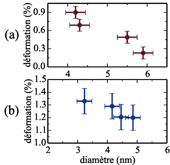
FIGURE 3.4: Dépendance de la dilatation des nanofils avec leur diamètre dans deux cas : (a) fils de nickel dans une matrice de cérium; (b) fils de \text{Co}_{0.4}\text{Ni}_{0.6} dans une matrice de titanate de strontium et de baryum.
