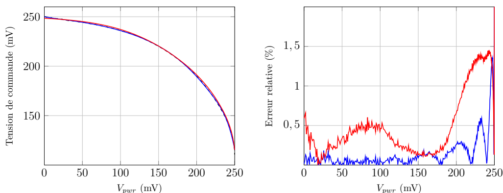
FIGURE III.5.6 – Approximation par réseau de neurones intégré de la tension de commande du déphaseur associée au HPA TEDCNES en fonction de V_{pwr} . A gauche : caractéristiques idéale (pointillés), issue du réseau de neurones mathématique (en bleu) et issue du réseau de neurones intégré (en rouge) A droite : erreur relative de modélisation par réseau de neurones mathématique (en bleu) et par réseau de neurones intégré (en rouge)
