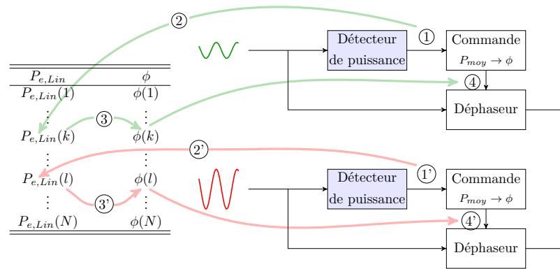
FIGURE II.2.8 – Etapes de la prédistorion en phase permettant d’appliquer au déphaseur la consigne de déphasage correcte. Le raisonnement (1') \rightarrow (2') \rightarrow (3') \rightarrow (4') est identique au raisonnement (1) \rightarrow (2) \rightarrow (3) \rightarrow (4) mais pour un signal de plus grande amplitude
