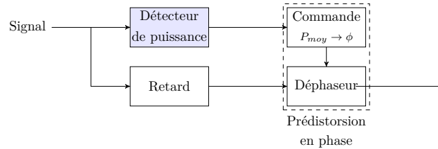
FIGURE II.2.9 – Module de prédistorion en phase avec retard
