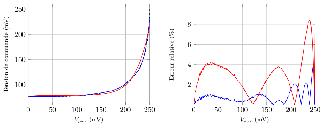
FIGURE III.5.2 – Approximation par réseau de neurones intégré de la tension de commande du VGA associée au HPA TEDCNES en fonction de V_{pwr} A gauche : caractéristiques idéale (pointillés), issue du réseau de neurones mathématique (en bleu) et issue du réseau de neurones intégré (en rouge) A droite : erreur relative de modélisation par réseau de neurones mathématique (en bleu) et par réseau de neurones intégré (en rouge)
