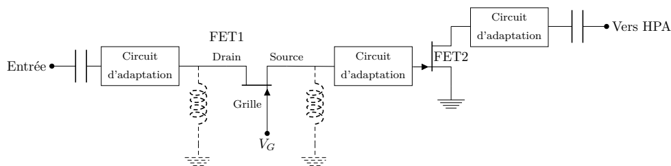
FIGURE B.10 – Prédistorion à base de transistors montés en cascode
