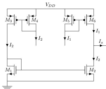
FIGURE III.3.14 – Conversion d'un courant différentiel en courant asymétrique
