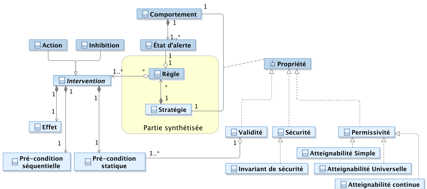
FIGURE 3.4 – Méta-modèle
