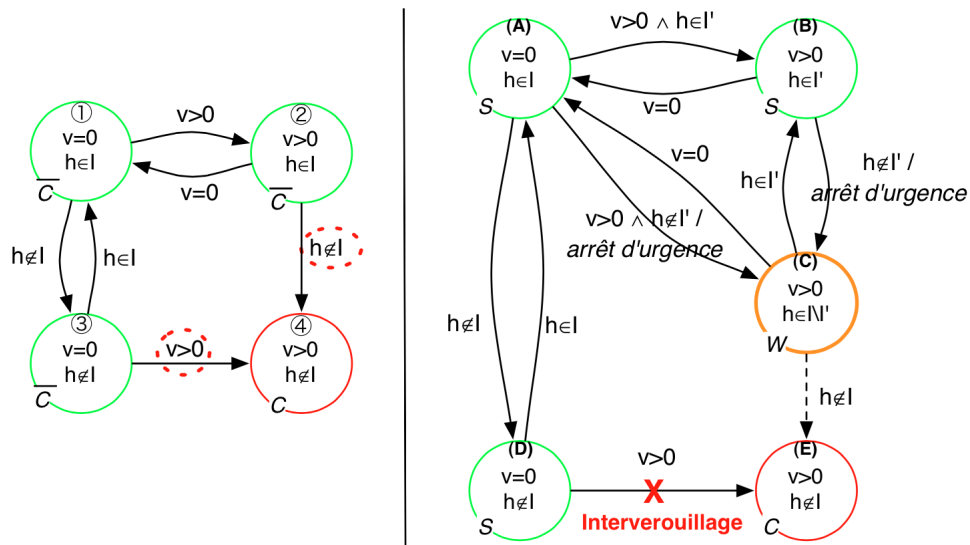
FIGURE 1.4 – Traitement de l’invariant «Les poignées doivent être à la bonne hauteur». L’invariant est formalisé avec les variables observables v , la vitesse, et h la hauteur des poignées. Sur le graphe de gauche, les transitions menant dans l’état catastrophique sont entourées en pointillées. Pour celle correspondant à un changement de hauteur, une marge peut être prise, ce qui explique le partitionnement de l’état 2 pour donner les états (B) et (C). Une intervention, l’arrêt d’urgence, est déclenchée lors de l’entrée dans l’état de marge. La deuxième transition vers l’état catastrophique est traitée par un interverrouillage, qui, en bloquant les roues, empêche le démarrage.
