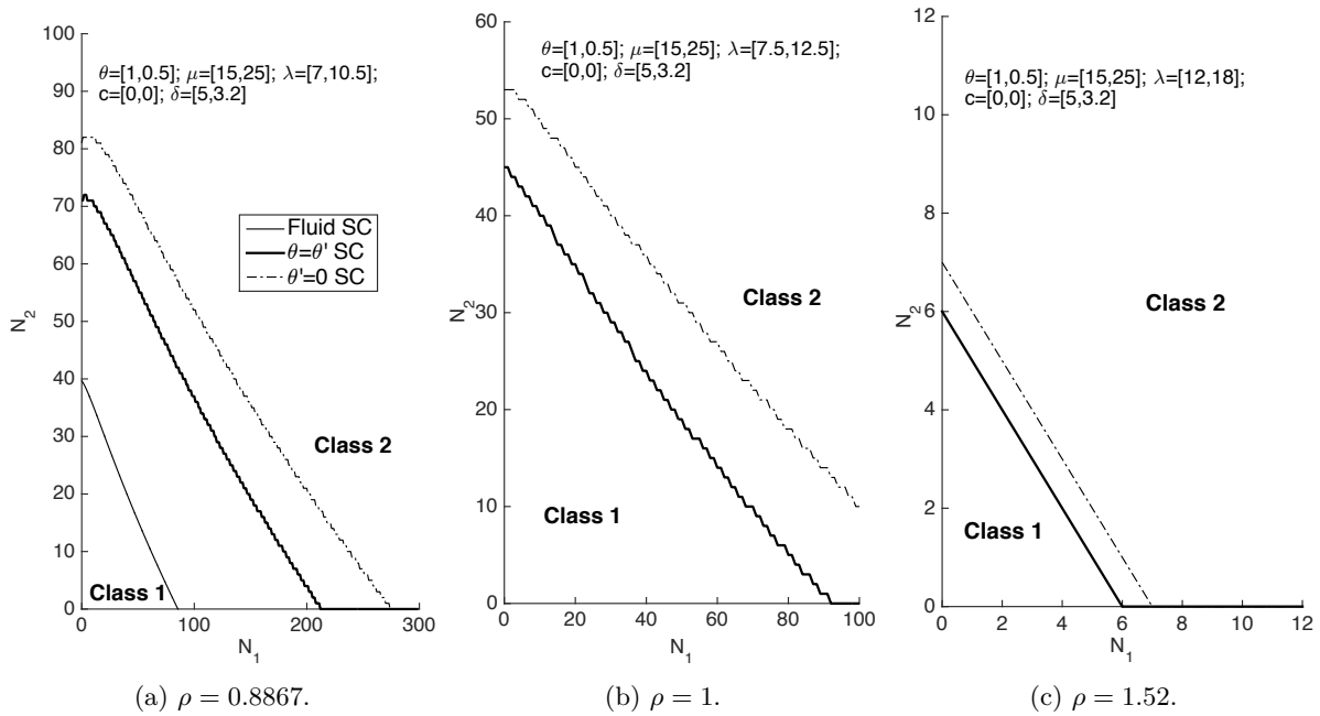
Irudia 5.8: 2. Adibideko trukatzefuntzioen konparaketa.
