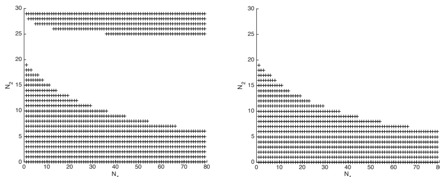
Irudia 1.3: Value iteration bidez lortutako emaitza zerbitzari-barkardun bi-klasetako ilara batentzat, bezeroak abandonatzen dutenean. “+”zeinua duen eremuan 1 klaseko bezeroak dute lehentasuna eta zeinurik gabeko eremuan 2 klaseko bezeroak. Ezkerreko irudian muga efektua ikus daiteke L_1 = 80, L_2 = 30 trun-kazio parametrotarako. Eskuineko irudian ez dago muga efekturik eta mozte parametroak L_1 = L_2 = 100 dira.
