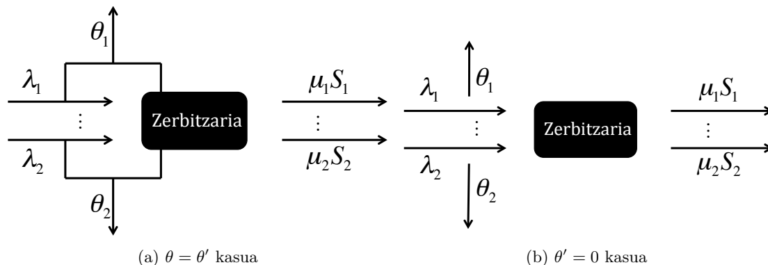
Irudia 5.1: Uzteak gerta daitezkeen ilara zerbitzari-bakar klase-anitza
