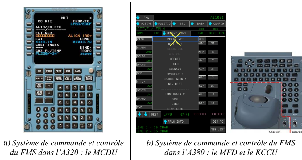
Figure 1.6. Évolution du système de commande et contrôle du FMS entre les glass cockpits (a) et les cockpits interactifs (b)
