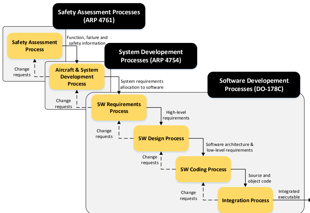
Figure 3.18. Processus de développement logiciel de la norme DO-178C
