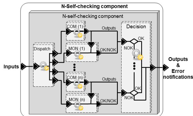
Figure 6.2. Architecture logicielle d'un composant n -autotestable
