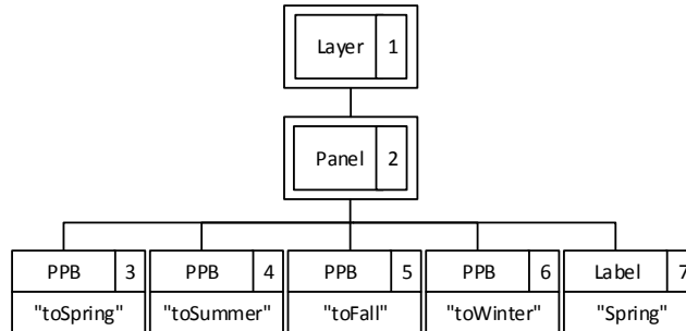
Figure 5.17. Arbres des widgets de l'application des quatre saisons
