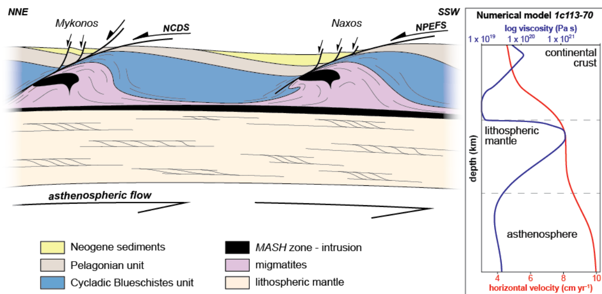
Figure 6.6 : coupe schématique montrant l'exhumation du dôme métamorphique des Cyclades (i.e. dômes de Mykonos et de Naxos), accompagnée par de grands systèmes de détachements. NCDS : North Cycladique Detachment System . NPEFS : Naxos-Paros Extensional Fault System . La déformation extensive dans cette lithosphère affaiblie par la présence de roches partiellement fondues (i.e. zone MASH , migmatites, intrusions) est contrôlée, en partie, par les flux asthénosphériques sous-jacents, comme le suggère le profil de viscosité et de vitesse obtenu à partir des modèles réalisés (cf. Chapitre 5 ), où la vitesse horizontale dans l'asthénosphère est transmise à la lithosphère.
