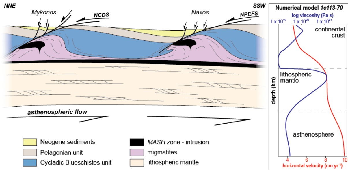
Figure 6.6 : coupe schématique montrant l'exhumation du dôme métamorphique des Cyclades (i.e. dômes de Mykonos et de Naxos), accommodée par de grands systèmes de détachements. NCDS : North Cycladique Detachment System . NPEFS : Naxos-Paros Extensional Fault System . La déformation extensive dans cette lithosphère affaiblie par la présence de roches partiellement fondues (i.e. zone MASH , migmatites, intrusions) est contrôlée, en partie, par les flux asthénosphériques sous-jacents, comme le suggère le profil de viscosité et de vitesse obtenu à partir des modèles réalisés (cf. Chapitre 5 ), où la vitesse horizontale dans l'asthénosphère est transmise à la lithosphère.
