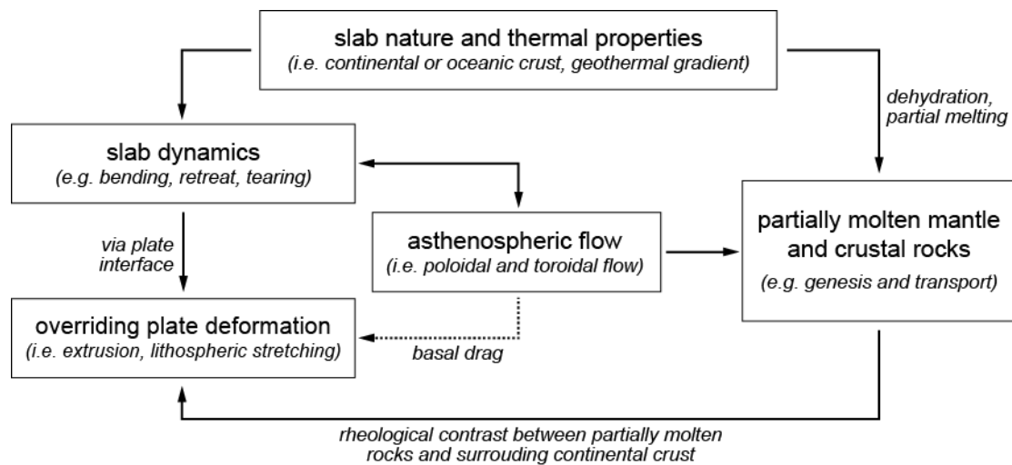
Figure 5.3 : schéma synthétisant l'ensemble les liens (i.e. contrôles et interactions) qui sont mis en évidence à partir de l'observation des modèles numériques 3D entre la dynamique mantellique et crustale d'une zone de subduction et les processus de genèse et transport de roches partiellement fondues (i.e. sources des magmas).
