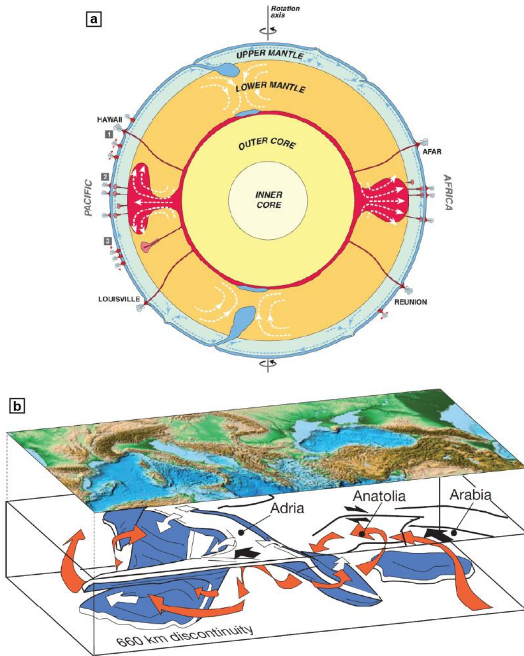
Figure 1.20 : la convection mantellique à différentes échelles. (a) Coupe schématique de la Terre montrant la dynamique mantellique caractérisée par de grandes cellules de convection dans le manteau supérieur et inférieur. [Courillot et al. , 2003]. (b) Bloc schématique de la géométrie des zones de subduction en profondeur et des flux asthénosphériques associés dans la région Méditerranéenne [Faccenna & Becker, 2010].
