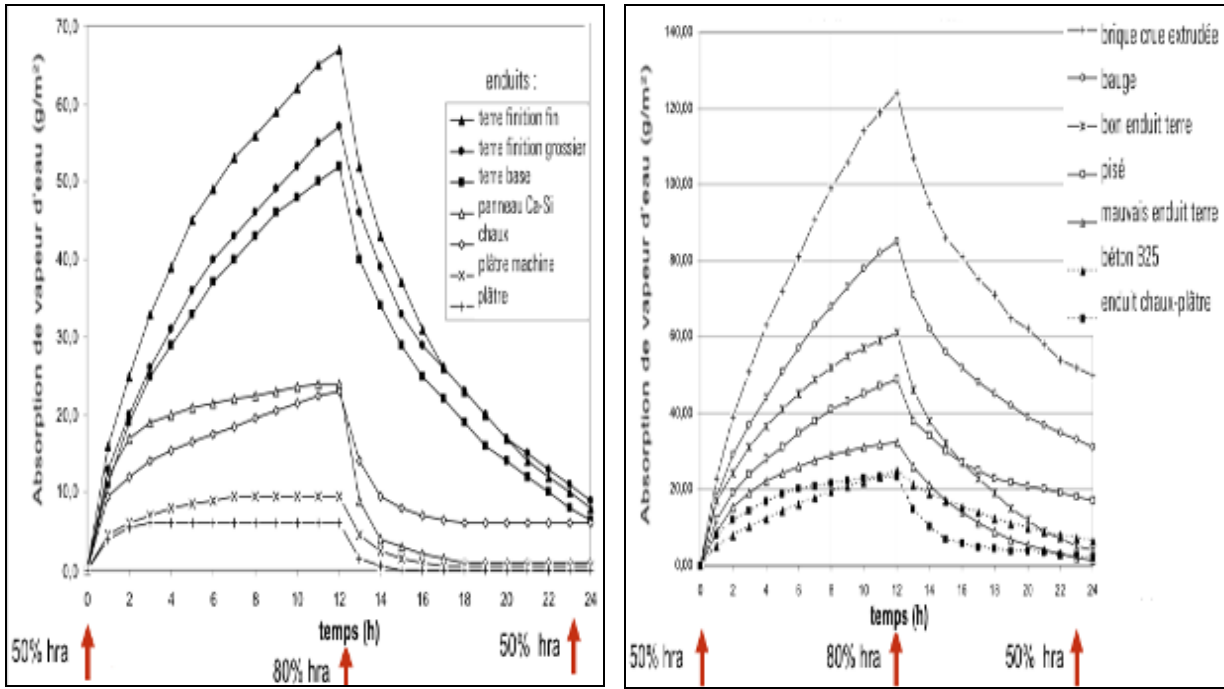
Figure 3.3. Courbes d'absorption et de désorption pour des échantillons de 1,5 cm d'épaisseur – Humidité relative de l'air (50/80/50) à T= 21°C
