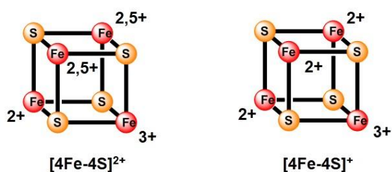
Figure II-3-d-1 : Représentation schématique de la valence de chaque atome de Fer d'un centre [4Fe-4S] « atypique » à l'état oxydé (gauche) et réduit (droite).
