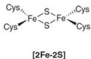
Figure II-2-a : Structure chimique d'un centre [2Fe-2S] (Fontecave et al. 2006).
