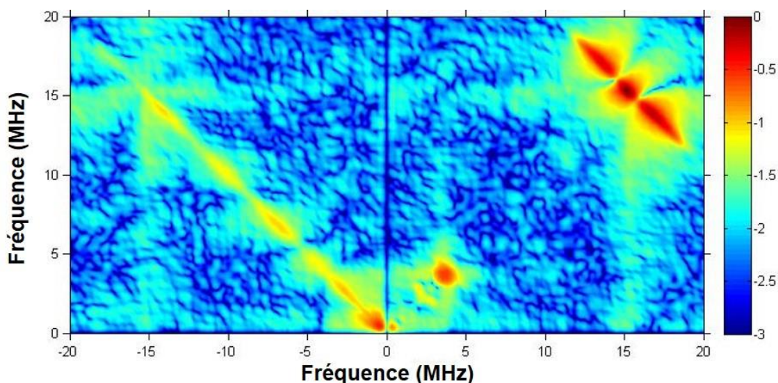
Figure I-3-d-2 : Spectre RPE HSCORE du mutant RimO-S. L'échantillon analysé contient 80 \mu\text{L} à 575 \mu\text{M} d'holoprotéine réduite. La réduction est réalisée par incubation avec 10 équivalents de dithionite pendant 30 minutes. Les conditions d'enregistrements de ce spectre sont : Température = 8 K / Champ magnétique = 3580 G / Fréquence = 9,71 GHz / Transformée de Fourier 2D.
