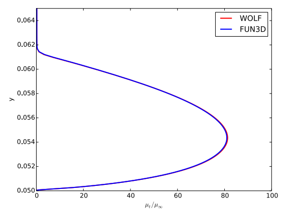
(d) Nondimensional eddy viscosity at x = 0.75 .
