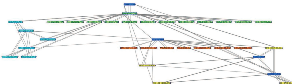
Figure 2.14 : Communautés d'acides aminés détectées par le clustering spectral
