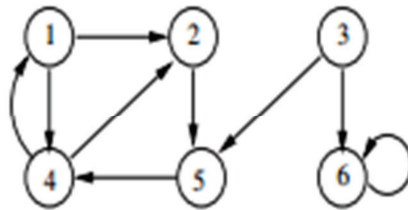
Figure 2.1 : Exemple d'un graphe orienté
