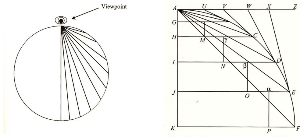
Figure 64. Méthode proposée par Leibniz pour le calcul de la surface du cercle
