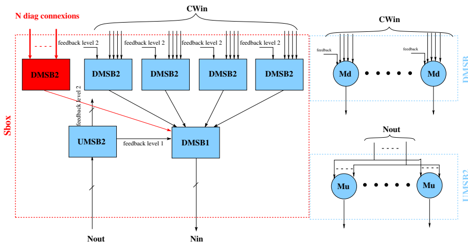
FIGURE 4.5 – Impact des connexions diagonales sur la criticité
