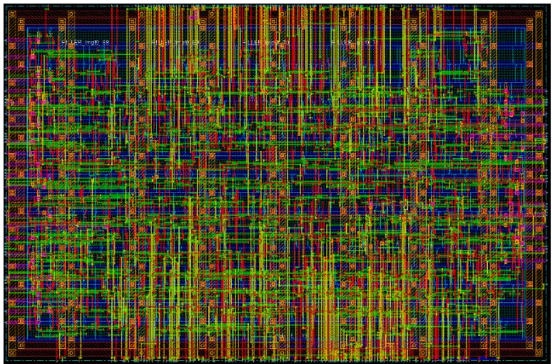
FIGURE 3.15 – Routage d'un cluster
