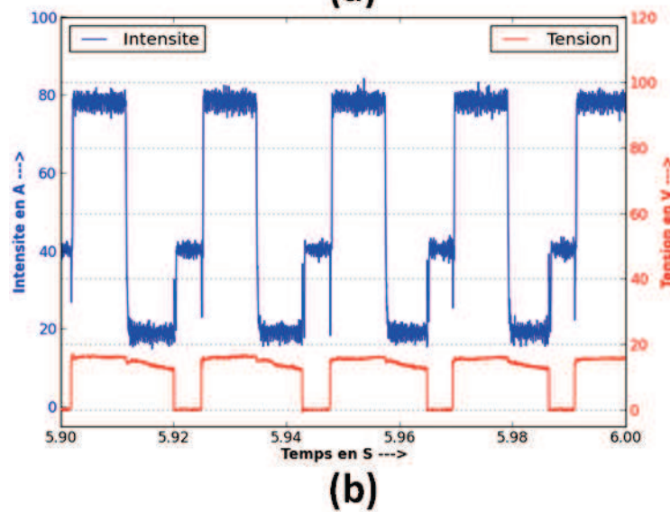
FIGURE II.7: Evolution des signaux de tension et d'intensité correspondant (a) au régime de transfert par court-circuit classique [70], et (b) au régime de transfert CMT.
