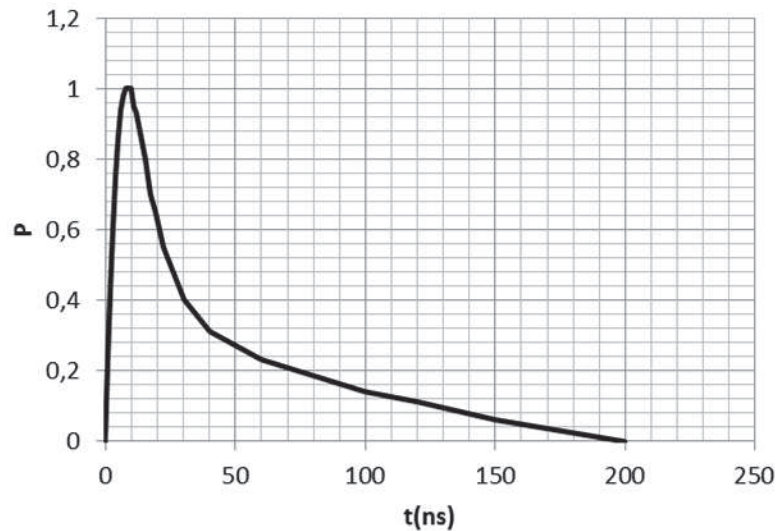
FIGURE IV.26: Exemple de profil de pression modélisé, appliqué au centre de la cible.
