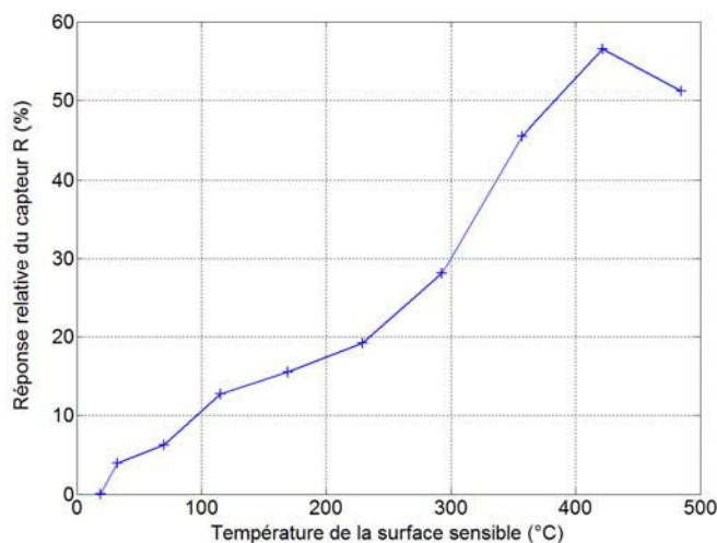
Figure II. 20 - Sensibilité du capteur au benzène en fonction de la température.
