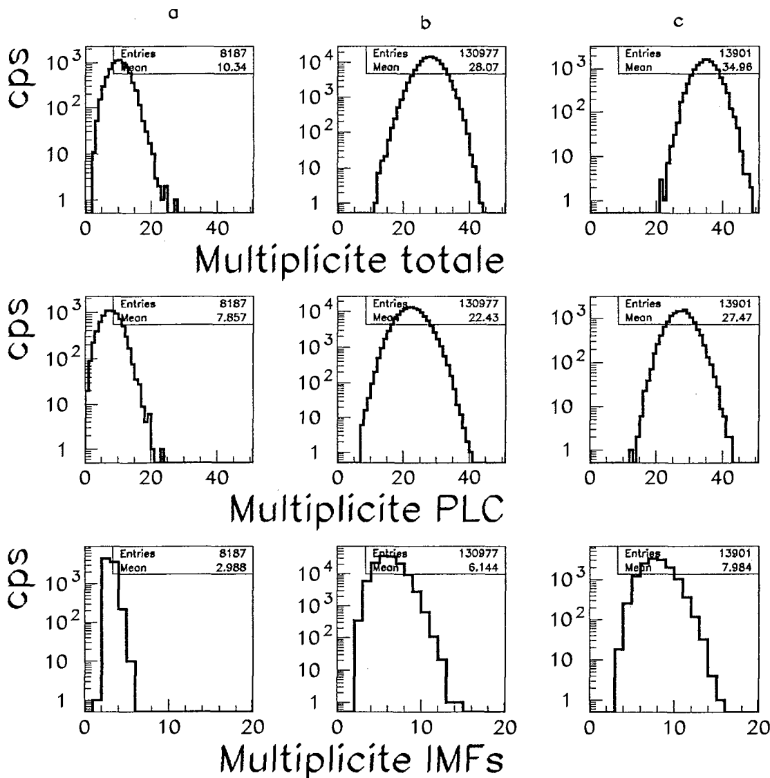
Figure IV.11: Multiplicités totales, des PLC et des IMF's pour la réaction Xe + Sn à 50 AMeV pour les trois coupures a, b et c définies sur la figure IV.9 : colonne de gauche extrémité gauche de la géodésique, au milieu tranche intermédiaire et colonne de droite extrémité droite de la géodésique. Les coupures en question sont présentées sur la figure IV.9.
