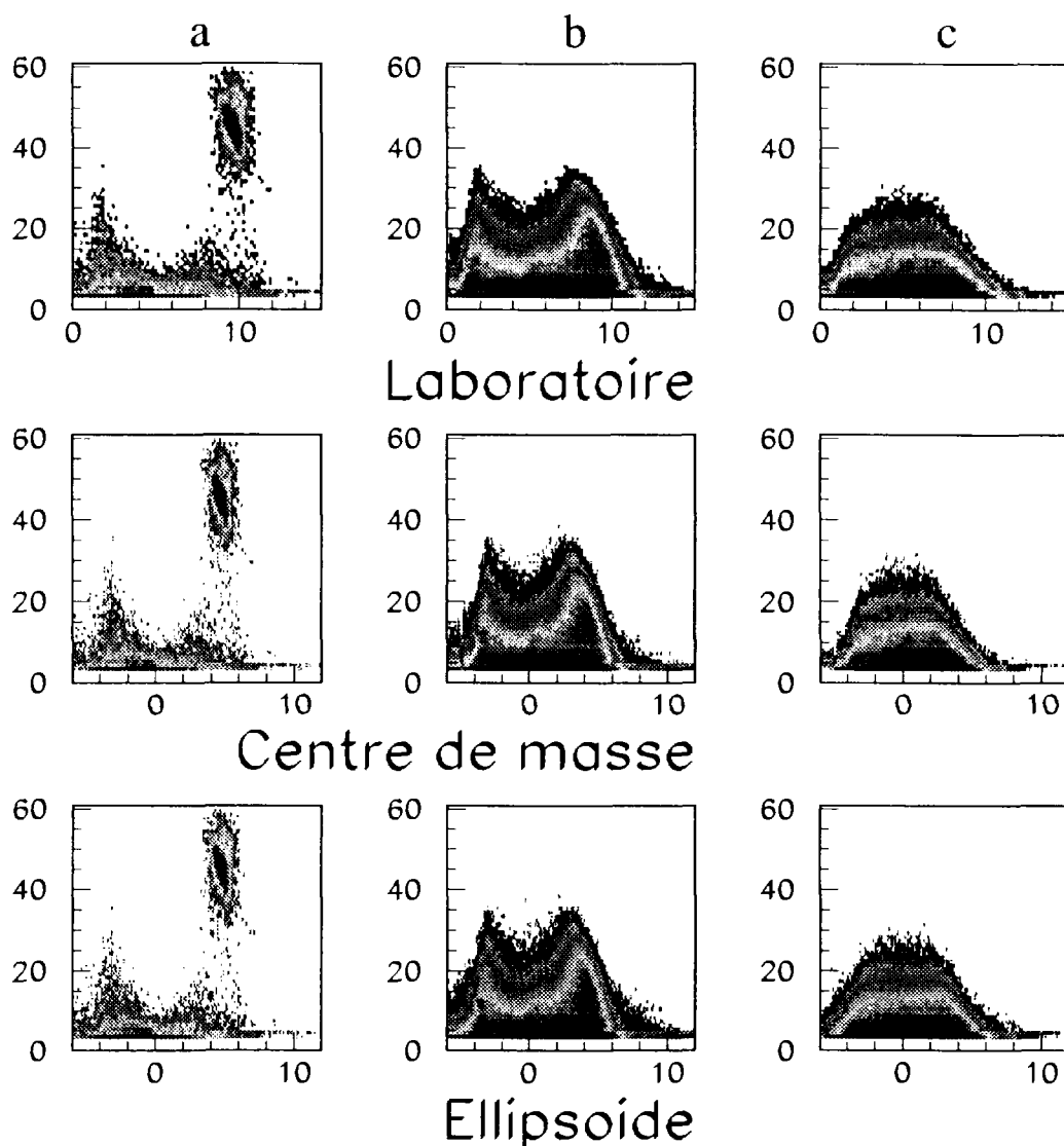
Figure IV.12: Corrélation entre la charge et la vitesse (cm/ns) dans le laboratoire (en haut), dans le centre de masse(milieu) et dans l'ellipsoïde(en bas) pour la réaction Xe + Sn à 50 A MeV pour trois coupures a, b et c définies sur la figure IV.9 dans la variable g, présentées sur la figure IV.9.
