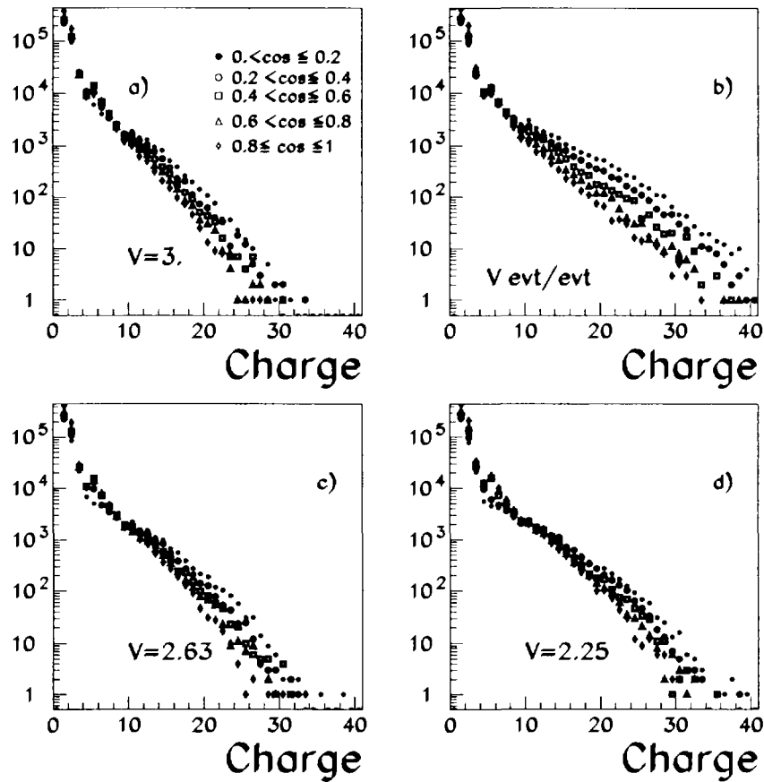
Figure V.24: Superposition des distributions de charge en fonction du domaine angulaire d'émission dans le centre de masse pour le système Ni + Au à 90 A.MeV pour les 4 calculs possibles : valeur théorique a), calcul événement par événement à partir des fragments b) ou calcul à partir des fragments c) et calcul à partir des protons d).
