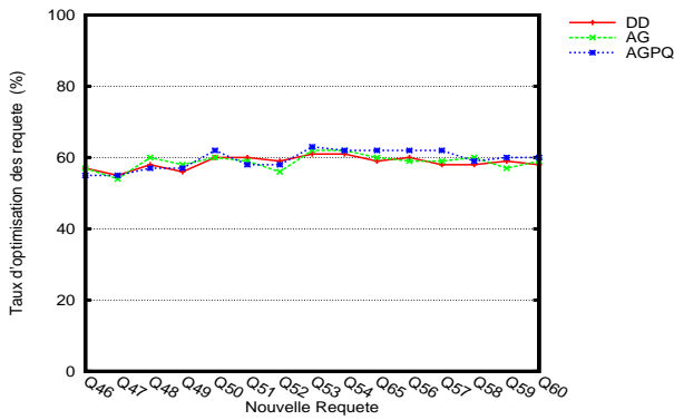
FIGURE 2.24 – Taux l’optimisation du coût (cas 60 requêtes avec Profiling)
