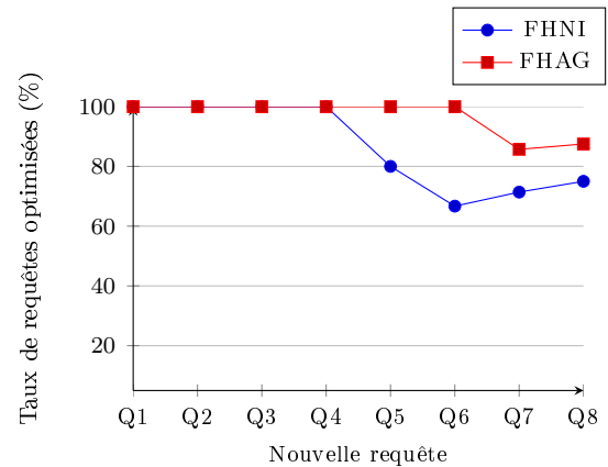
FIGURE 2.19 – Taux de requêtes optimisées (cas 8 requêtes)
