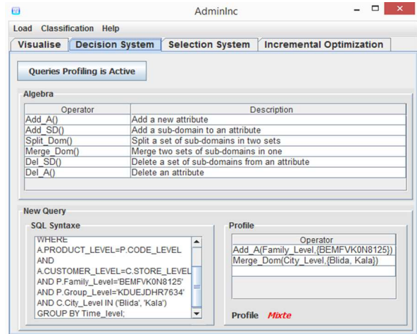
FIGURE 6.5 – Activation du Système Décisionnel, Algèbre et Profil de requête
