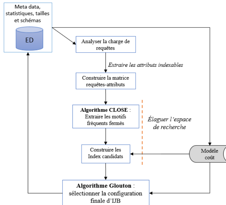
FIGURE 1.5 – Architecture pour la sélection des IJB : Aouiche et al.
