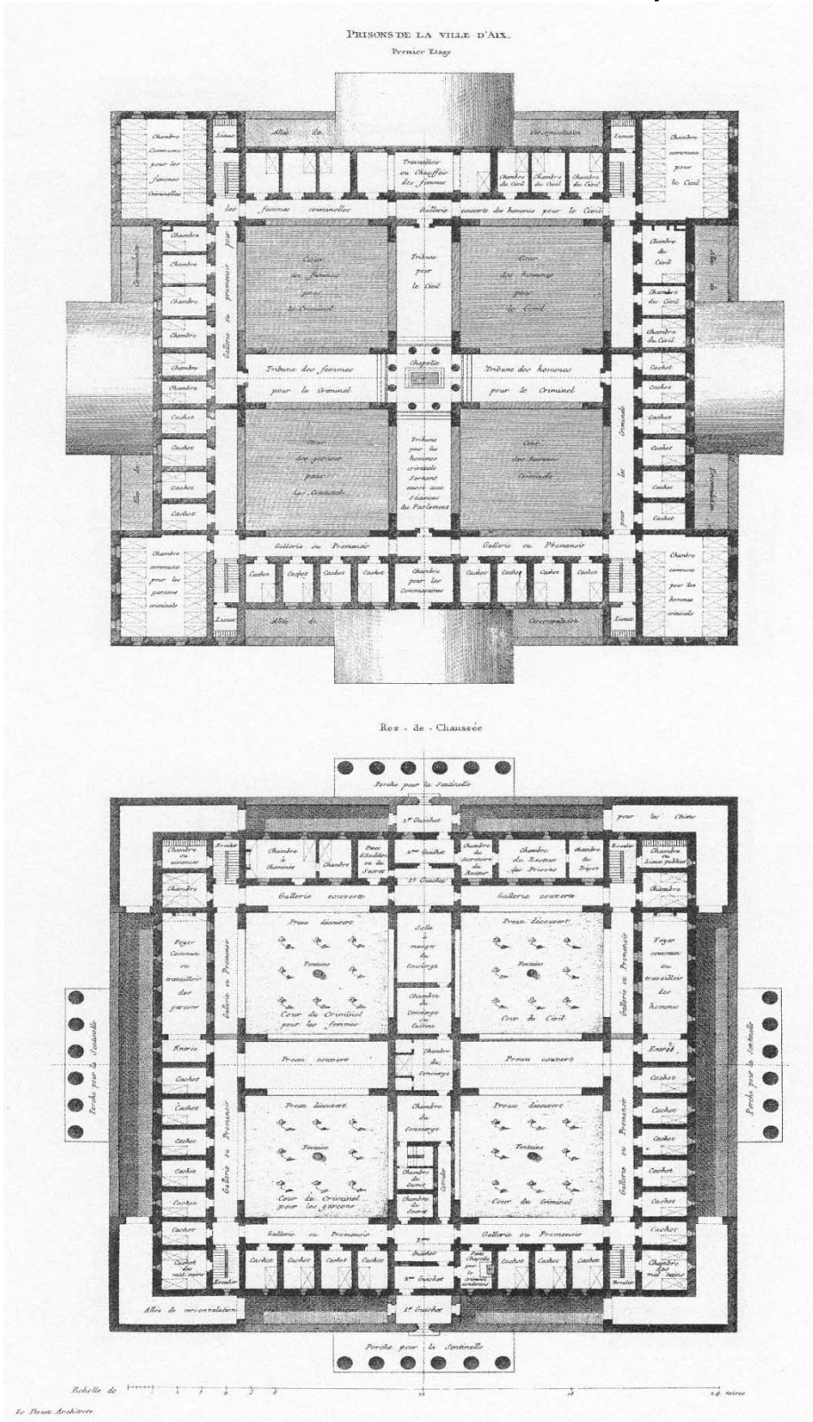
Claude-Nicolas Ledoux, L'architecture considérée sous le rapport de l'Art, des mœurs et de la législation , Paris, Ledoux, 1804, 2 vol., pl. 187
