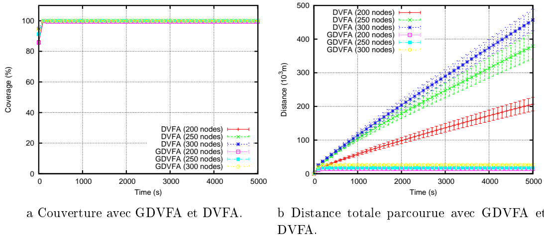
Figure B.7: Taux de couverture et distance totale parcourue avec DVFA et GDVFA.
