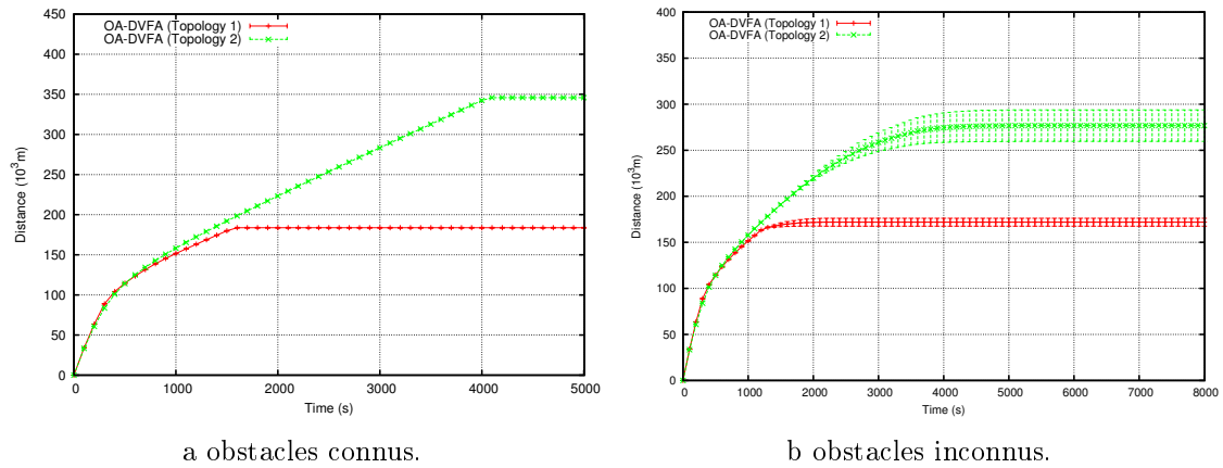
Figure B.10: Distance totale parcourue en fonction du temps.
