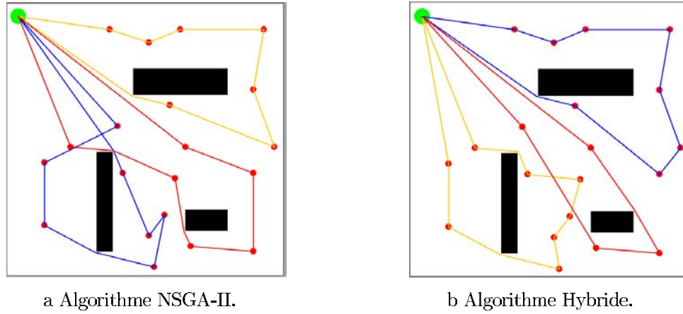
Figure B.15: Tours effectués par 3 robots avec 20 PoIs et des obstacles.
