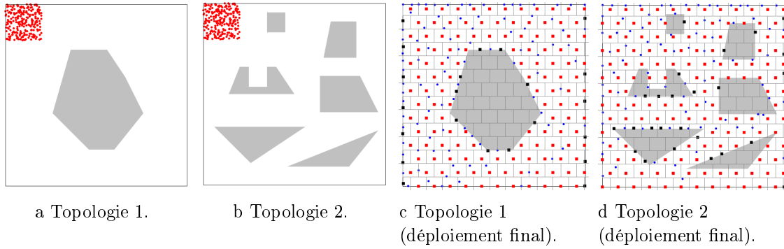
Figure B.8: Déploiements initiaux et finaux.
