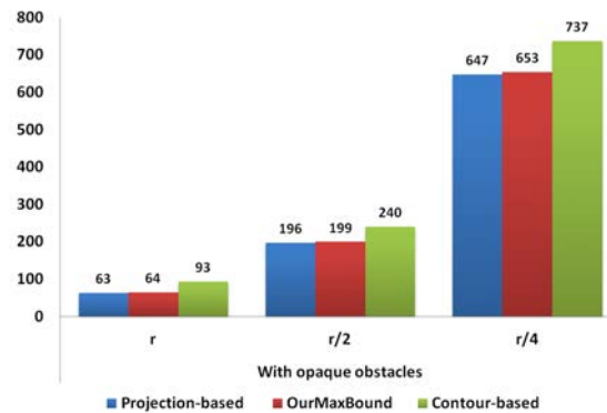
Figure B.12: Impact du rayon de capture sur le nombre total de noeuds.
