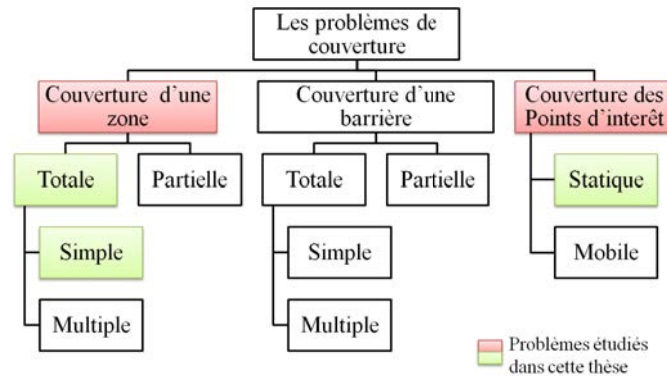
Figure B.1: Les problèmes de couverture.
