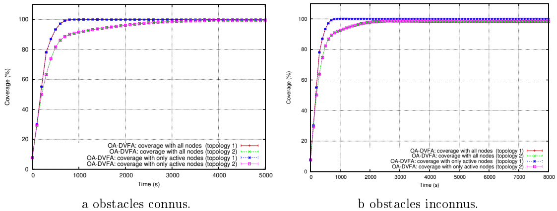
Figure B.9: Taux de couverture et distance totale parcourue avec OA-DVFA.
