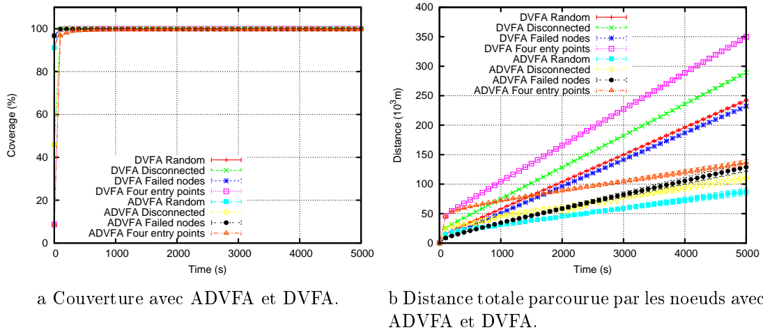
Figure B.6: Taux de couverture et distance totale parcourue avec ADVFA et DVFA.
