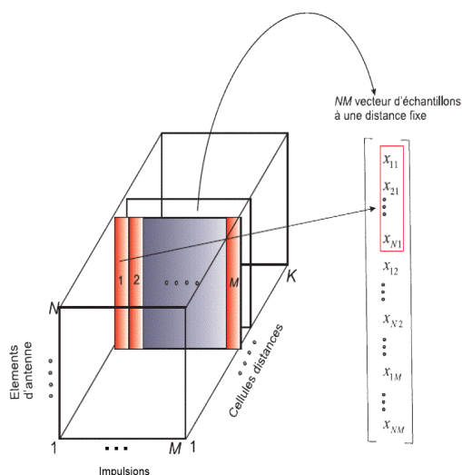
FIGURE 4.3 – Data Cube STAP et arrangement de données.
