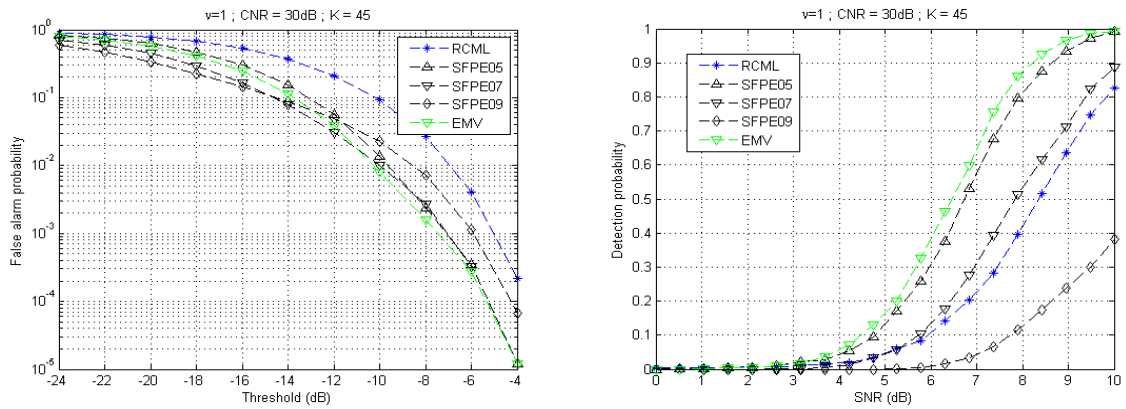
FIGURE 4.6 – Gauche : probabilité de fausse alarme en fonction du seuil. Droite : probabilité de détection en fonction du SNR pour PFA = 10^{-3} . K = 3R , \nu = 1 , CNR = 30\text{dB} .
