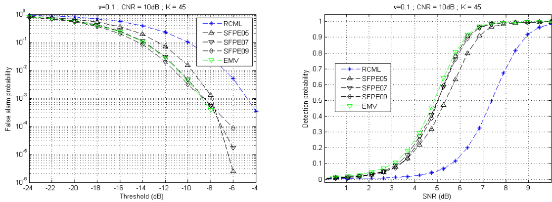
FIGURE 4.9 – Gauche : probabilité de fausse alarme en fonction du seuil. Droite : probabilité de détection en fonction du SNR pour PFA= 10^{-3} . K = 3R , \nu = 0.1 , CNR= 10dB.
