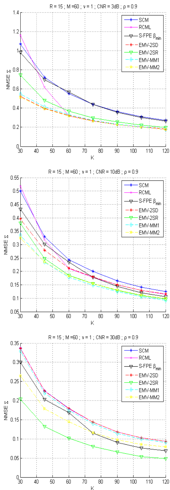
FIGURE 2.2 – NMSE sur \Sigma_{tot} des différents estimateurs. M = 60 , R = 15 , \nu = 1 . De haut en bas : CNR = [3, 10, 30]dB.
