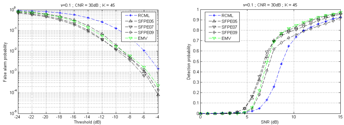
FIGURE 4.7 – Gauche : probabilité de fausse alarme en fonction du seuil. Droite : probabilité de détection en fonction du SNR pour PFA = 10^{-3} . K = 3R , \nu = 0.1 , CNR = 30\text{dB} .
