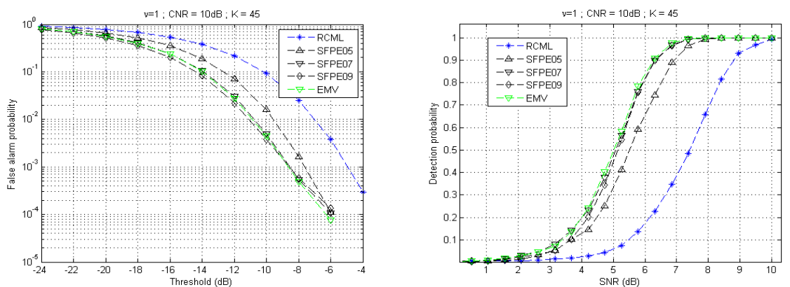
FIGURE 4.8 – Gauche : probabilité de fausse alarme en fonction du seuil. Droite : probabilité de détection en fonction du SNR pour PFA = 10^{-3} . K = 3R , \nu = 1 , CNR = 10\text{dB} .
