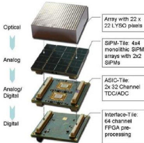
Figure 18: schéma du système de photodétection Cristal / SiPM / système ASIC (Application-Specific Integrated Circuit) pour la numérisation du signal analogique / système de pré-traitement FPGA (field-programmable gate array) : il s'agit d'un circuit logique intégré programmable capable de traiter différentes informations du signal numérique dont l'énergie d'impulsion totale de l'évènement et l'instant t de cette impulsion pour l'appariement des paires de photons coïncidents. Schéma extrait de l'article de Vandenberghe et al. [128].
