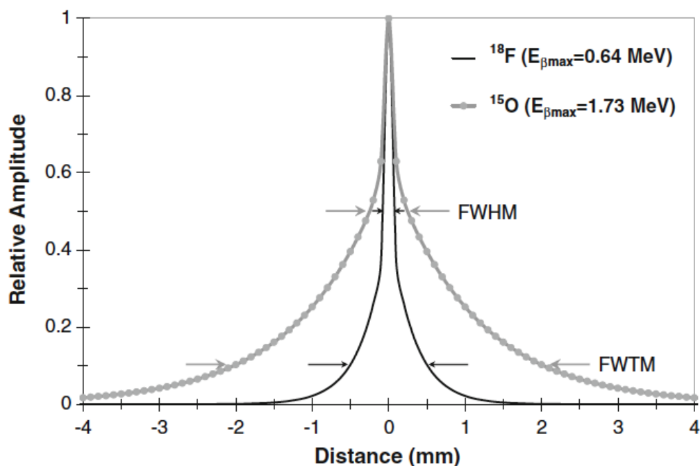
Figure 14 : Profil de distribution du parcours du positron dans les tissus pour le ^{18}\text{F} et ^{15}\text{O} (FWHM = Full-width-at-half-maximum et FWTM = Full-width-at-tenth-of-maximum). En abscisse: distance parcouru par le positon ; en ordonnée : nombre relatif de positons. Schéma extrait de l'article de Lecomte et al. [125].
