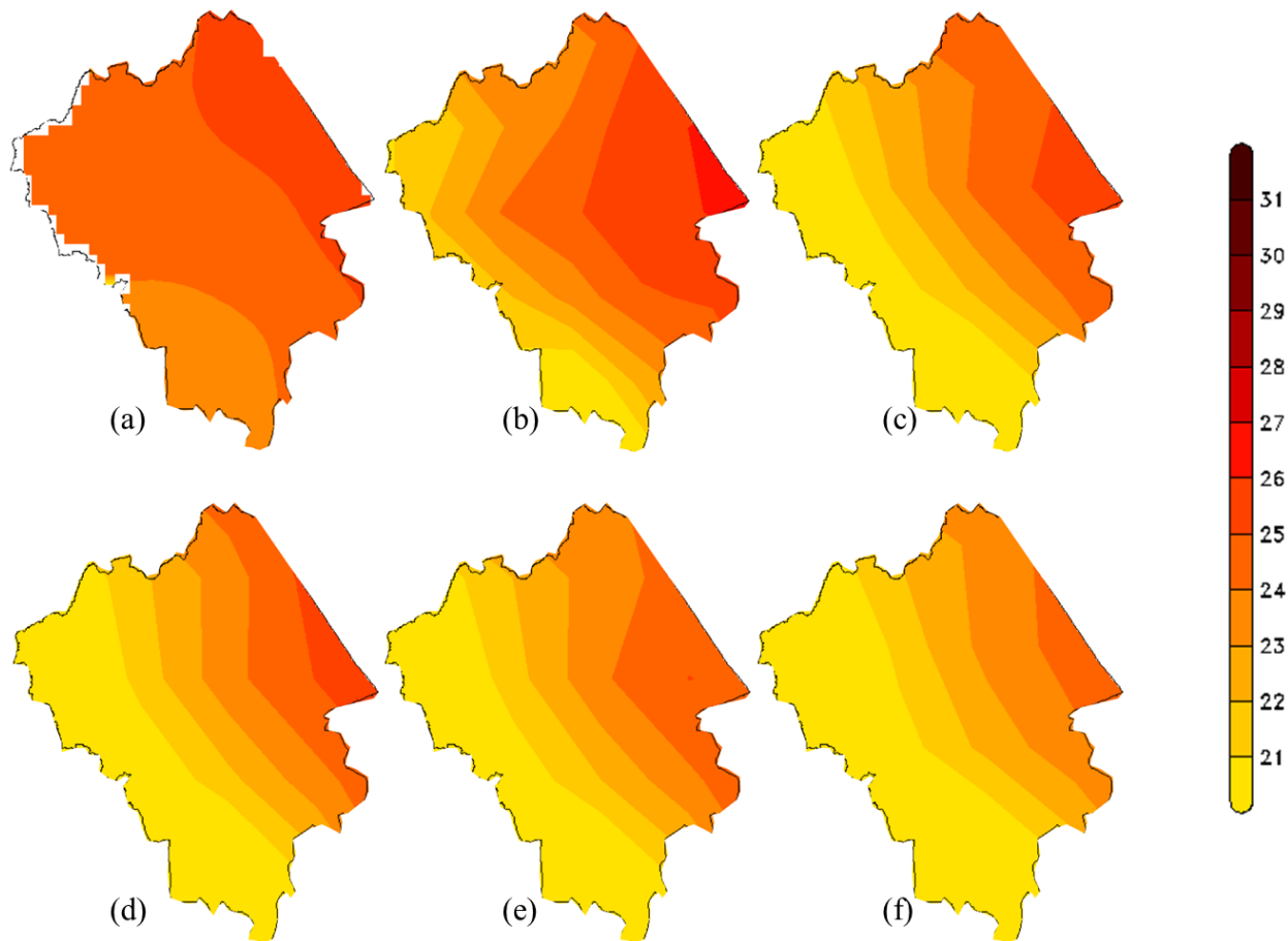
Figure 5.2. Present day climate for temperature (°C) for (a) STATION (b) APHRODITE (c) WRF/ERA (d) WRF/ECHAM (e) WRF/CCSM (f) WRF/MIROC
