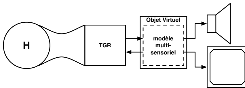
Figure 1.7. Architecture pour la simulation du geste instrumental
