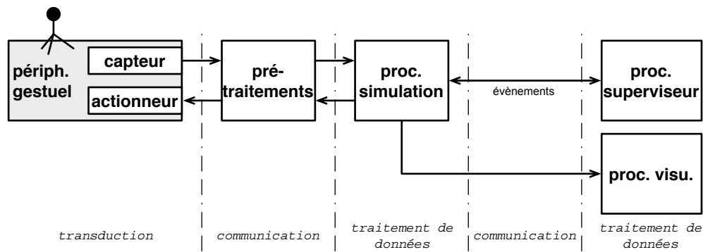
Figure 4.2. Composants fonctionnels de la boucle de simulation haptique
