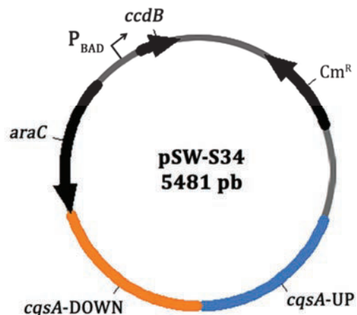
Figure 45 : Cartographie du plasmide pSW-S34. ccdB : gène codant pour la toxine CcdB ; araC : gène codant pour le régulateur AraC. P_{BAD} : promoteur inducible par le complexe AraC/arabinose.
