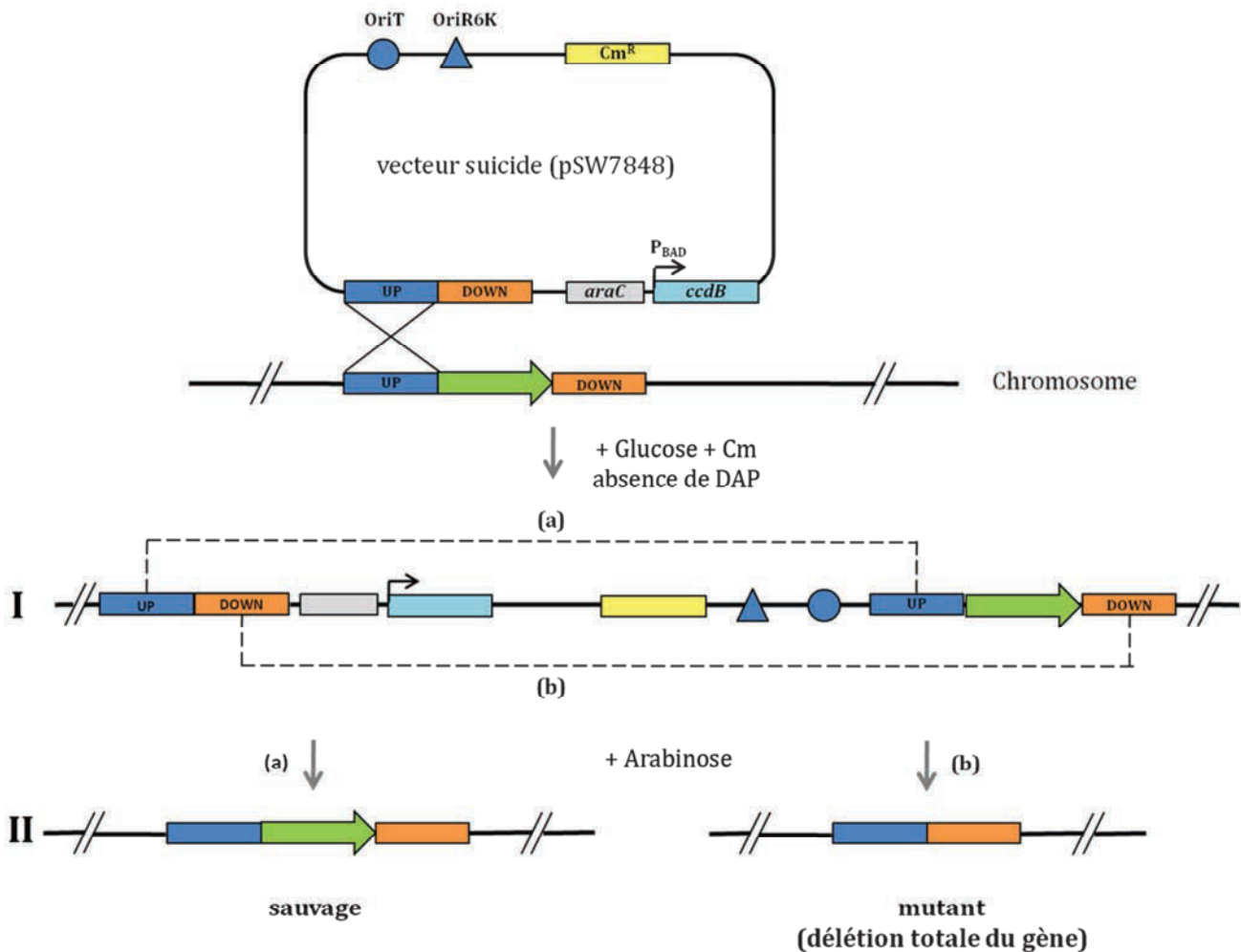
Figure 22 : Principe de la mutagénèse dirigée du gène cqsA chez V. tapetis par double recombinaison homologue. I: première recombinaison homologue; II: deuxième recombinaison homologue; Cm: chloramphénicol; araC : gène codant pour le régulateur AraC; ccdB : gène codant pour la toxine CcdB; OriT : origine de transfert; OriR6K : origine de réplication R6K.
