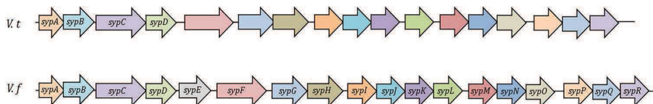
Figure 40 : Représentation schématique de l'organisation du locus syp chez V. tapetis CECT4600 (V.t) et V. fischeri ES114(V.f). (Données obtenues à partir de l'outil MaGe).
