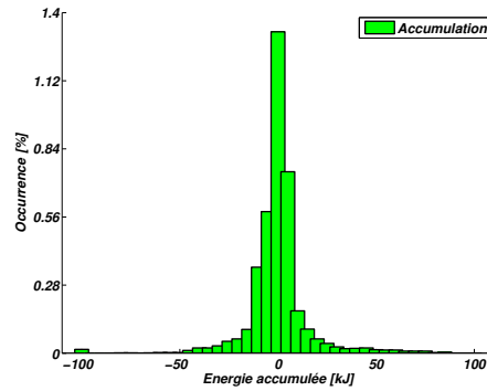
(a) Accumulation d'énergie sur le nœud U_a
