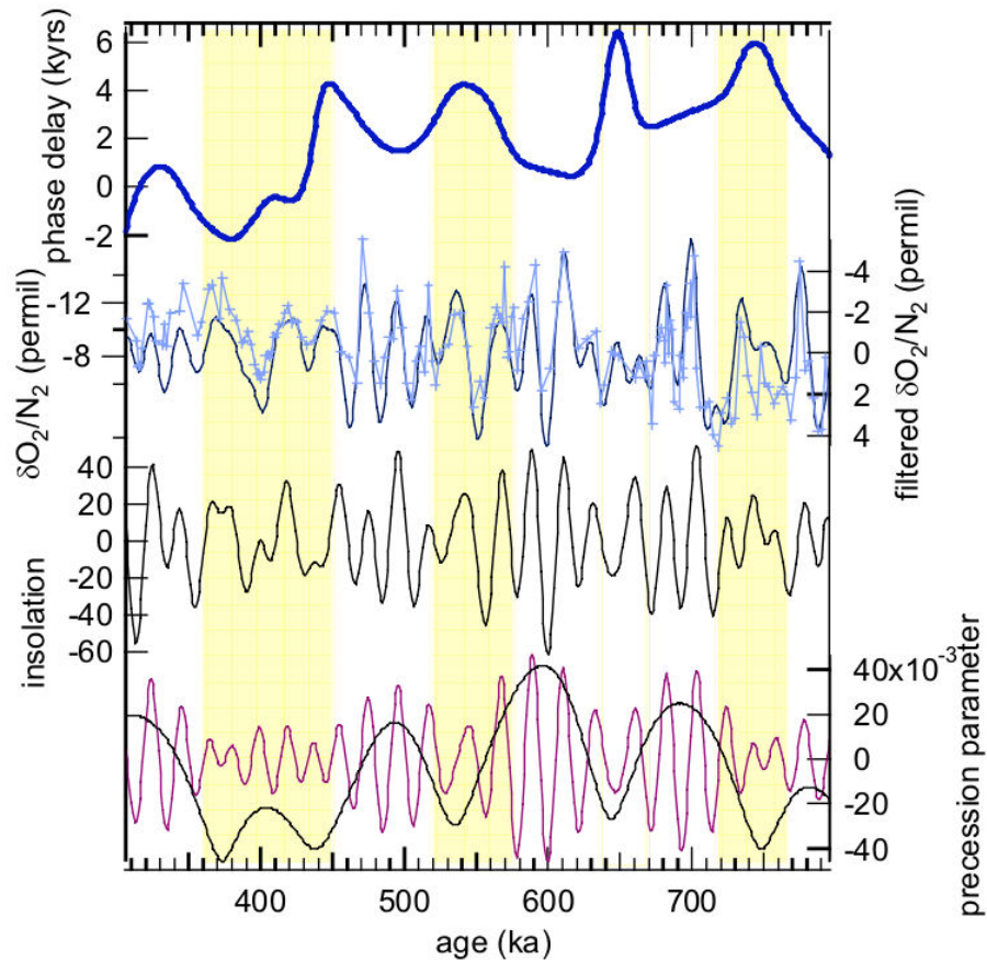
FIGURE 1.5 – Evolution du \delta O_2/N_2 mesuré à EDC entre 300 et 800 ka. De bas en haut : courbes de précession et d'excentricité, insolation locale au solstice d'été, courbe composite du \delta O_2/N_2 (données corrigées et données mesurées sur la glace à -50^\circ\text{C} ) et filtrée entre 15–100 ka, retard entre le \delta O_2/N_2 et l'insolation locale (filtrés entre 15 et 100 ka). En Jaune sont mises en évidence les périodes où le \delta O_2/N_2 ne ressemble pas à l'insolation locale. Extrait de Landais et al. [2012].
