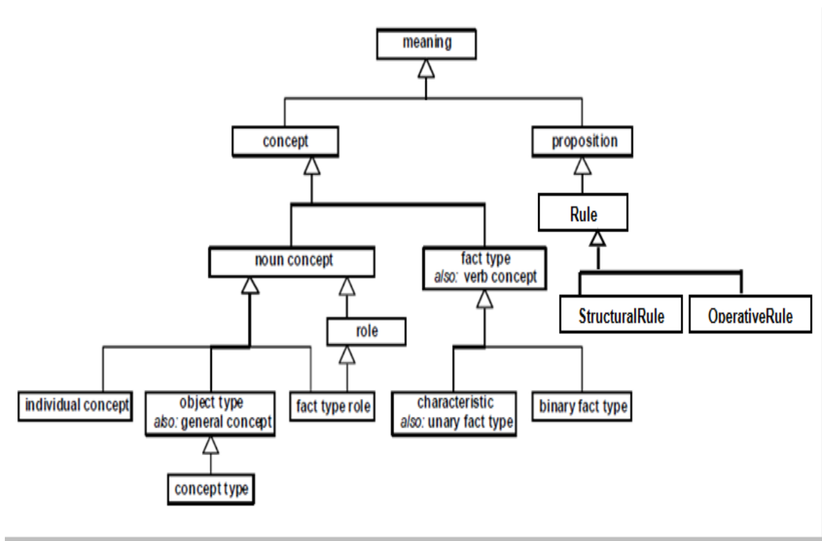
Figure 3.9 : Extrait du méta-modèle SBVR : Meanings (OMG, 2008a)
