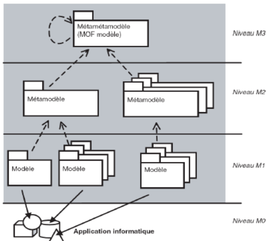
Figure 3.2 : Architecture à quatre niveaux du MDA
