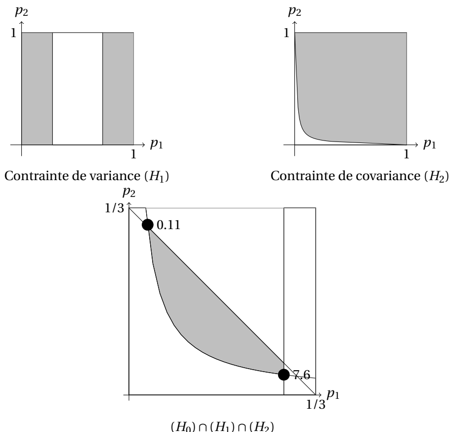
FIGURE 4.4 – Illustration de contraintes de variances et co-variances. Les zones grises correspondent à l'ensemble des couples (p_1, p_2) valides en fonction des contraintes indiquées ainsi que de la contrainte (H_0) d'équilibre des réactifs (permettant de se ramener à un espace plan). Les points noirs correspondent aux valeurs extrêmes de p_1/p_2 .
