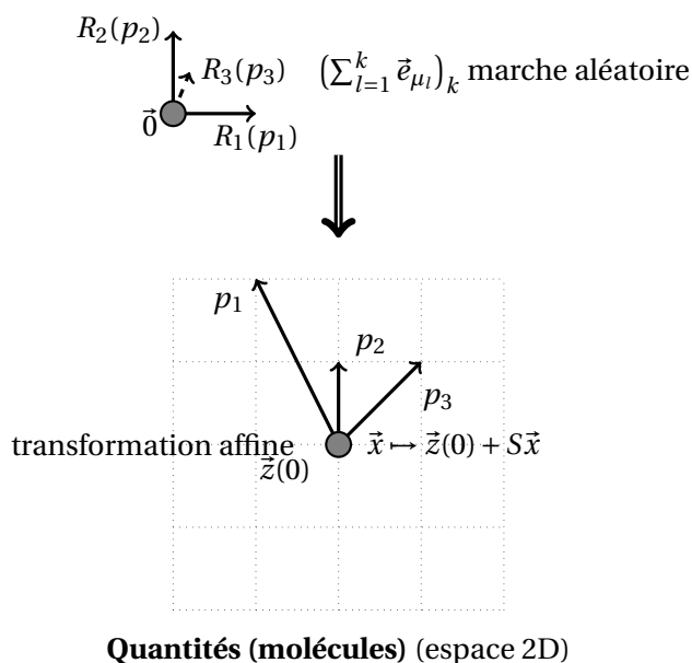
FIGURE 3.5 – Illustration du comportement de marche aléatoire sur l'exemple du réseau \{X \rightarrow 2Y; \emptyset \rightarrow Y; \emptyset \rightarrow X + Y\} . La sphère représente l'état courant du réseau et les flèches les nouveaux états possibles après l'occurrence de chacune des réactions qui a lieu avec probabilités p_i .
