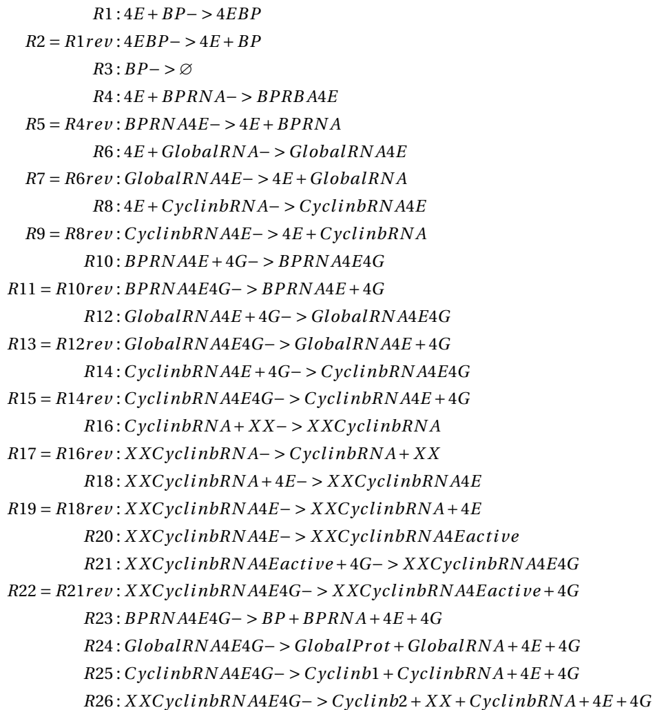
FIGURE 1.2 – Modèle de synthèse protéique à deux voies chez l'oursin. Le but de ce modèle est d'introduire le cas particulier de la synthèse de la cyclineB qui serait synthétisée par deux voies, c'est-à-dire deux mécanismes distincts. Le mécanisme de la seconde voie est inspiré de celui d'une espèce marine voisine.
