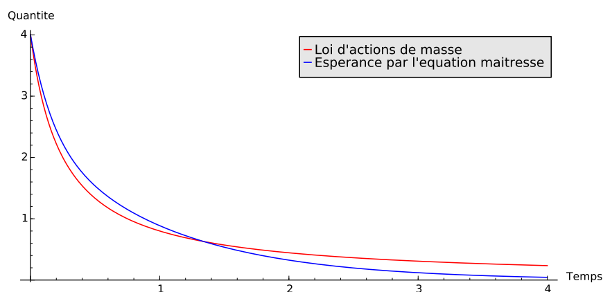
FIGURE 2.1 – Comparaison entre loi d'action de masse et équation maîtresse pour l'exemple des désintégrations par paires. En rouge, la loi d'action de masse prédit une décroissance inverse. En bleu, l'espérance issue de l'équation maîtresse prédit une décroissance exponentielle. Il est donc faux en général d'énoncer que la loi d'action de masse décrit les valeurs moyennes des quantités de matière.
