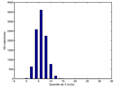
Processus discrétisé, \delta t = 0,001
