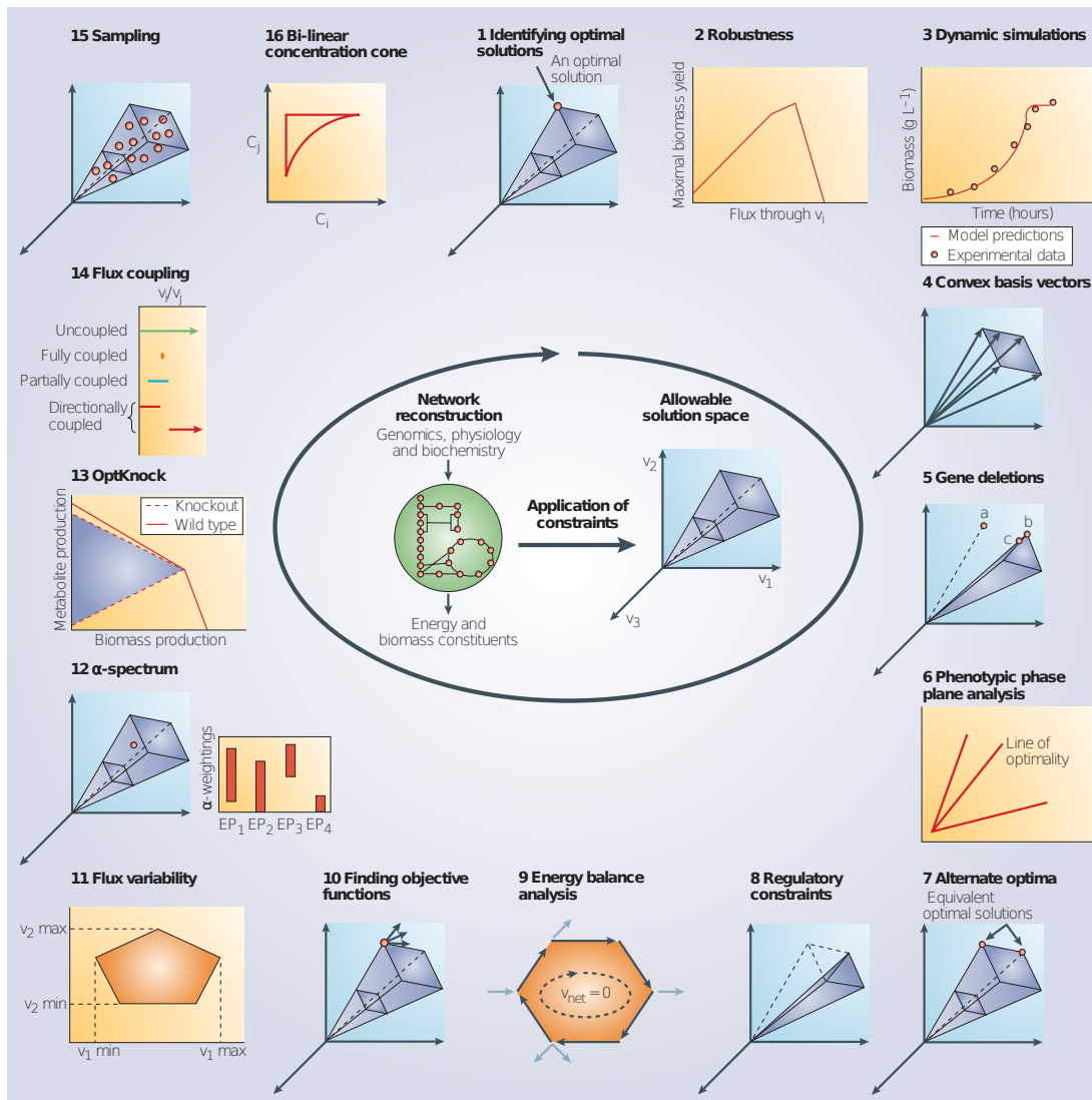
FIGURE 1.3 – Quelques méthodes d'analyse reposant sur un système de contraintes des flux à l'équilibre. (image extraite de [PRP04])
