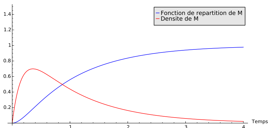
FIGURE 2.2 – Loi de probabilité du temps de vie d'un système de molécules se désintégrant par paires. Cette information ne peut-être obtenue par la lois d'action de masse.
