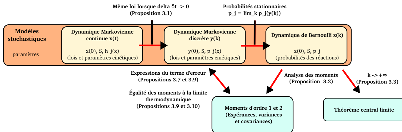
FIGURE 3.1 – Diagramme représentant les résultats principaux du chapitre 3.
