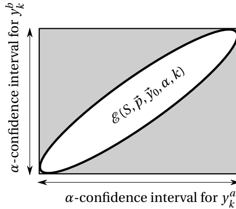
FIGURE 4.5 – Comparaison entre l'ellipsoïde de confiance et la multiplication des intervalles de confiance pour deux espèces. La figure illustre l'avantage de l'utilisation de méthodes multivariées. Le rectangle obtenu par multiplication des interfaces est plus grand que l' \alpha -ellipsoïde de confiance. La zone grise correspond aux prédictions exclues par la méthode multivariée grâce à l'utilisation des corrélations entre les deux espèces.
