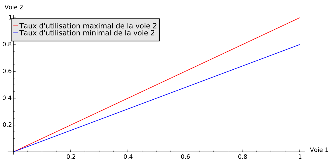
FIGURE 1.4 – Comparaison des taux d'utilisation des deux voies dans le modèle de synthèse protéique chez l'oursin. Ce graphique représente des bornes pour les valeurs possibles de f_{26} en fonction de celles de f_{25} et d'après les hypothèses que nous avons formulées.
