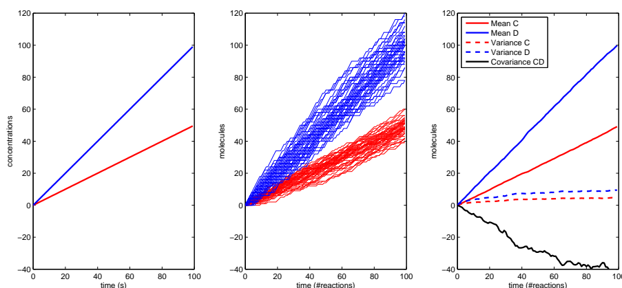
FIGURE 4.2 – Données de départ pour discriminer les modèles 1 ou 2. Les données ont pour forme un ensemble de trajectoires dont on a estimé les moments d'ordre 1 et 2.
