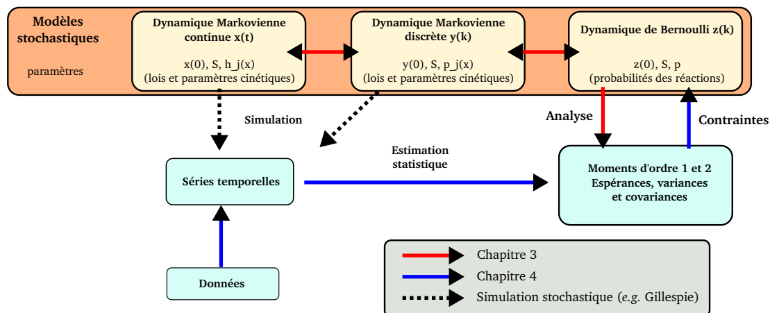
FIGURE 4.1 – Diagramme résumant les principales approches décrites dans les chapitres 3 et 4
