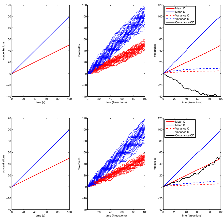
FIGURE 1 – Réseaux distinguables par leurs moments d'ordre 2 Dynamiques différentielles et stochastiques pour le modèle 1 (première ligne) et le modèle 2 (seconde ligne) décrits dans Eq. (3). Les courbes rouges (resp. bleues) représentent les quantités de C (resp. D). La première colonne représente la solution de l'équation différentielle issue de la loi d'action de masse. La seconde colonne représente 50 générations de trajectoires aléatoires obtenues à l'aide d'un algorithme de simulation stochastique. Les paramètres cinétiques et stochastiques ont été fixés à 1 et il y a 1000A et 1000B initialement. La troisième colonne représente les estimations des espérances, des variances et des covariances croisées entre C et D . Ces estimations sont obtenues à partir des 50 trajectoires de la seconde colonne. On constate que seule la trajectoire des covariances de C et D permettent de distinguer ces réseaux.
