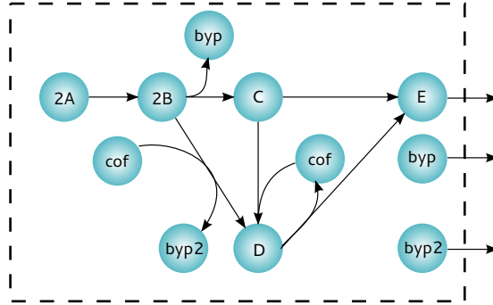
FIGURE 4.7 – Retour sur l'exemple du réseau métabolique introductif dont les réactions et la matrice de stœchiométrie ont été introduits dans le chapitre 1.
