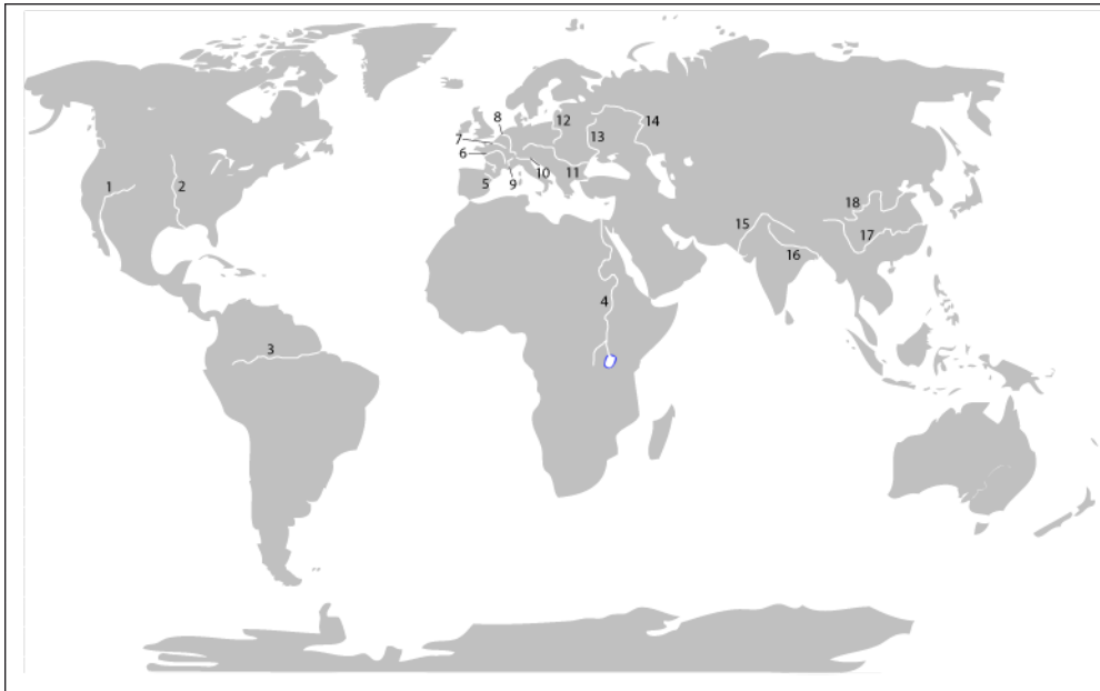
1- Colorado. 2- Mississippi. 3- Amazone. 4- Nil. 5- Ebre. 6- Loire. 7- Seine. 8- Rhin. 9- Rhône. 10- Pô. 11- Danube. 12- Vistule. 13- Dniepr. 14- Volga. 15- Indus. 16- Gange. 17- Yang Tsé. 18. Huang Hé
