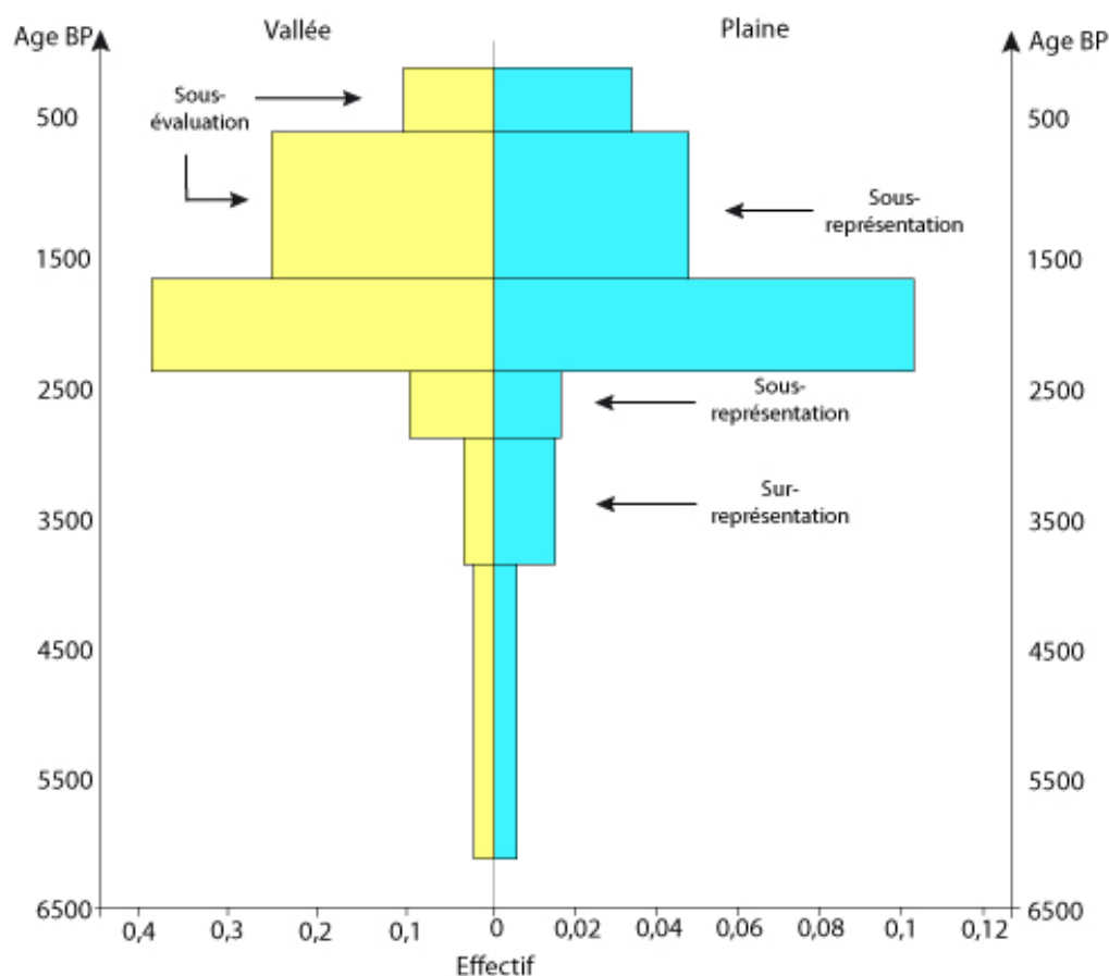
Figure 26 : Représentation graphique de la normalisation par la durée du nombre de site par période, dans la vallée et dans la plaine alluviale
