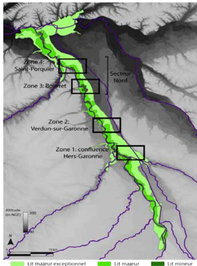
Figure 12 : Localisation des secteurs préférés
