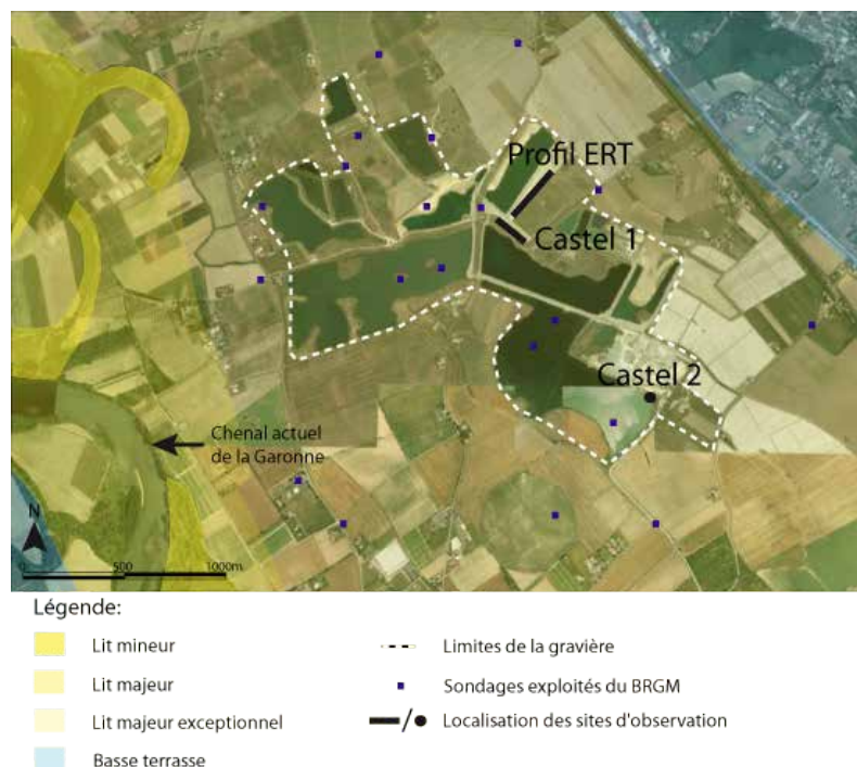
Figure 41 : Localisation de la zone de travail dans le secteur de Castelnaud-d'Estretfonds
