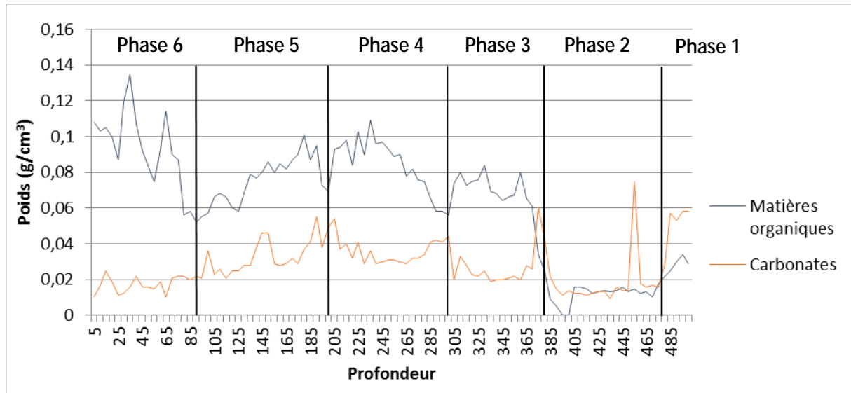
Figure 67 : Courbe de poids ( \text{g}/\text{cm}^3 ) de matière organique et de carbonates dans RAN 3
