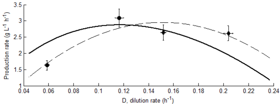
Figure 0.3 Modélisation l'étape SSPHF à l'état stationnaire. Comparaison entre les données expérimentales et le modèle pour l'essai 1 (●) et l'essai 2 (◆). (—) Modèle à l'état stationnaire ( - - - ) Approximation polynomiale des données expérimentales.
