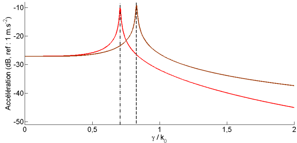
Figure 2-35 : Amplitude de l'accélération spectrale de la plaque in-vacuo à f = 2f_c ; (—) : modèle de Love-Kirchhoff, (—) : modèle de Mindlin-Timoshenko ; (---) : \gamma = k_f , (---) : \gamma = k_{f\_mt}
