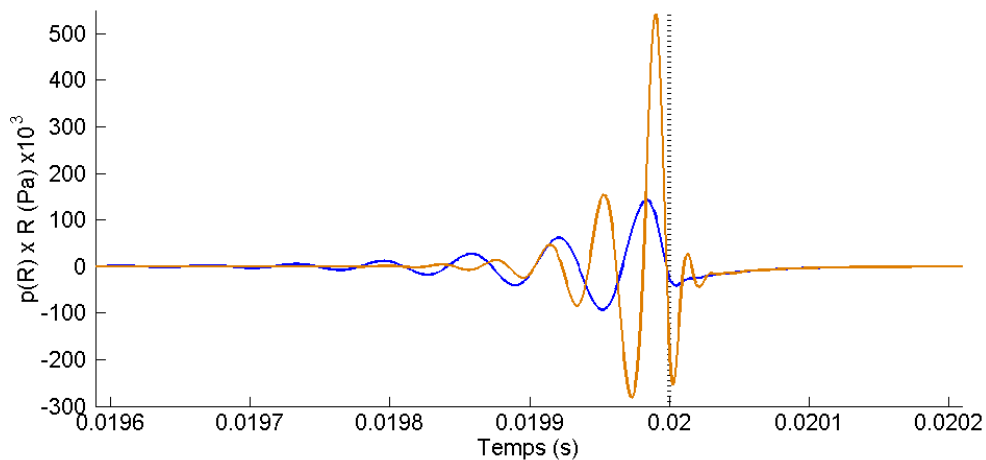
Figure 2-46 : Signaux temporels de pression rayonnée en champ lointain à \theta = 45^\circ (—) : modèle de Love-Kirchhoff, (—) : modèle de Mindlin-Timoshenko ; ( \cdots ) : t = t_{a\_ray} ,
