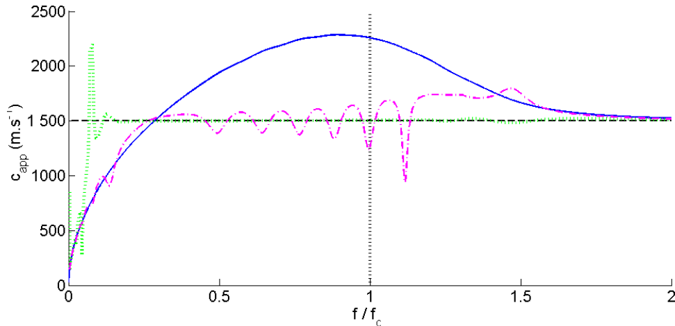
Figure 2-22 : Célérité de groupe d'onde de pression rayonnée en champ proche ; (—) : z = 0 m , (- - -) : z = 0.25 m , (· · ·) : z = 0.5 m ; (· · ·) : f = f_c , (---) : c_{app} = c_0
