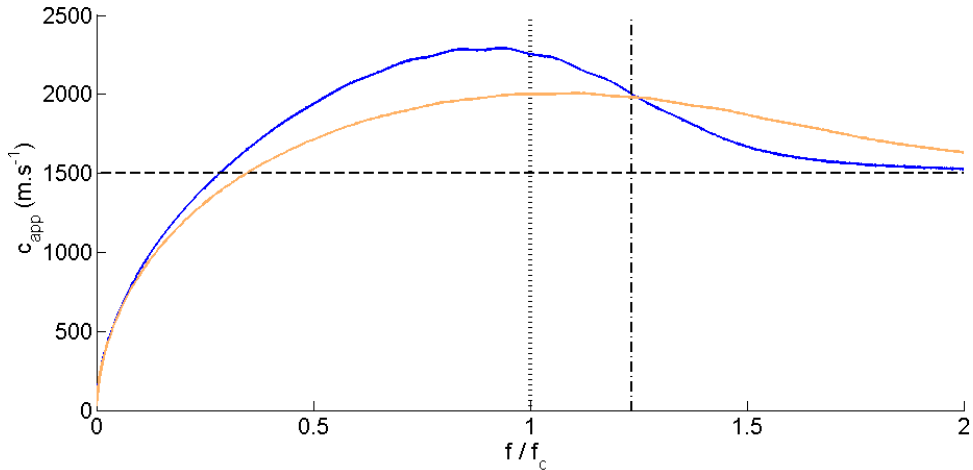
Figure 2-41 : Célérité de groupe d'onde de plaque immergée à r = 5 m ; (—) : modèle de Love-Kirchhoff, (—) : modèle de Mindlin-Timoshenko ; (···) : f = f_c , (- - -) : f = f_{c\_mt}
