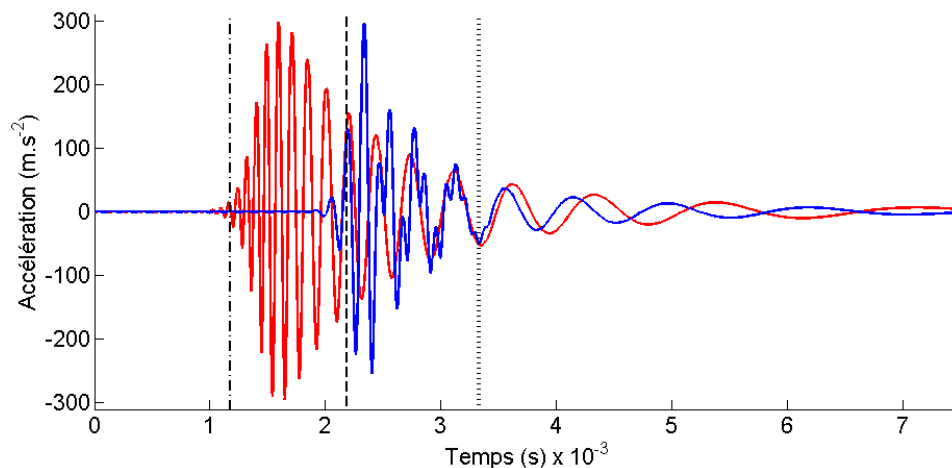
Figure 2-16 : Réponses temporelles d'accélération vibratoire à r = 5 m ; (—) : plaque in-vacuo, (—) : plaque immergée ; (···) : t = t_{G_{fl}} , (---) : t = t_{G_{fl\_eau}} , (···) : t = t_{a\_vib}
