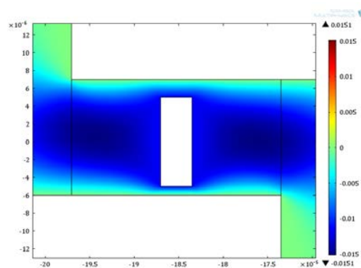
(d) Surface graph of velocity field at 16 kHz.
