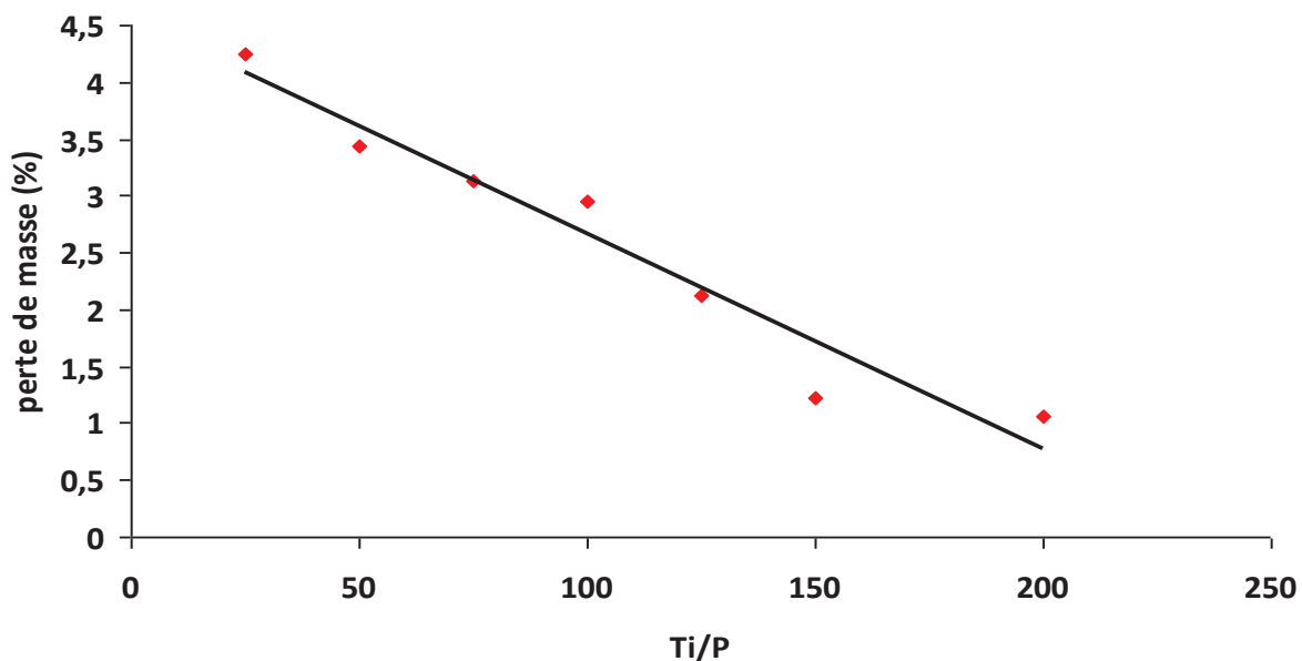
Figure 7 : variation de la perte de masse en analyse thermogravimétrique entre 300 et 500°C en fonction du rapport Ti/P de départ.
