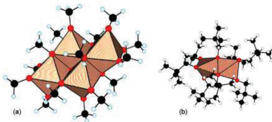
Figure 6: Structures observées à l'état solide pour les composés Ti(OR)_4
