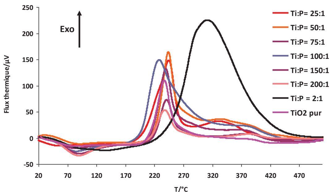
Figure 6 : Analyses thermodifférentielles des nanoparticules de TiO 2 pur et hybrides
