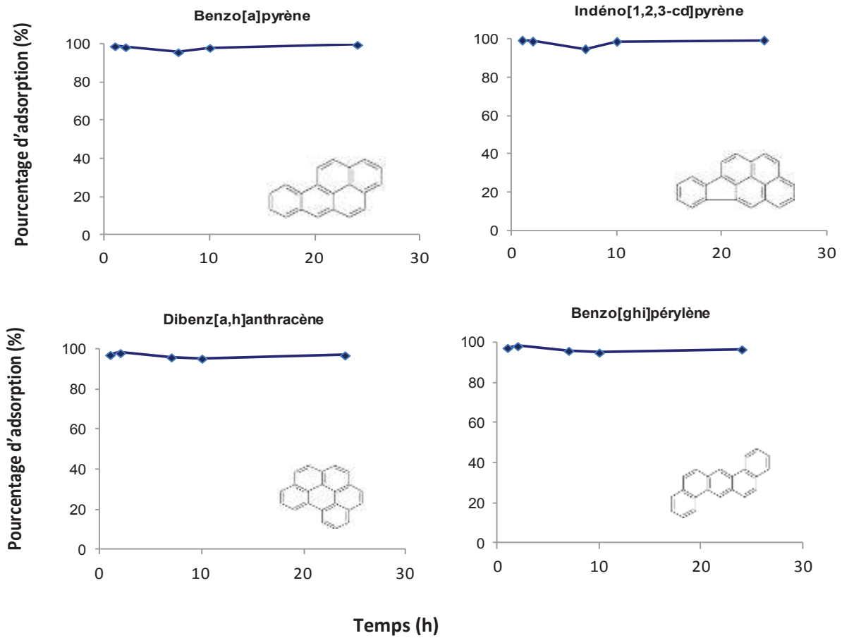
Figure 14 : Cinétiques d'adsorption des 16 HAP EPA sur le matériau (ZrO_2)_{100}(AVP)_1
