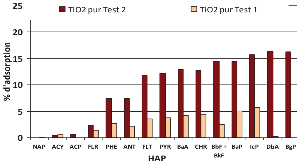
Figure 7 : tests de reproductibilité des résultats d'adsorption sur les mélanges TiO 2 pur+ silice
