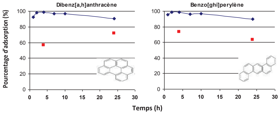
Figure 13 : Cinétiques d'adsorption des 16 HAP EPA sur le (TiO_2)_{100} (tetrahydroisoquinoline) 1
