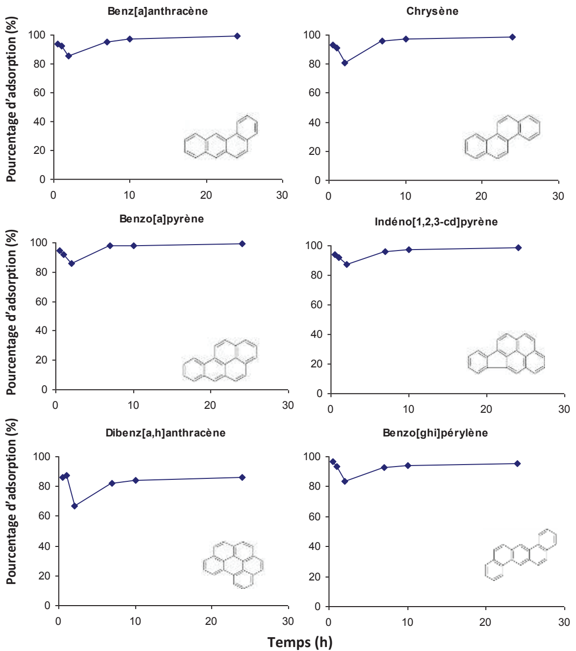
Figure 16: Cinétiques d'adsorption des 16 HAP EPA sur le tissu PP-COOH greffé par (TiO_2)_{100}(AVP)_1 à 0,2M
