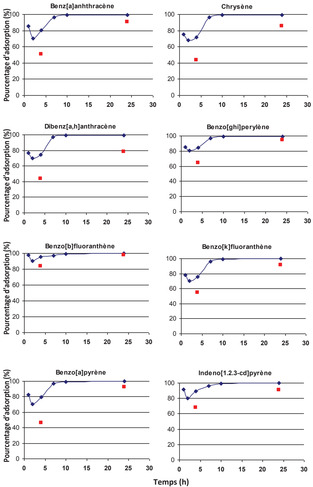
Figure 12 : Cinétiques d'adsorption des 16 HAP EPA sur le (TiO_2)_{100} (naphthylméthylamine) 1
