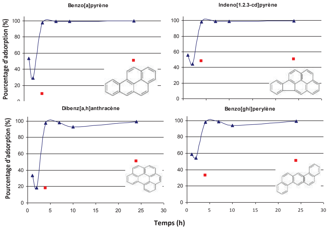
Figure 9 : Cinétiques d'adsorption des 16 HAP EPA sur le matériau (TiO_2)_{100} (AVP) 1
