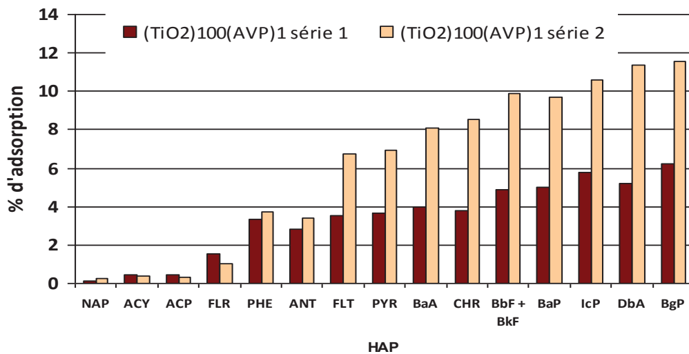
Figure 8 : tests de reproductibilité des résultats d'adsorption sur les mélanges (TiO 2 ) 100 (AVP) 1 +silice
