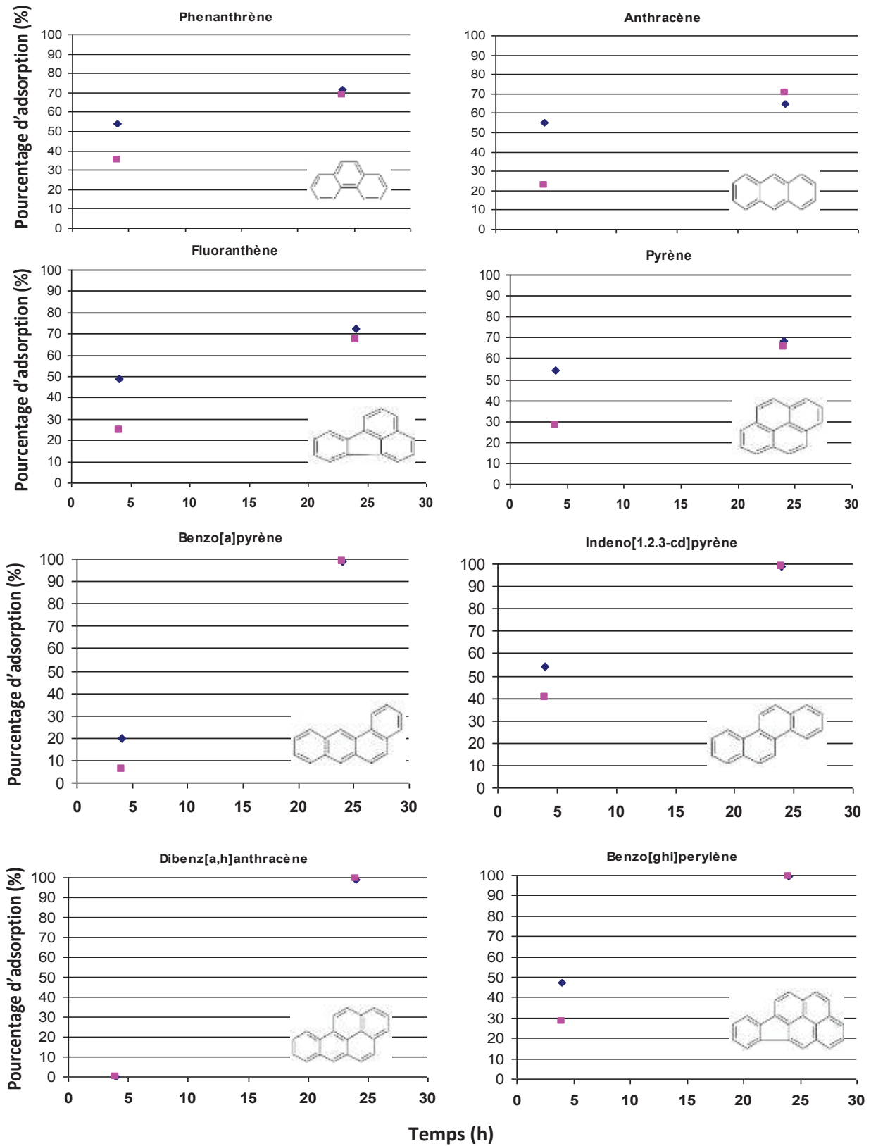
Figure 10 : Cinétiques d'adsorption des 16 HAP EPA sur (TiO_2)_{25}(AVP)_1 et lavage eau (◆) ou eau+éthanol (■).
