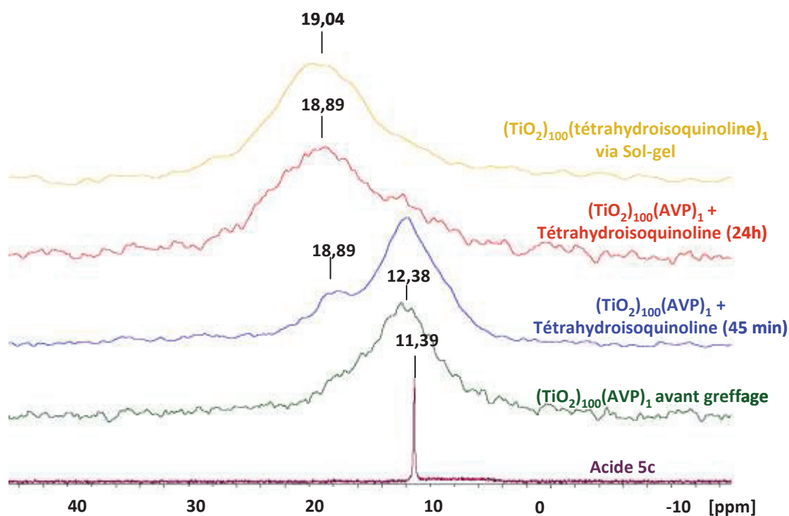
Figure 28 : Spectres RMN ^{31}\text{P} du (\text{TiO}_2)_{100}(\text{tétrahydroisoquinoline})_1 par pré- et post-fonctionnalisation
