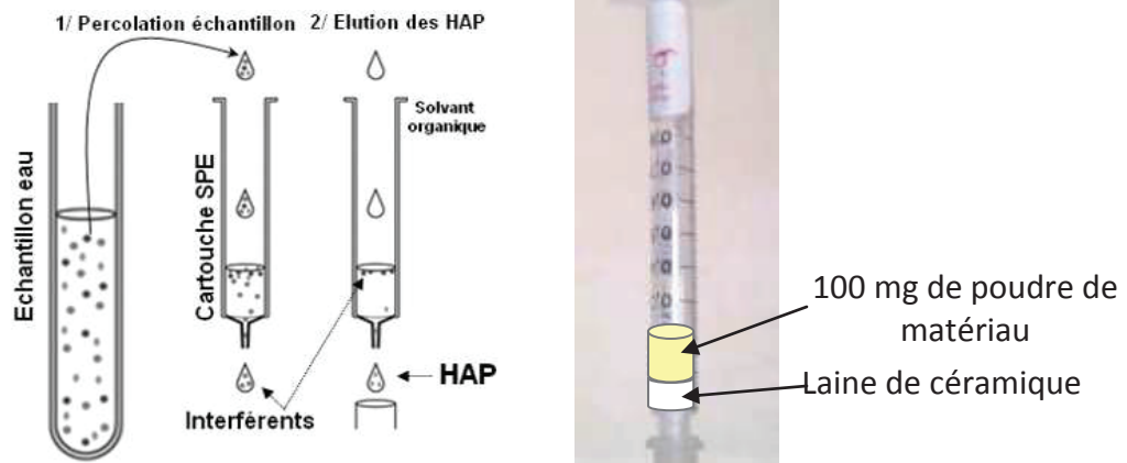
Figure 1 : Principe de la technique d'extraction des HAP par SPE
