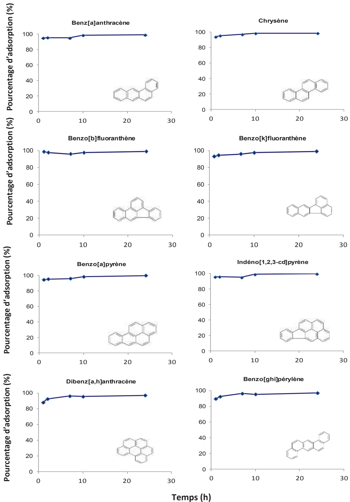
Figure 15: Cinétiques d'adsorption des 16 HAP EPA sur le matériau (ZrO_2)_{90}(TiO_2)_{10}(AVP)_1
